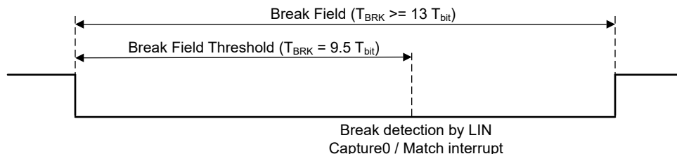
图 19-6. LIN 中断域检测
