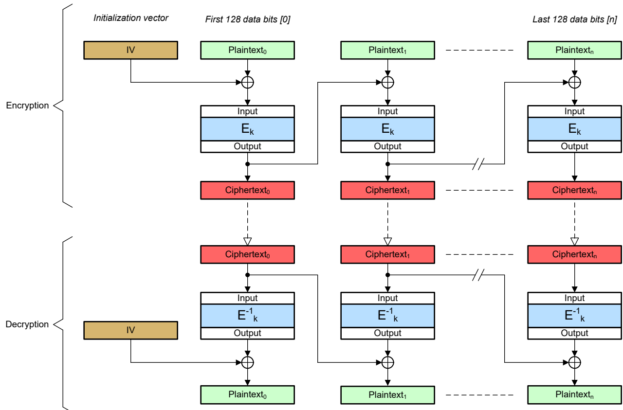
图 11-3. CBC 密码
