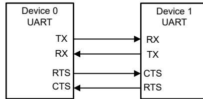
图 19-9. 流控
