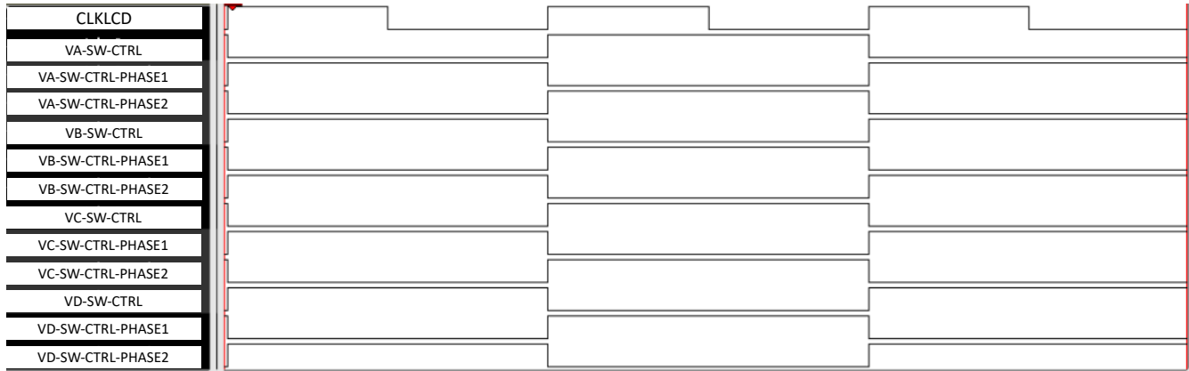
图 24-25. 开关控制信号 - 1/4 偏置模式
