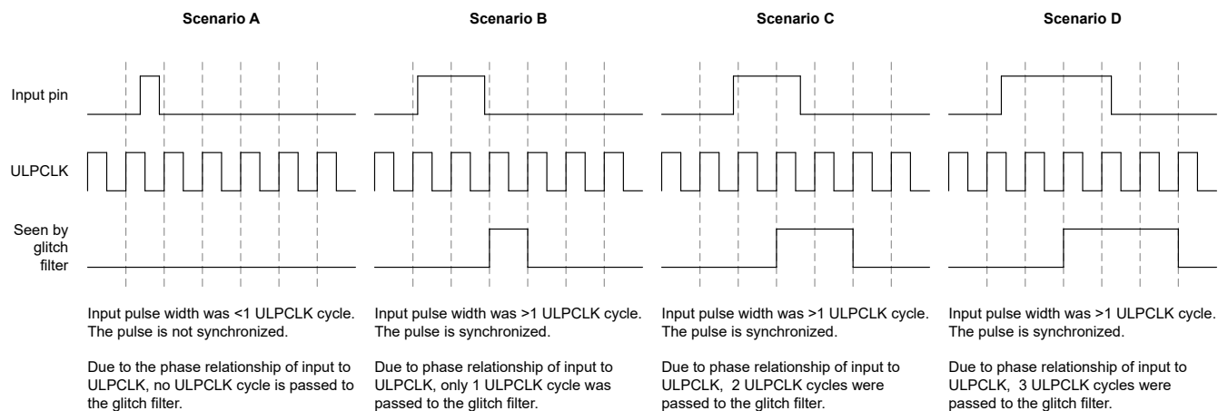
图 13-3. GPIO 输入同步器和干扰滤波场景
