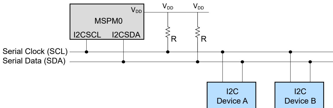
图 21-2. 总线连接图
