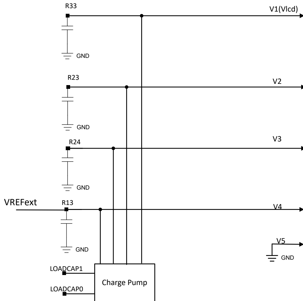
图 24-15. 在模式 6 下生成电压
