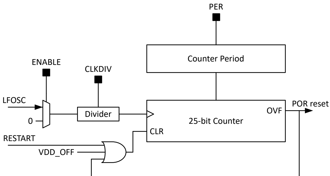
图 26-1. 独立看门狗计时器 (IWDT) 方框图
