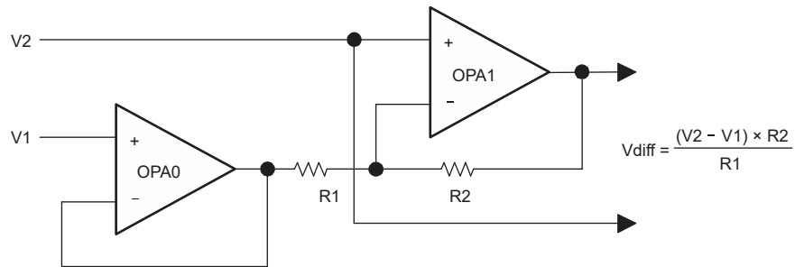
图 16-7. 双 OPA 差分放大器的方框图和公式
