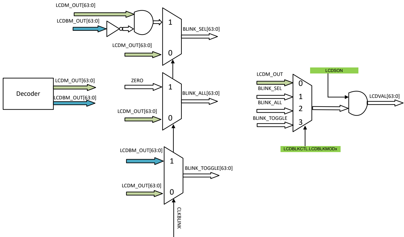
图 24-31. 闪烁覆盖
