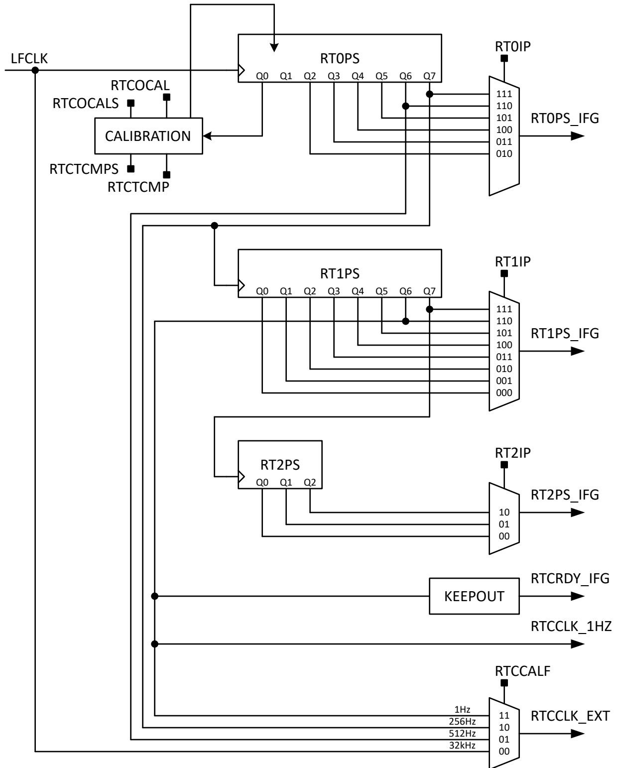
图 25-3. RTC 预分频器和间隔计时器事件
