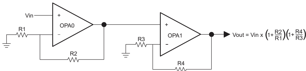
图 16-9. 双 OPA 同相到同相级联放大器的方框图和公式
