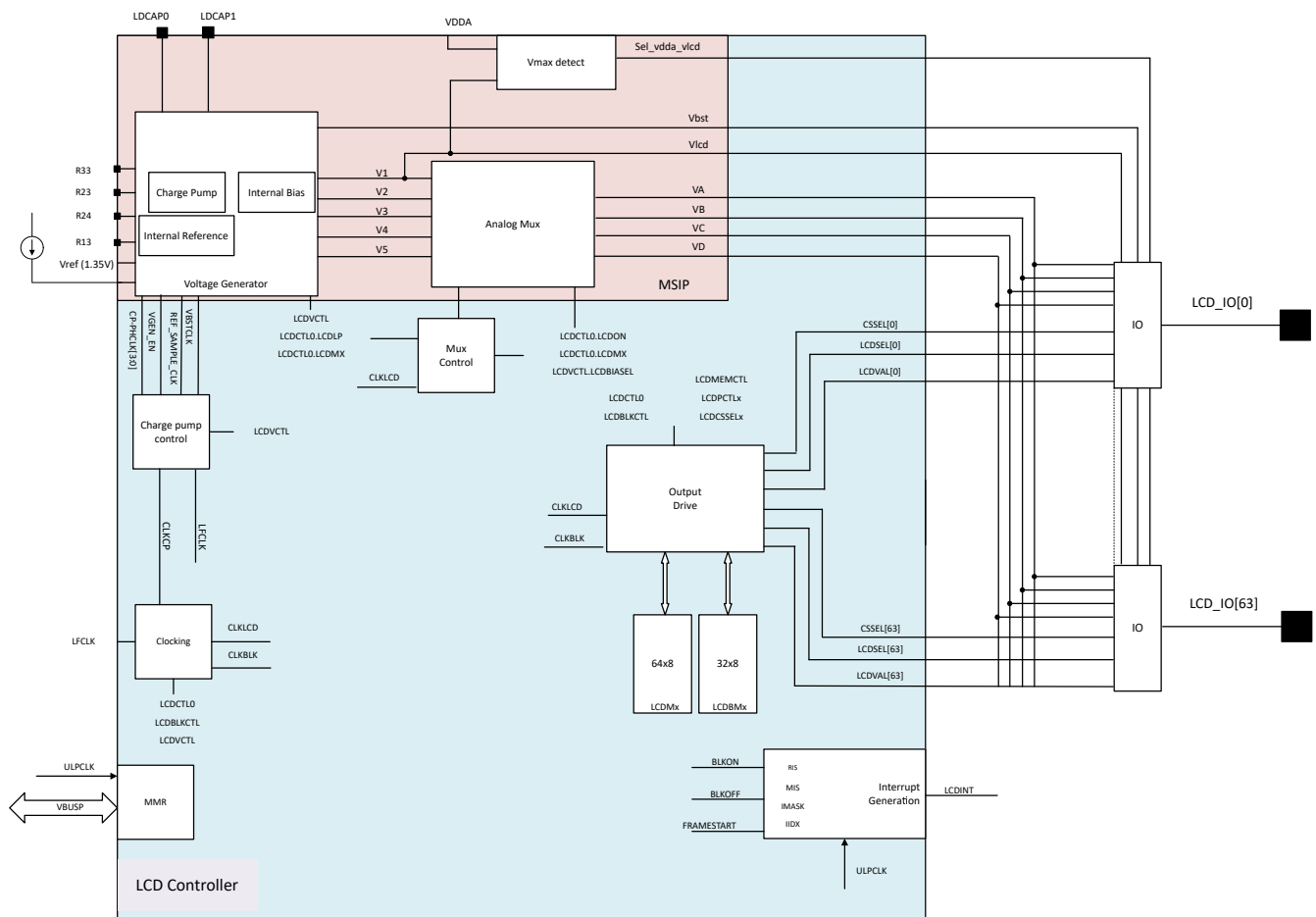
图 24-1. LCD 控制器方框图
