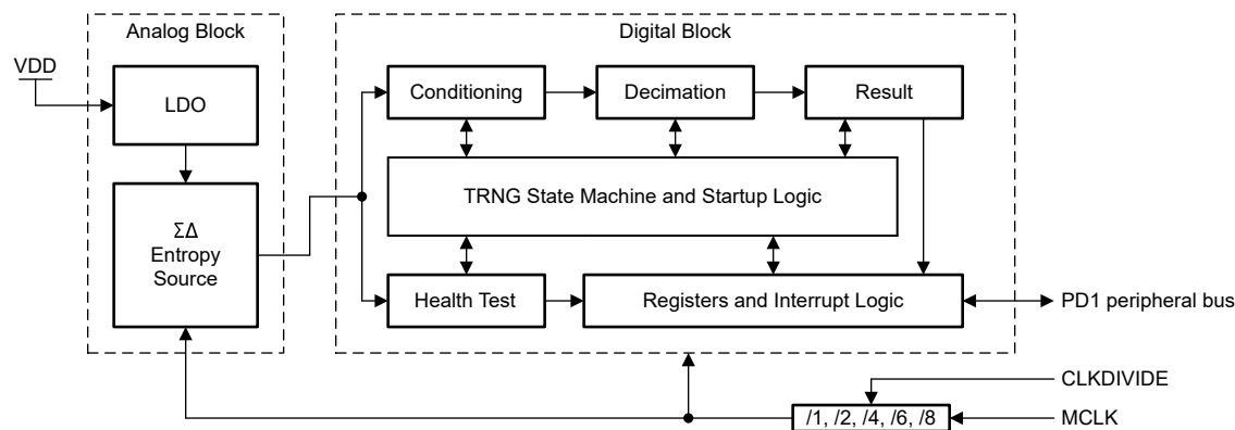
图 10-1. TRNG 方框图
