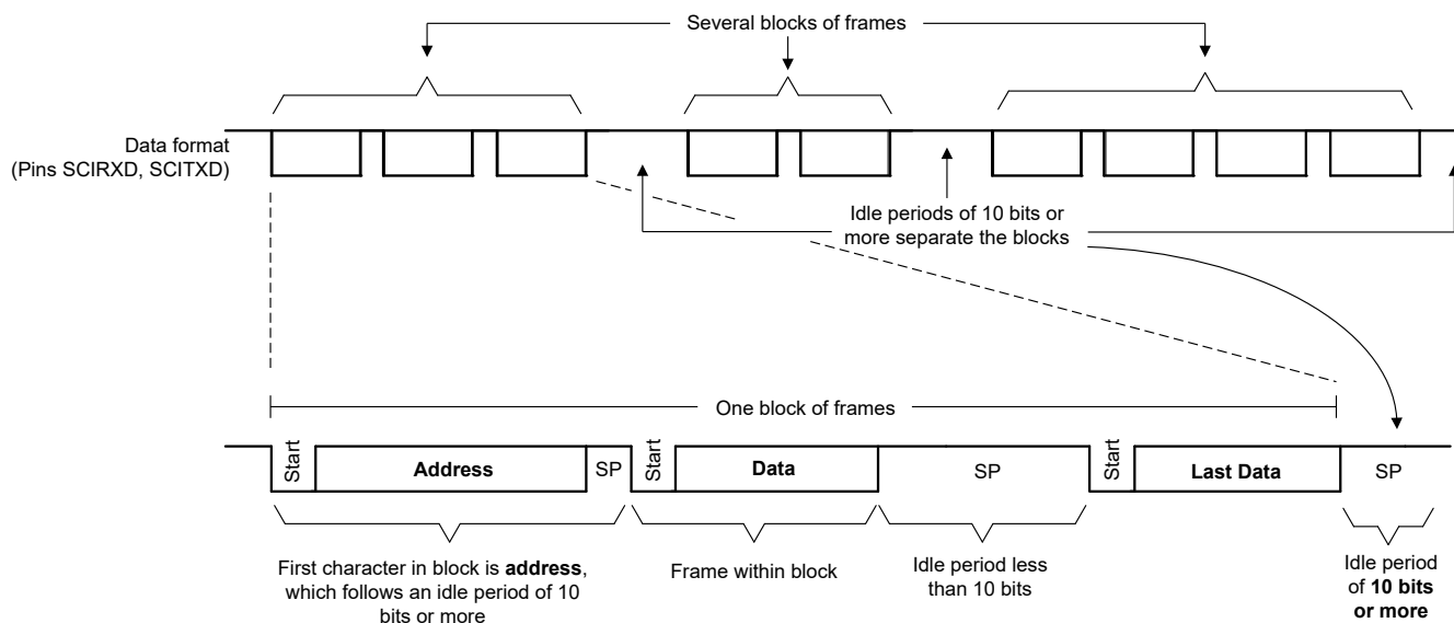
图 19-10. 空闲线多处理器
