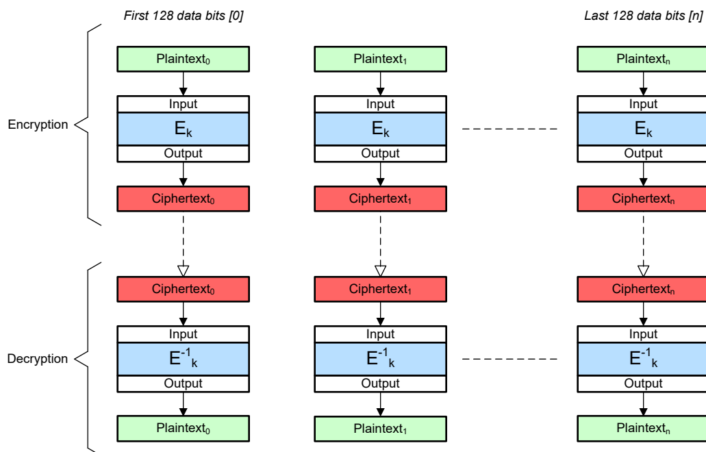
图 11-2. ECB 密码
