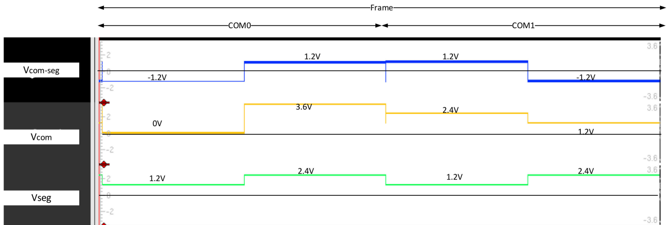
图 24-4. 1/3 偏置段相对于所有 COM0 关闭
