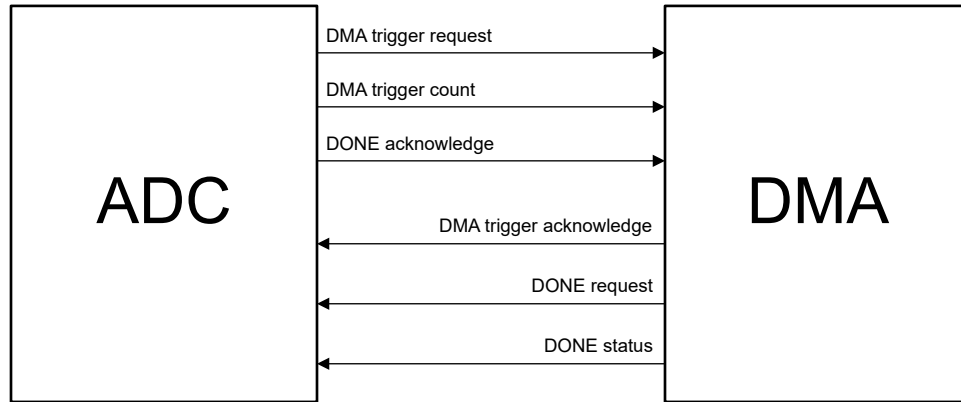
图 14-5. 内部 ADC-DMA 接口
