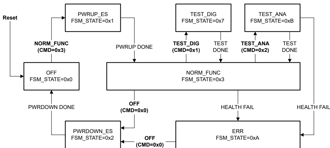
图 10-2. TRNG 状态流程
