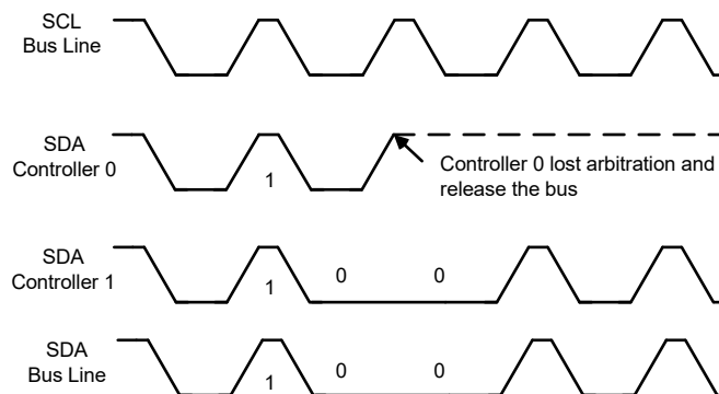
图 21-8. 两个控制器发送器之间的仲裁过程
