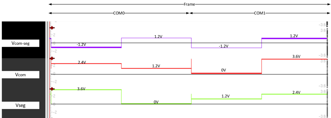
图 24-5. 1/3 偏置段相对于 COM0 关闭
