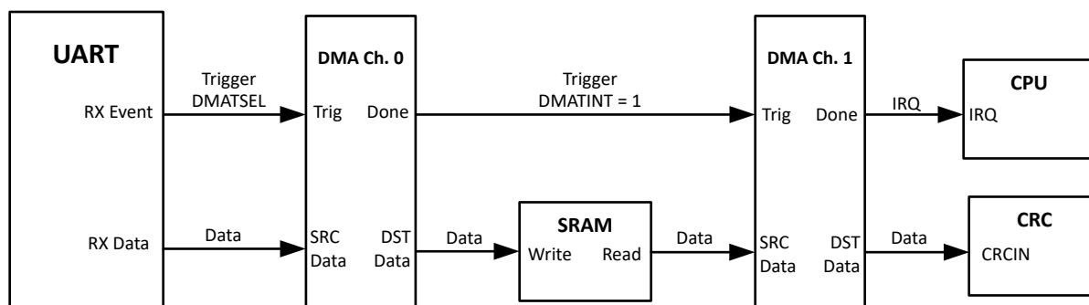
图 5-3. DMA 级联通道
