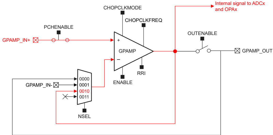
图 17-3. 采用 ADC 缓冲器配置的 GPAMP
