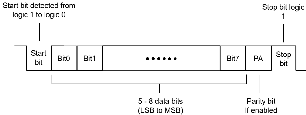
图 19-2. UART 字符帧
