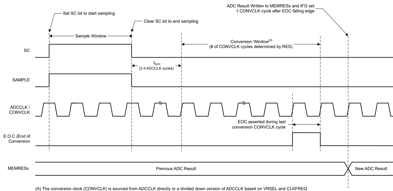
图 14-4. 手动采样模式 ADC 采样和转换时序图
