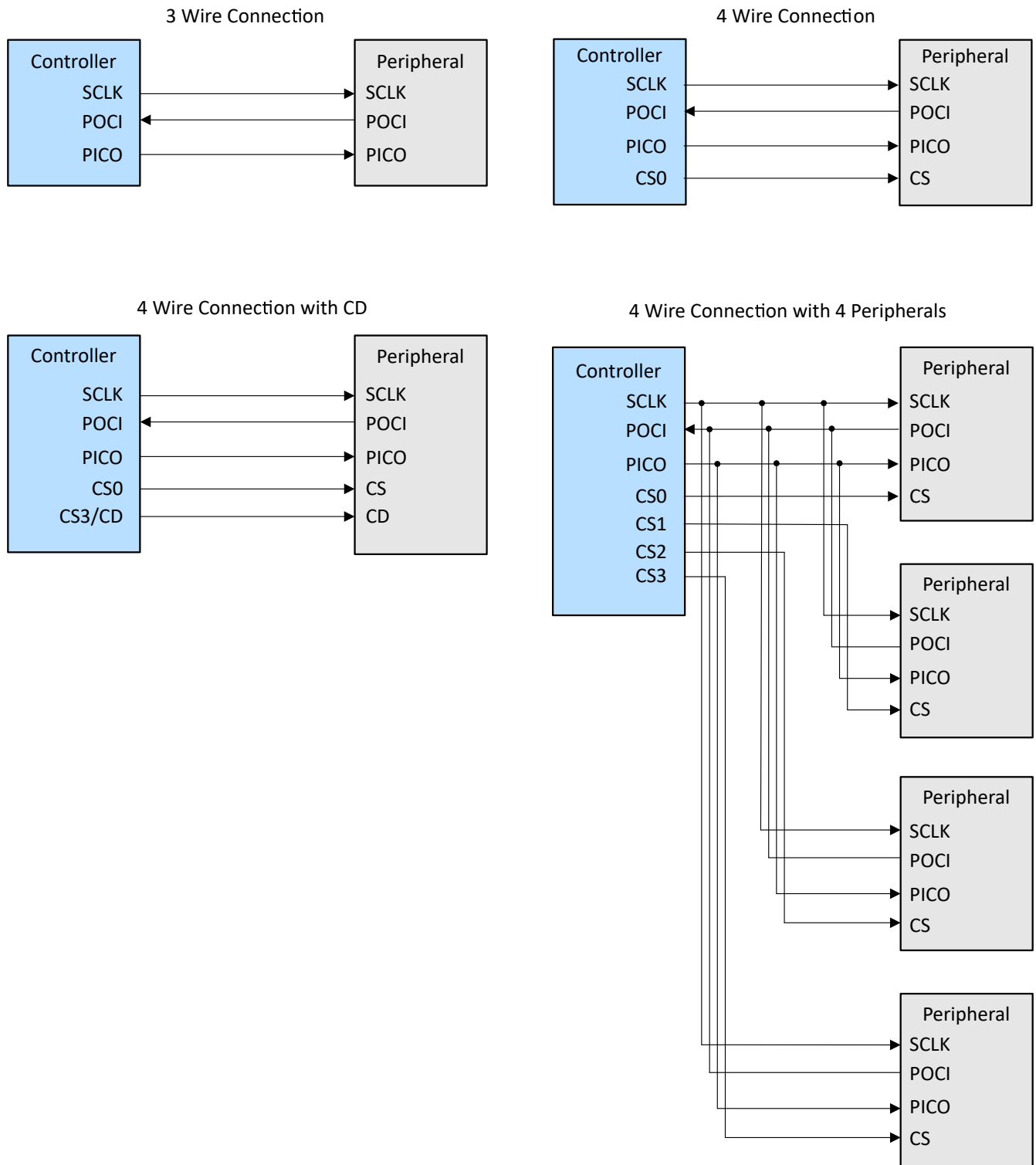
图 20-2. 针对不同 SPI 配置的外部连接
