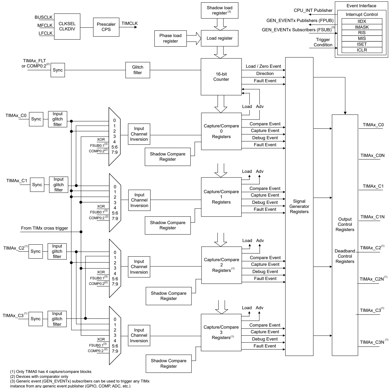
图 23-2. TIMA 方框图
