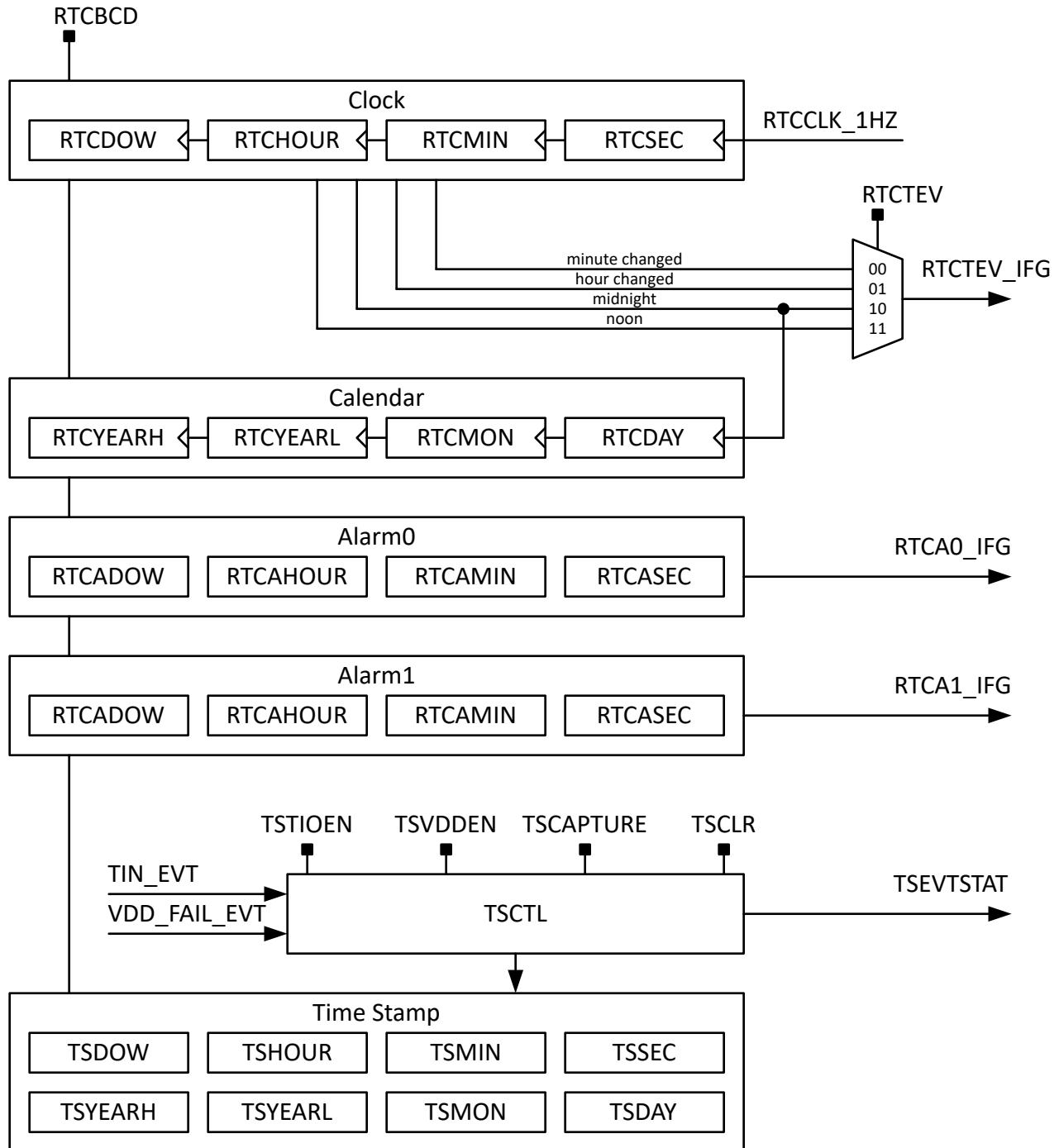
图 25-4. RTC 方框图和时间戳
