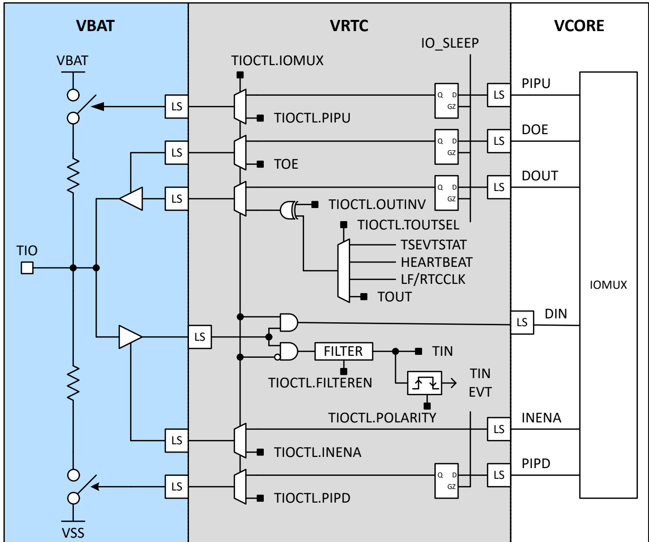
图 8-5. 防篡改 I/O 电路图
