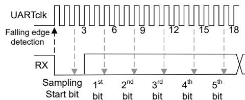
图 19-3. UART 过采样模式
