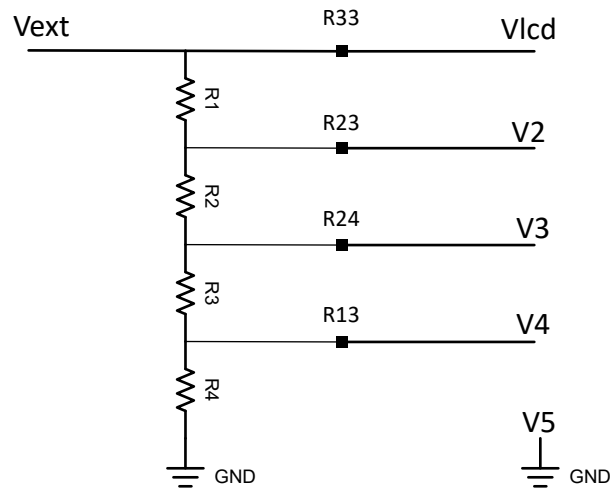
图 24-9. 在模式 0 下生成电压
