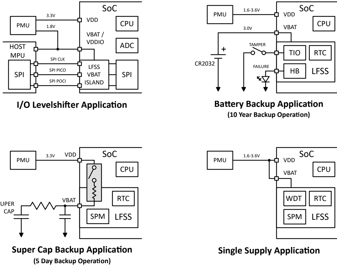
图 8-3. LFSS 典型应用用例
