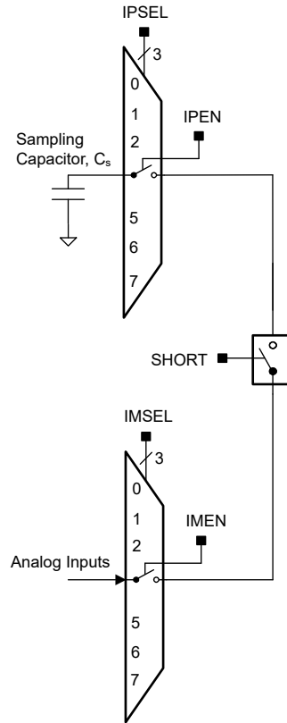
图 15-4. 比较器短路开关
