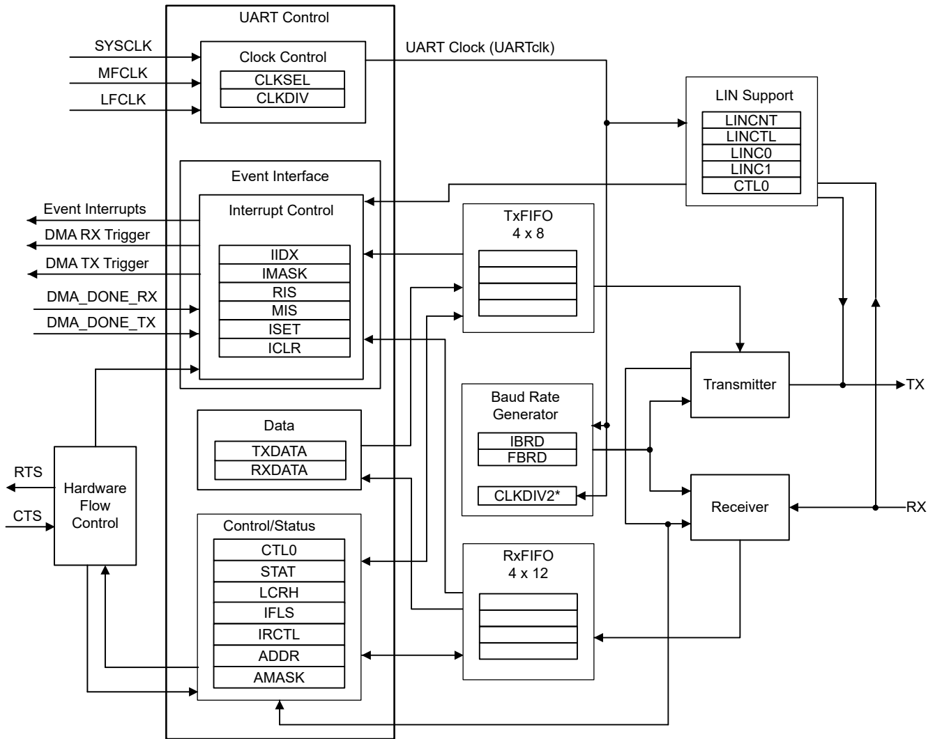
图 19-1. UART 功能方框图
