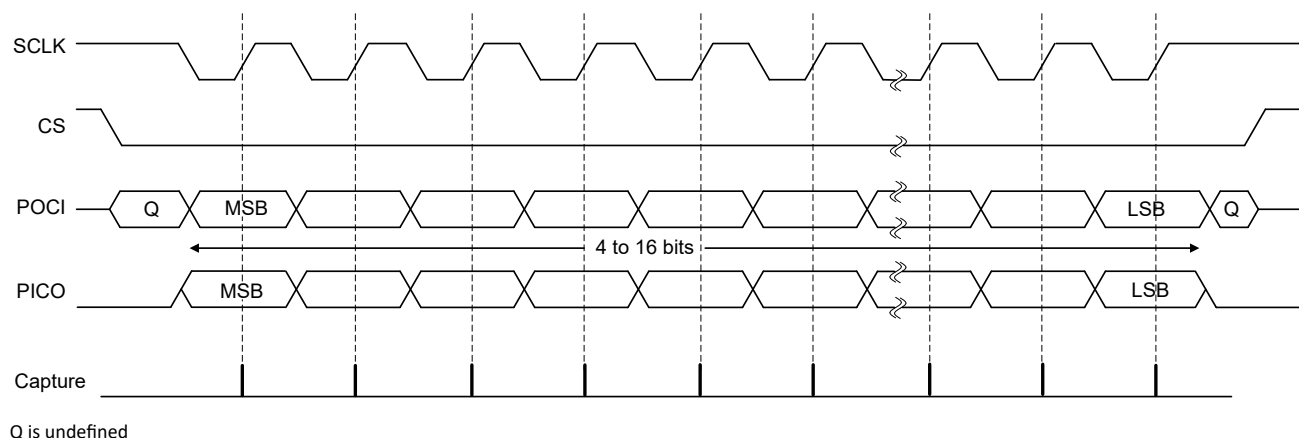
图 20-7. SPO = 1 和 SPH = 1 时的 Motorola SPI 帧格式
