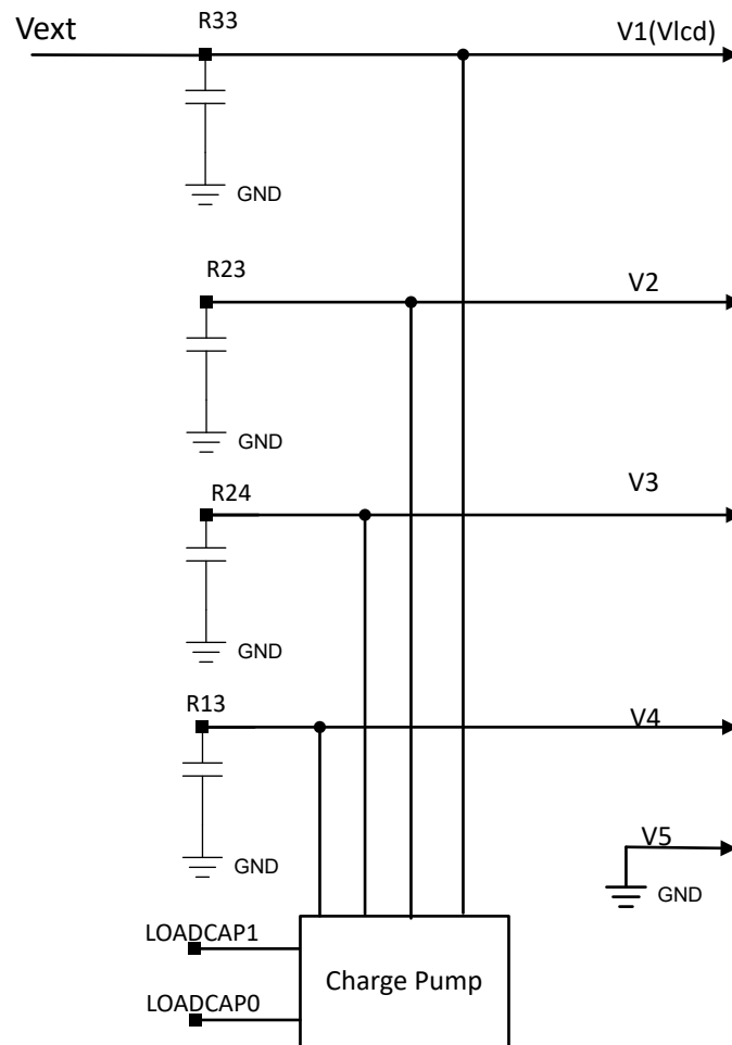
图 24-13. 在模式 4 下生成电压
