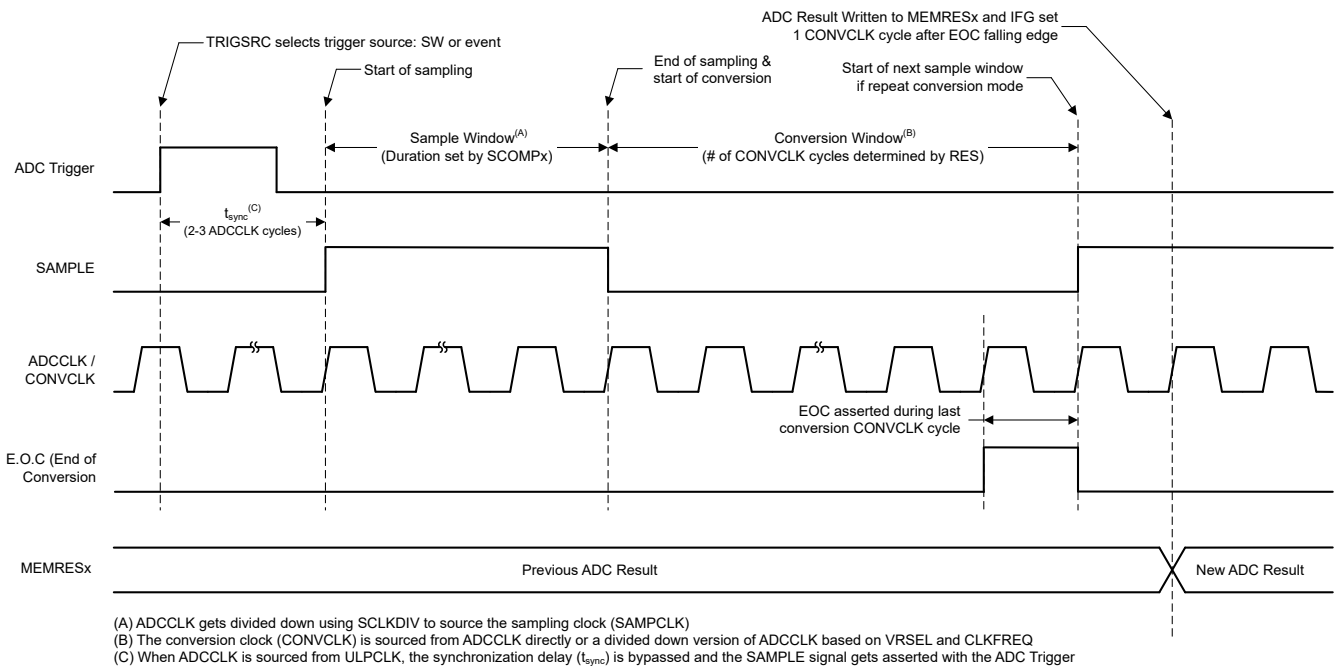
图 14-3. 自动采样模式 ADC 采样和转换时序图
