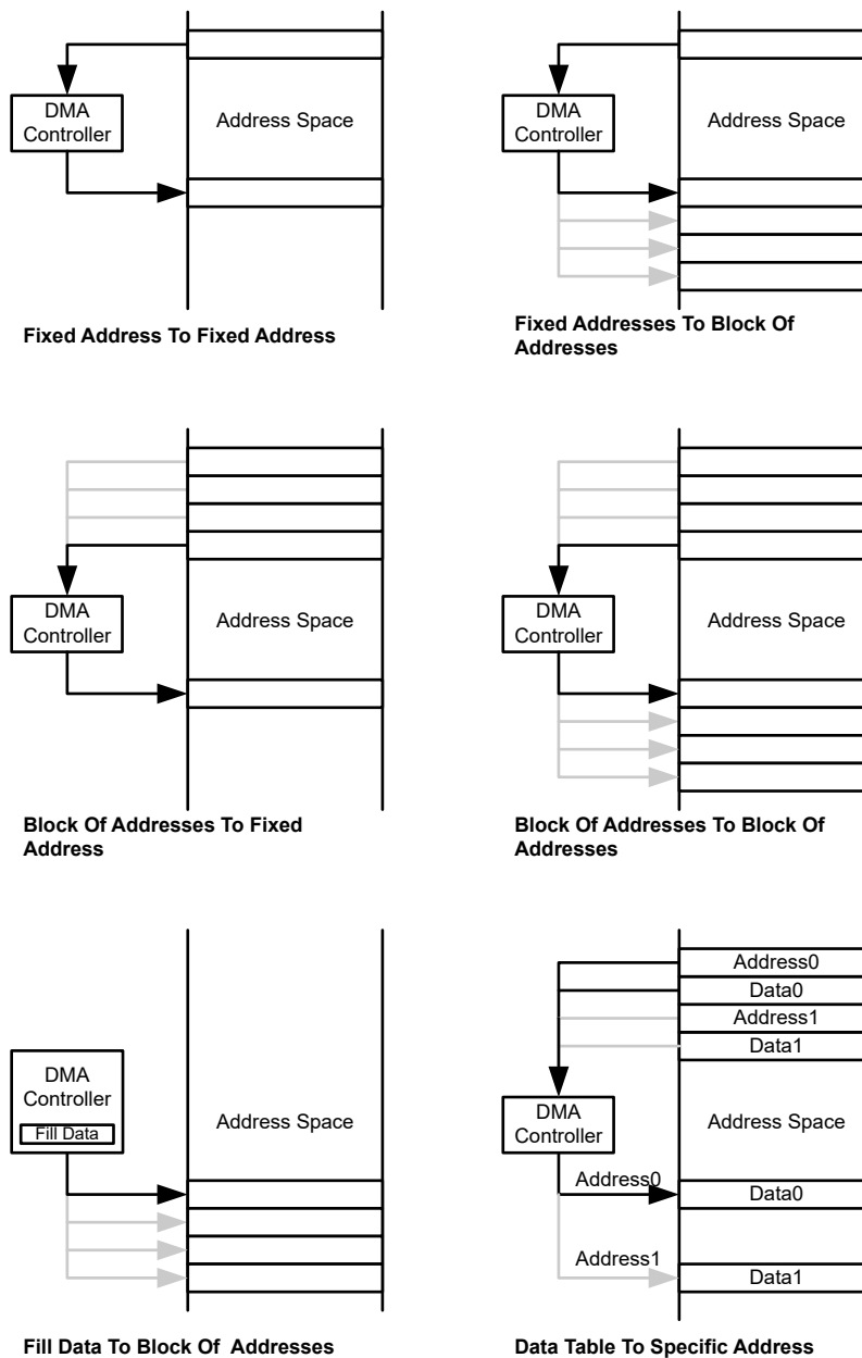
图 5-2. DMA 寻址模式
