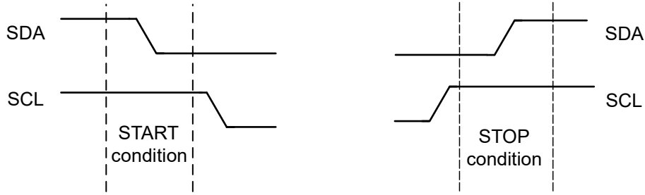
图 21-5. START 和 STOP 条件
