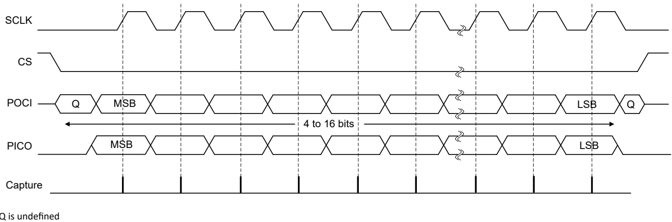
图 20-4. SPO = 0 和 SPH = 0 时的 Motorola SPI 格式
