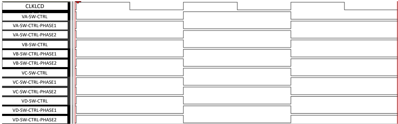
图 24-23. 开关控制信号 - 1/3 偏置模式
