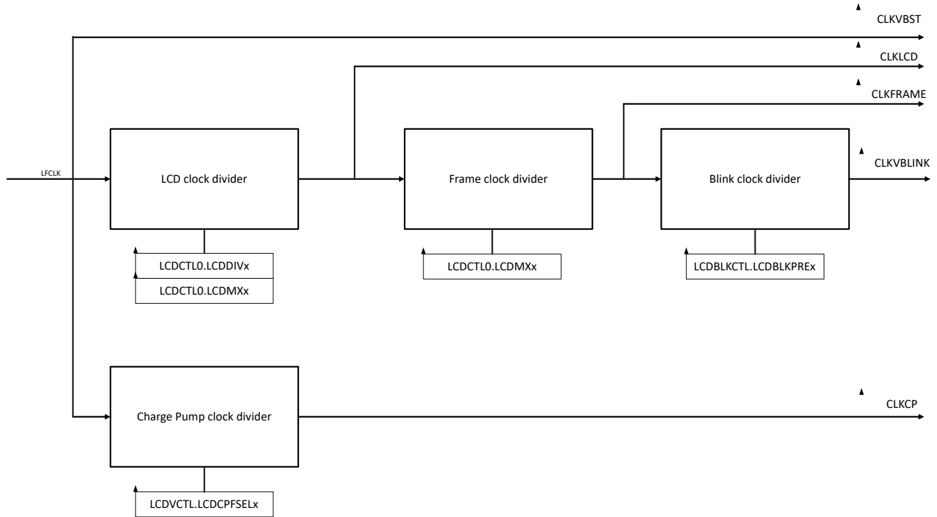
图 24-6. LCD 时钟
