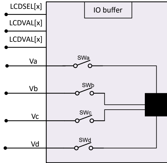
图 24-32. IO 多路复用
