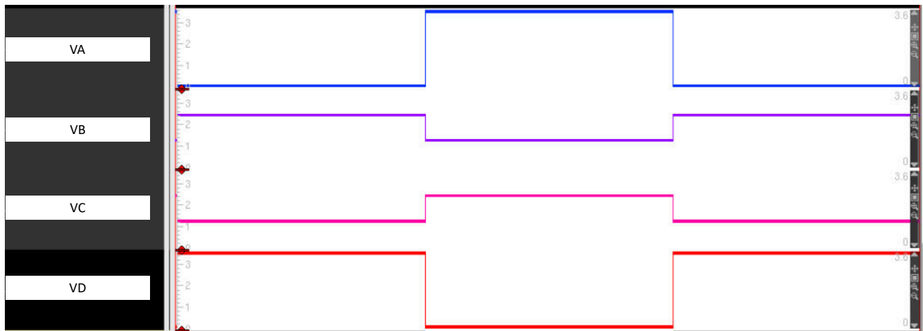
图 24-22. 模拟多路复用器输出 - 1/3 偏置模式
