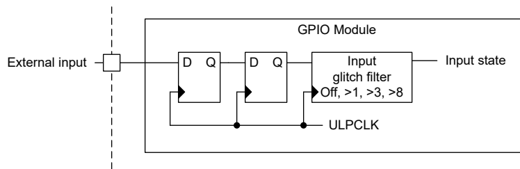
图 13-2. GPIO 输入同步器
