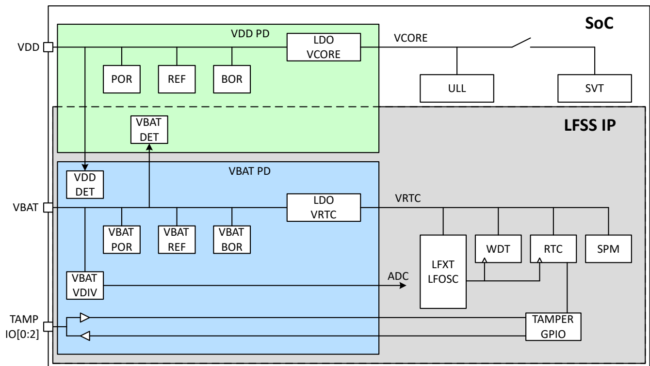
图 8-1. LFSS 概述
