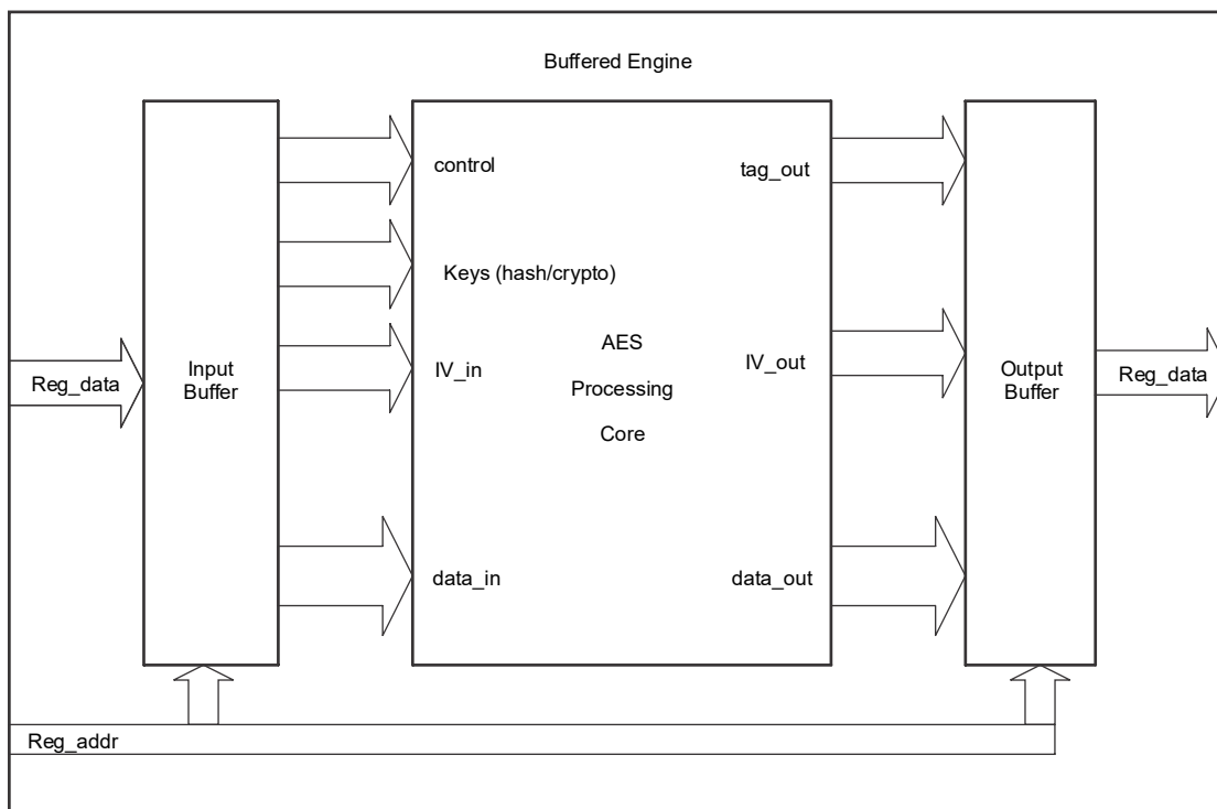
图 11-1. AESADV 方框图
