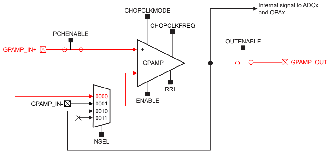
图 17-4. 单位增益配置中的 GPAMP
