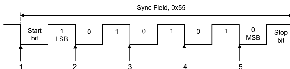
图 19-7. LIN 同步域检测
