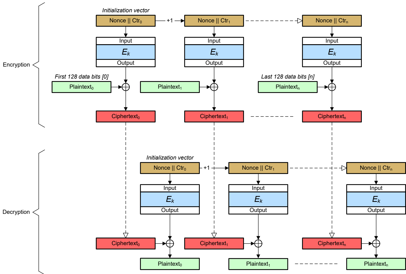
图 11-6. CTR 密码
