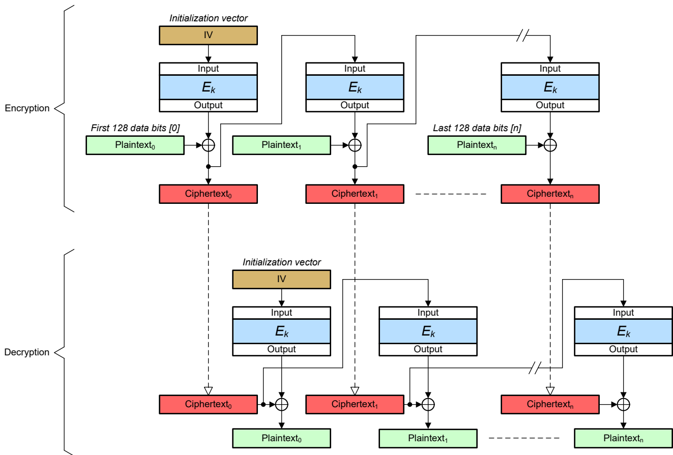
图 11-5. CFB 密码
