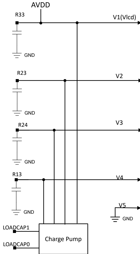
图 24-14. 在模式 5 下生成电压
