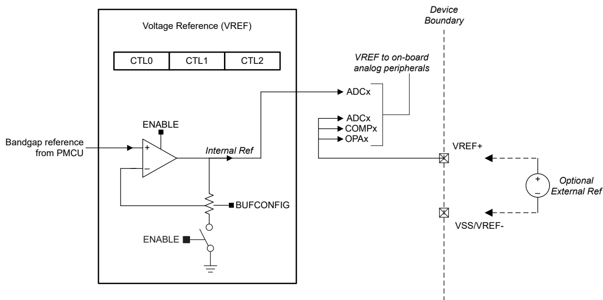
图 18-1. VREF 方框图
