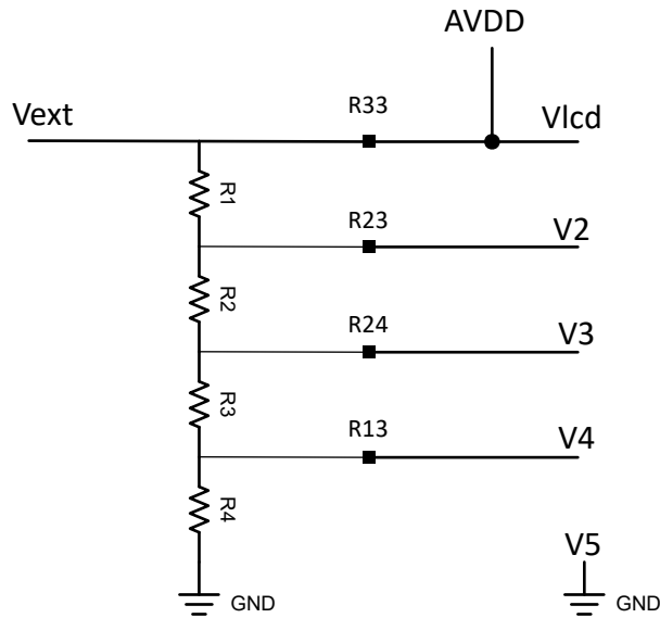
图 24-10. 在模式 1 下生成电压
