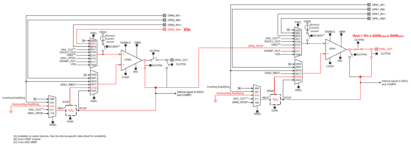
图 16-10. 同相到同相级联放大器配置中的两个 OPA
