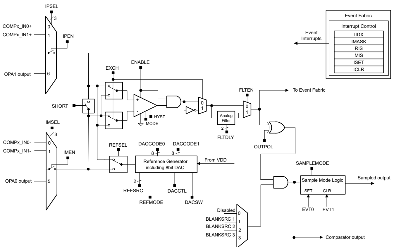
图 15-1. 比较器方框图
