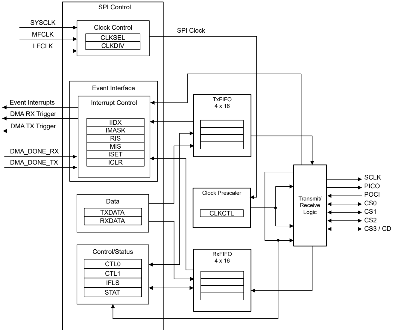
图 20-1. SPI 功能方框图
