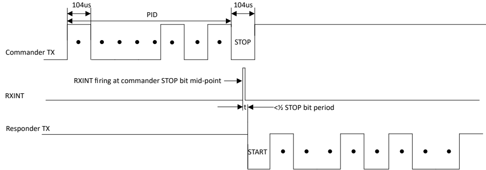
图 19-8. LIN 响应者传输延迟
