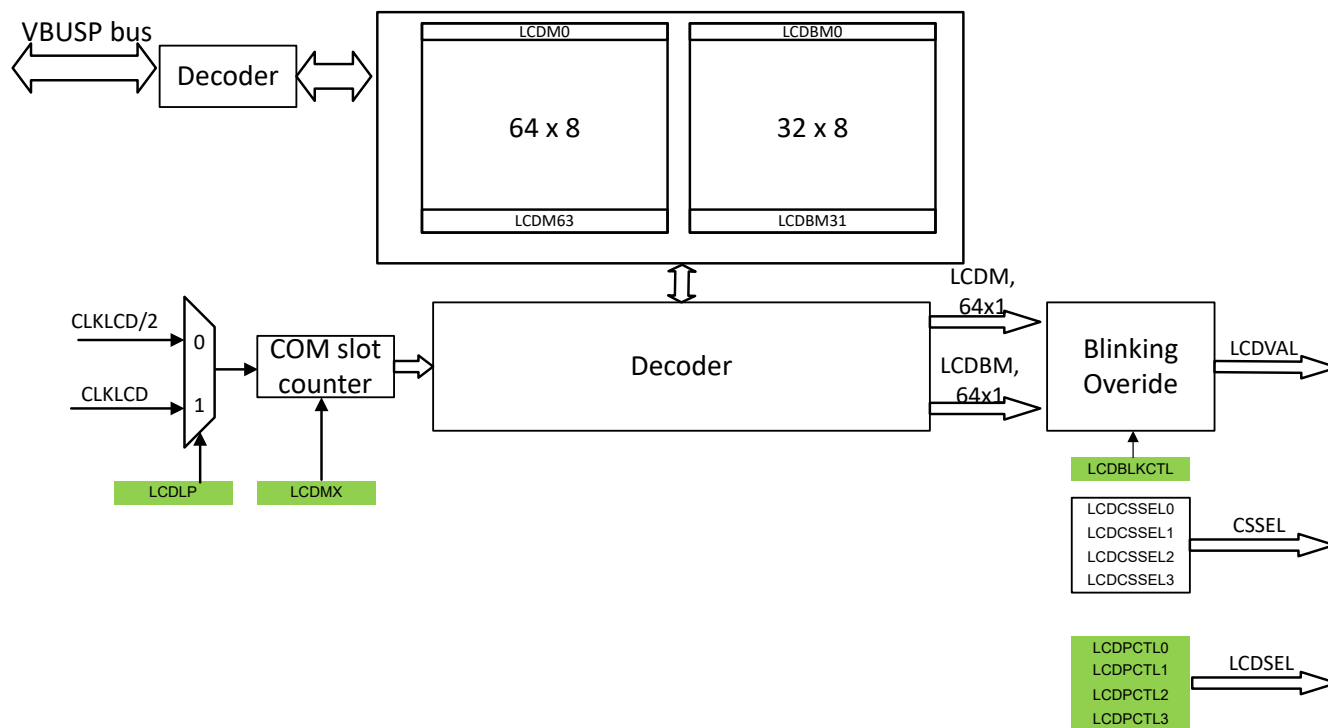
图 24-28. 开关控制信号低功耗模式
