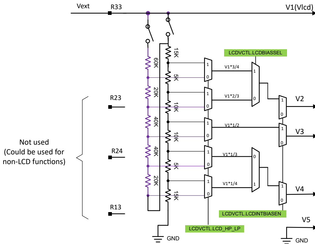
图 24-11. 在模式 2 下生成电压
