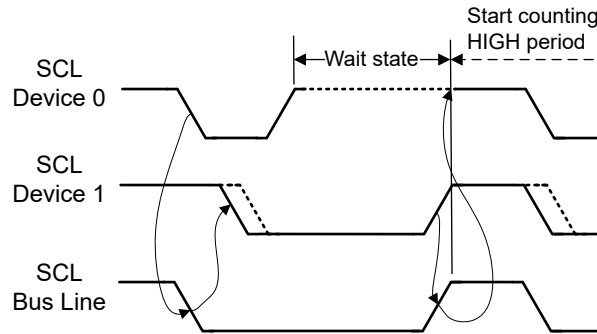
图 21-9. 时钟同步
