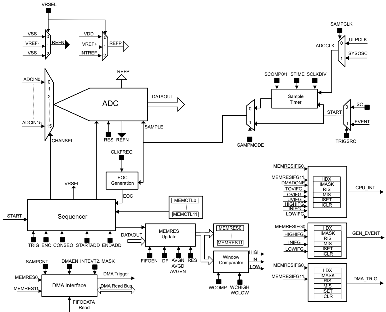
图 14-1. ADC 方框图
