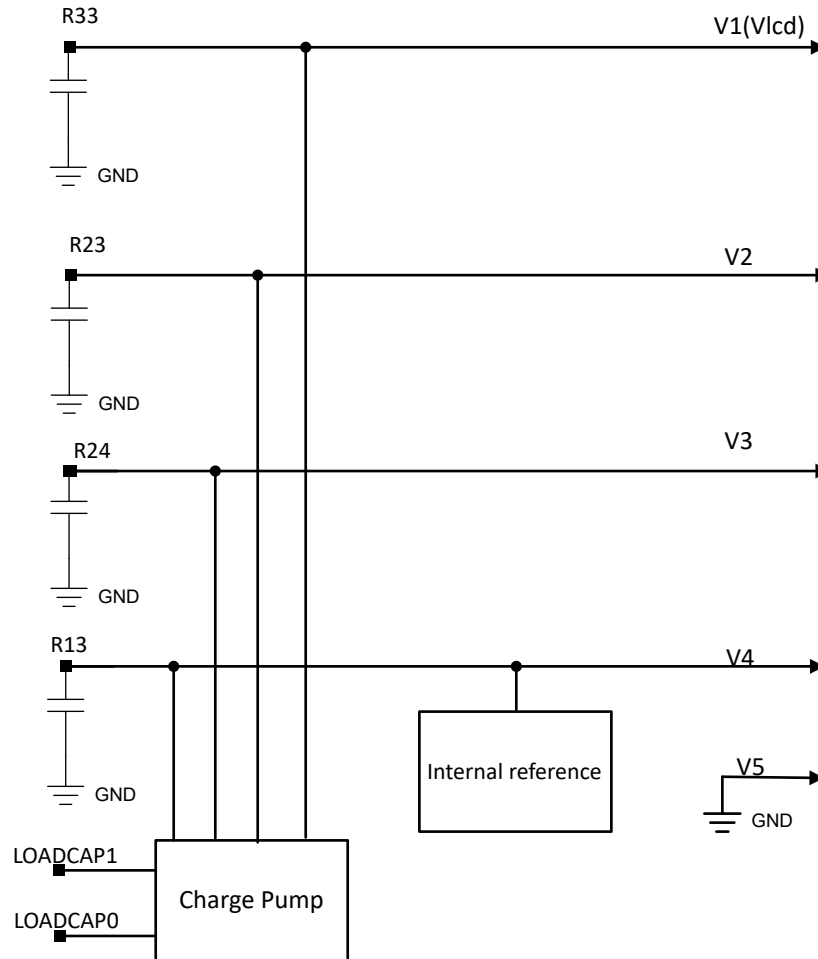
图 24-16. 在模式 7 下生成电压
