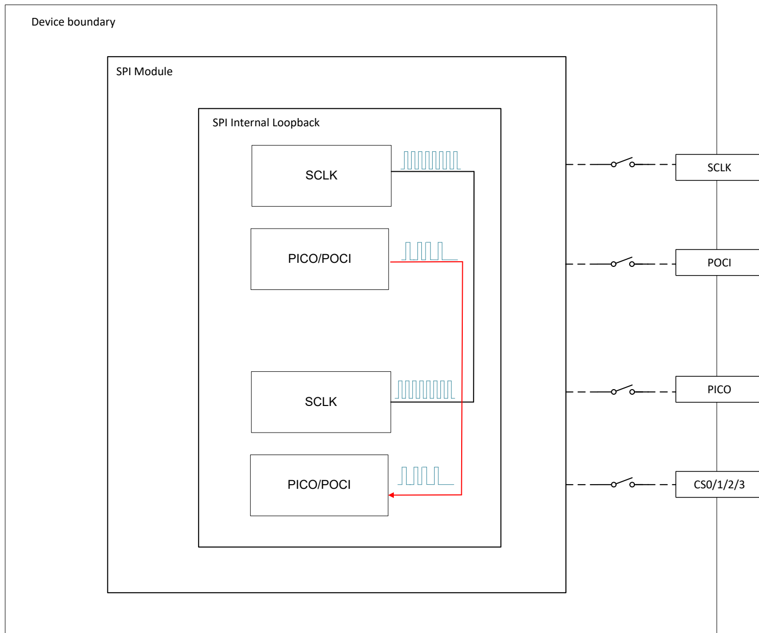
图 20-3. 内部环回模式
