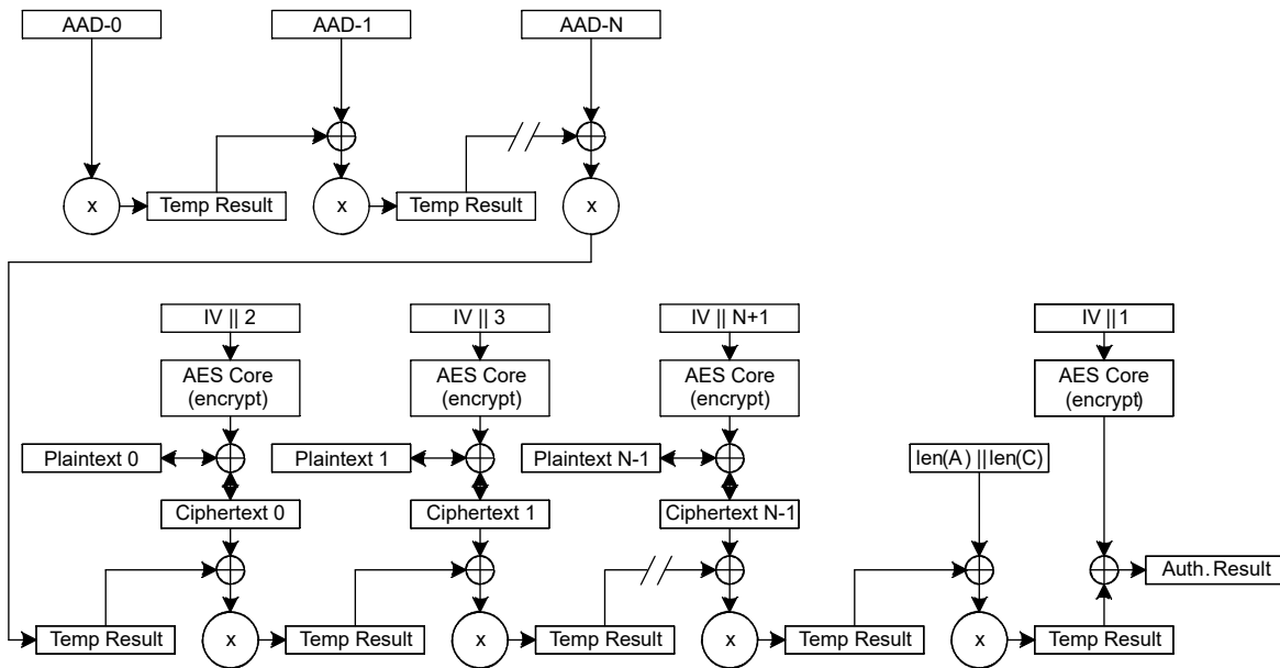
图 11-7. GCM 协议操作
