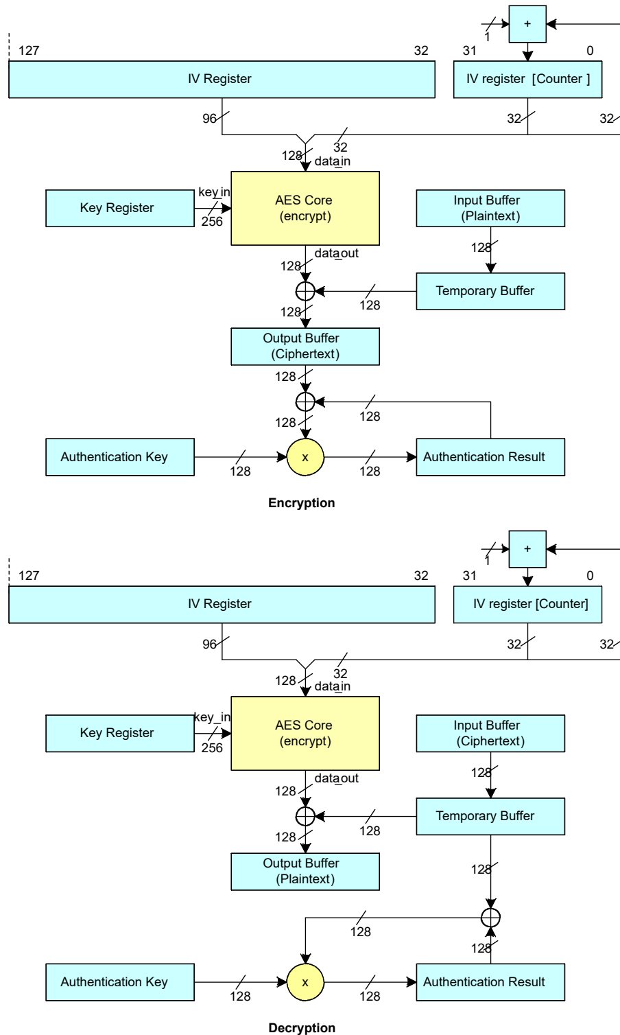
图 11-8. 数据块的 GCM 操作
