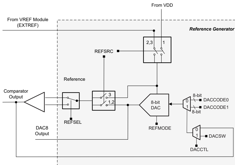
图 15-3. 基准电压发生器方框图
