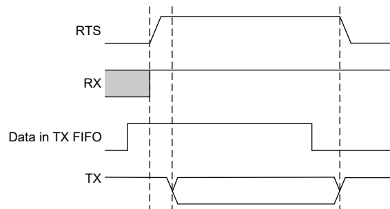
图 19-11. RS485 数据交换
