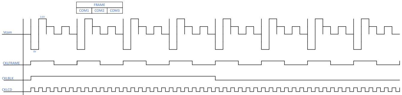
图 24-7. CLKLCD、CLKFRAME 和 CLKBLK 关系
