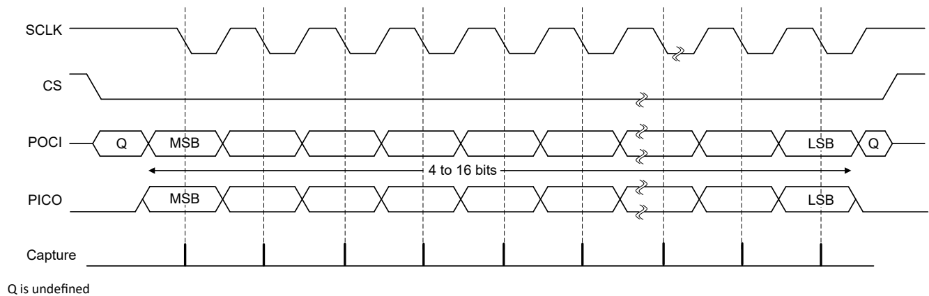
图 20-6. SPO = 1 和 SPH = 0 时的 Motorola SPI 帧格式
