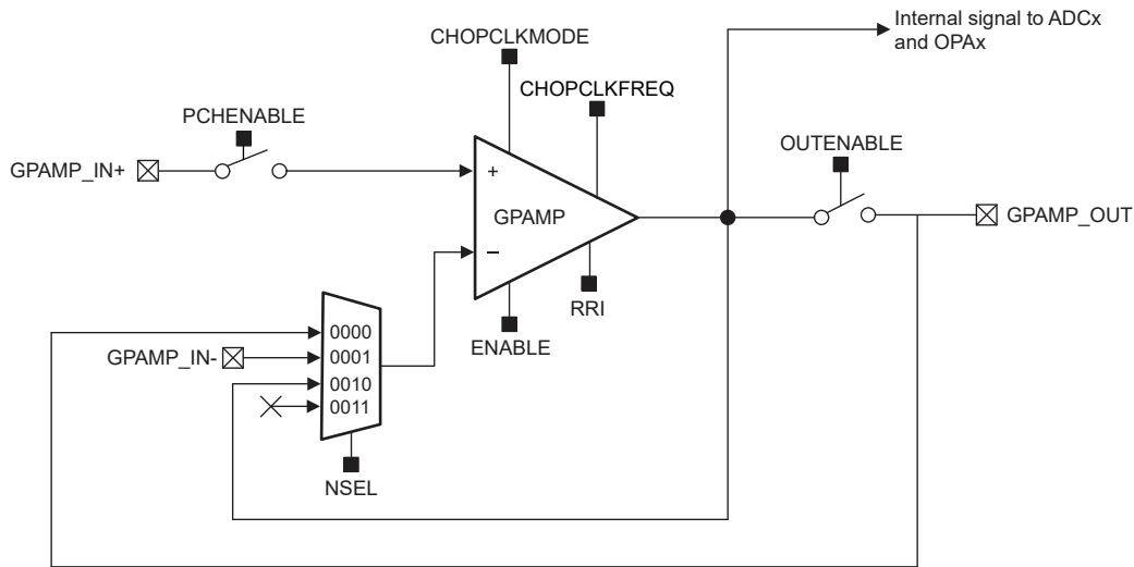
图 17-1. GPAMP 方框图
