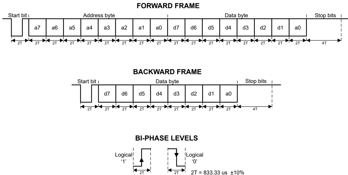
图 19-13. DALI 协议
