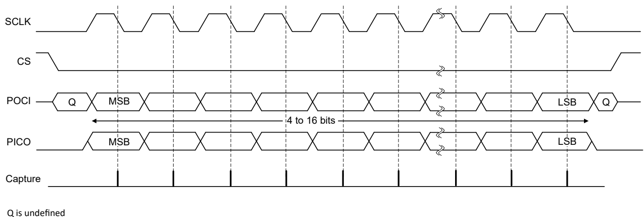
图 20-5. SPO = 0 和 SPH = 1 时的 Motorola SPI 帧格式
