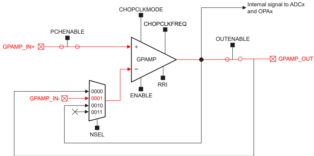
图 17-2. 通用 (GP) 模式下的 GPAMP
