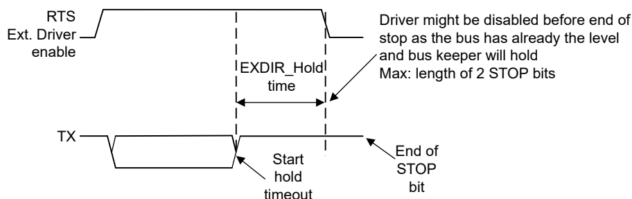
图 19-12. RS485 外部控制
