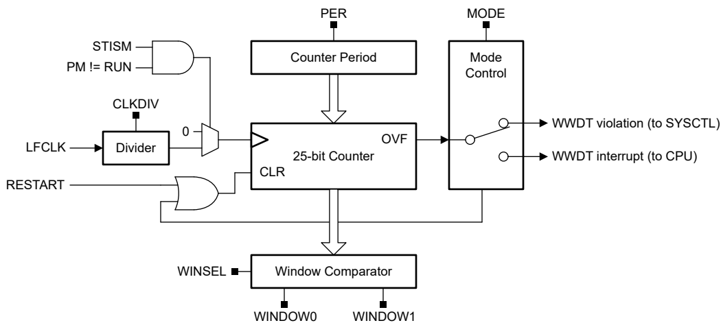
图 27-2. WWDT 方框图
