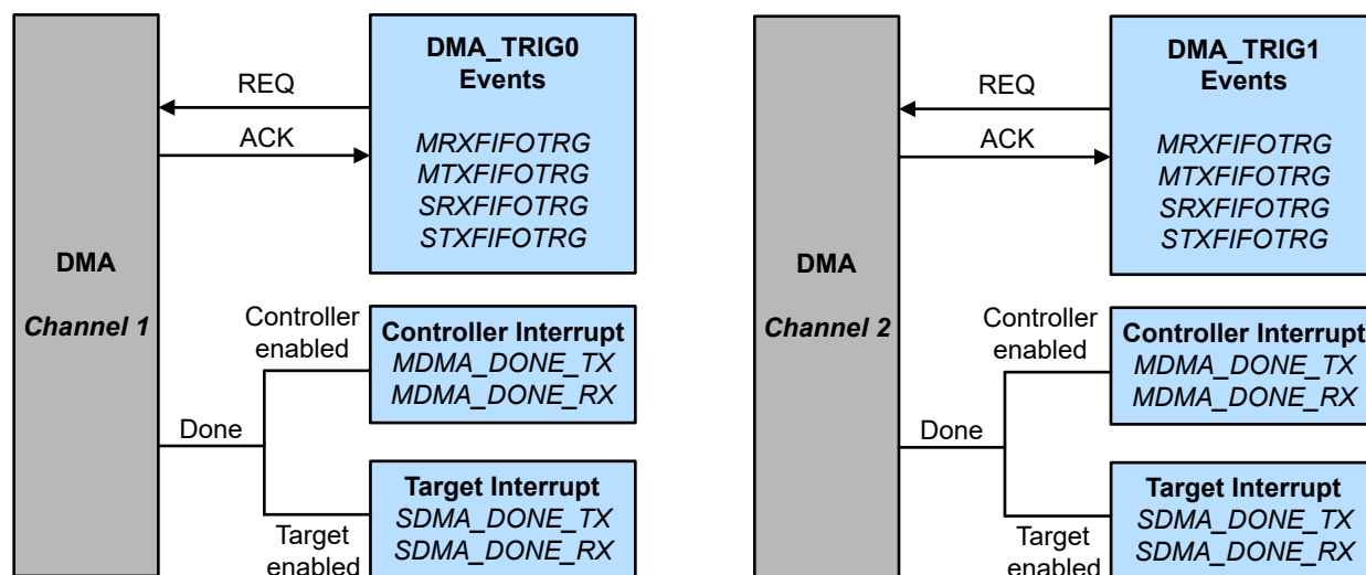
图 21-17. I 2 C DMA 触发和状态
