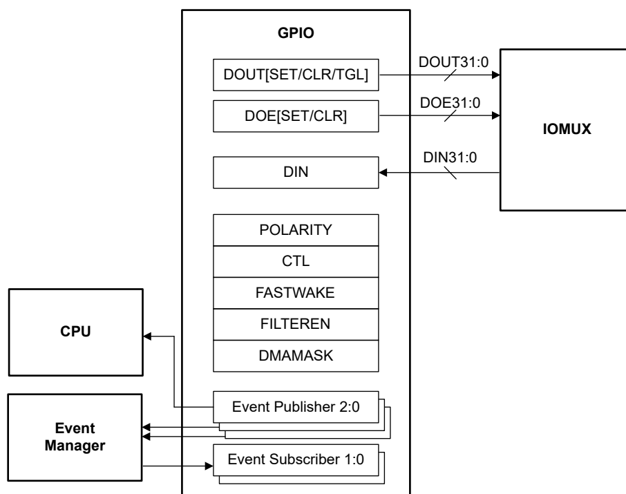
图 13-1. GPIO 方框图
