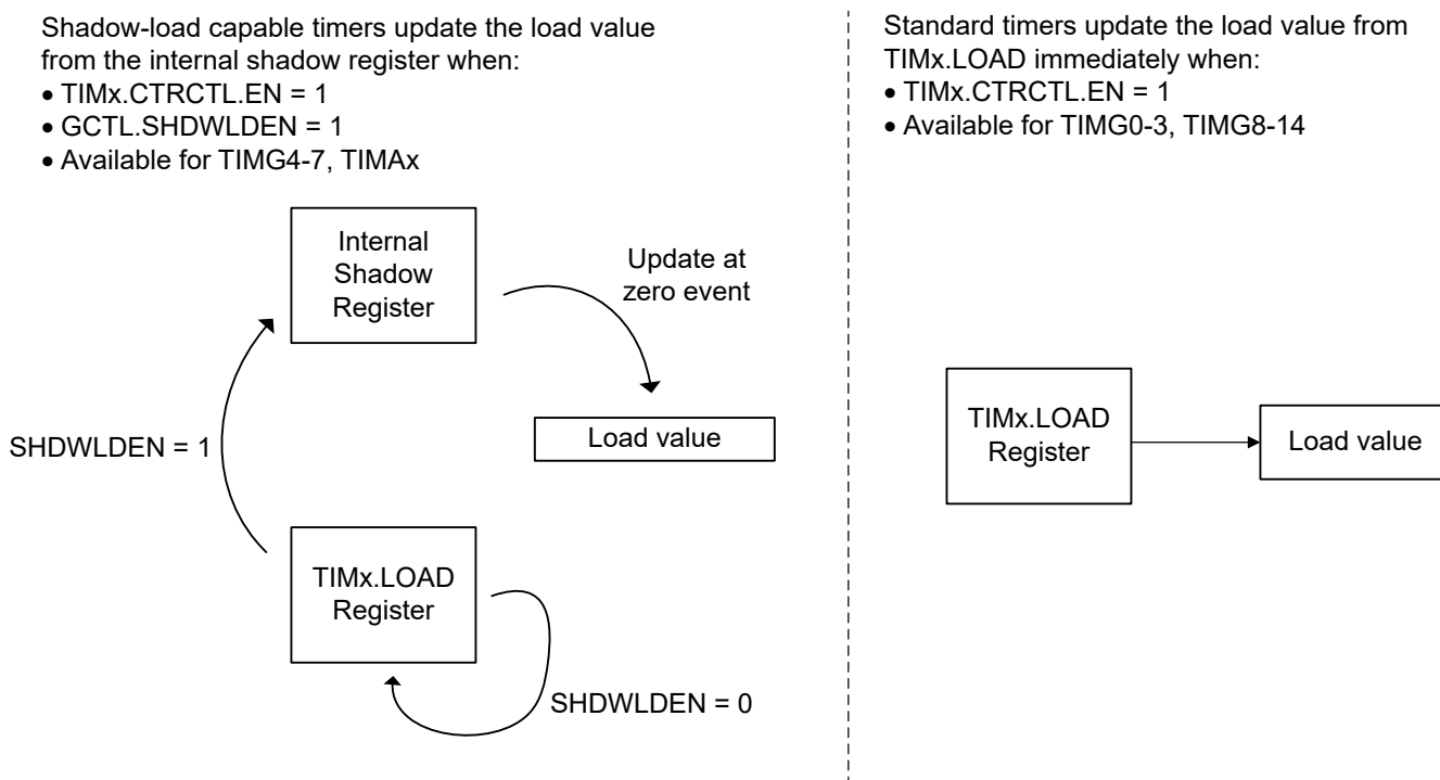
图 23-24. 当 EN=1 时 TIMx 实例的加载值更新
