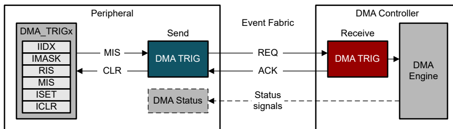
图 7-2. DMA 路由
