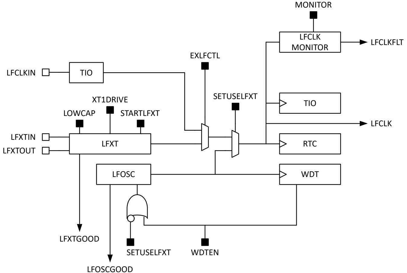
图 8-2. LFSS 低频时钟系统
