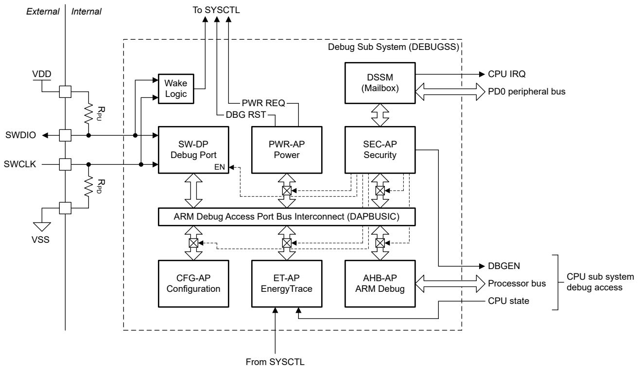
图 28-1. 调试子系统方框图
