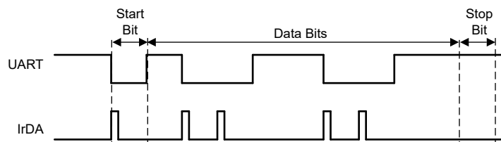
图 19-14. IrDA 协议
