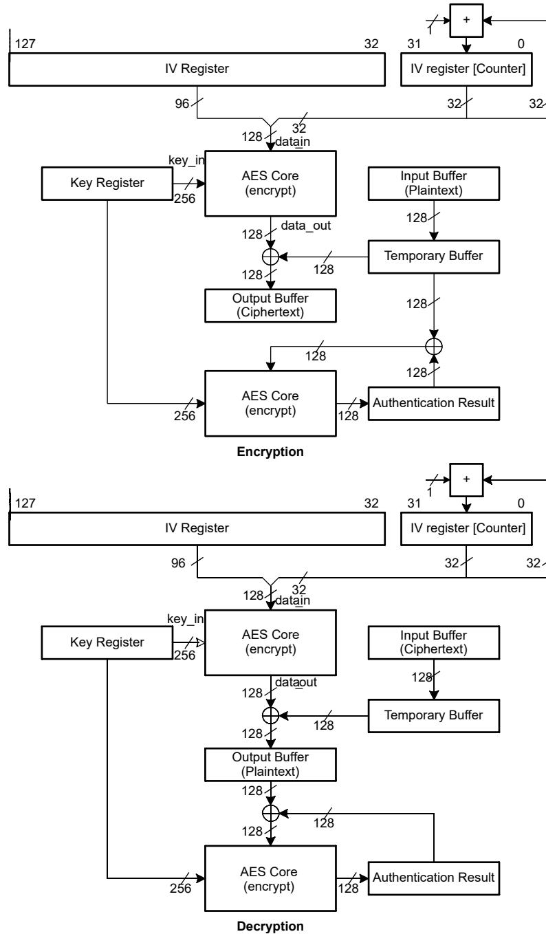
图 11-10. CCM 操作
