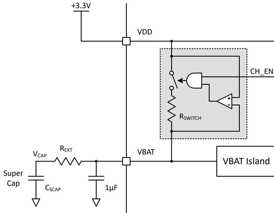
图 8-4. 超级电容器充电电路
