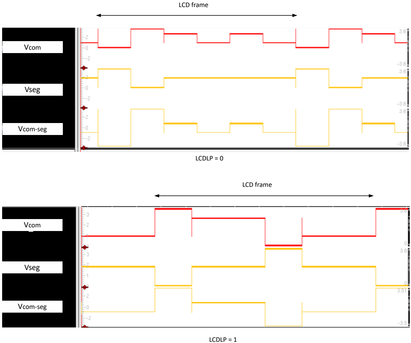
图 24-27. 开关控制信号
