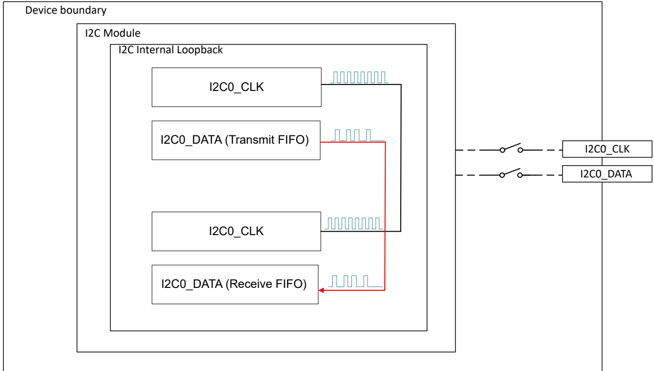
图 21-10. I 2 C 内部环回模式
