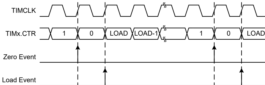
图 23-6. 向下计数模式事件生成
