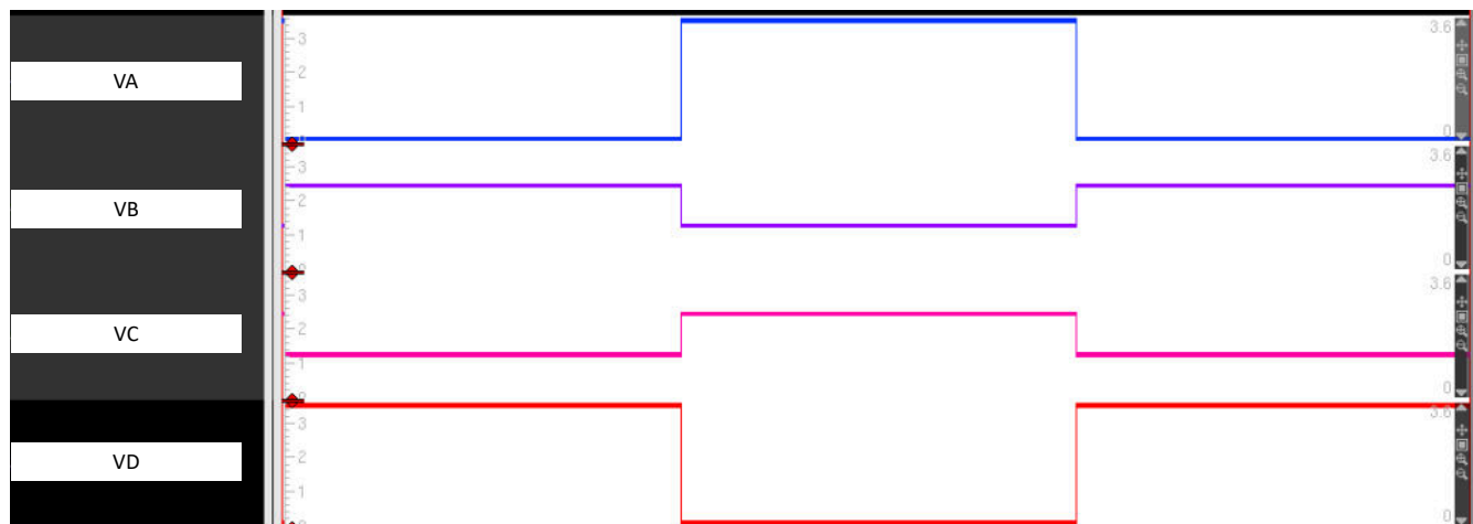
图 24-20. 模拟多路复用器输出 - 静态模式
