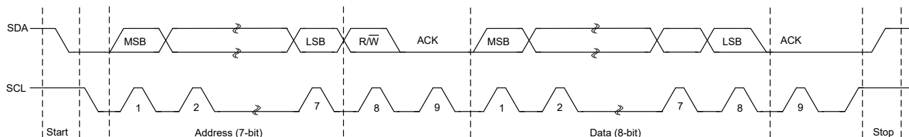
图 21-3. 模块数据传输
