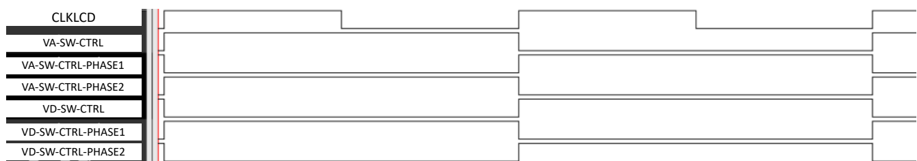
图 24-21. 开关控制信号 - 静态模式
