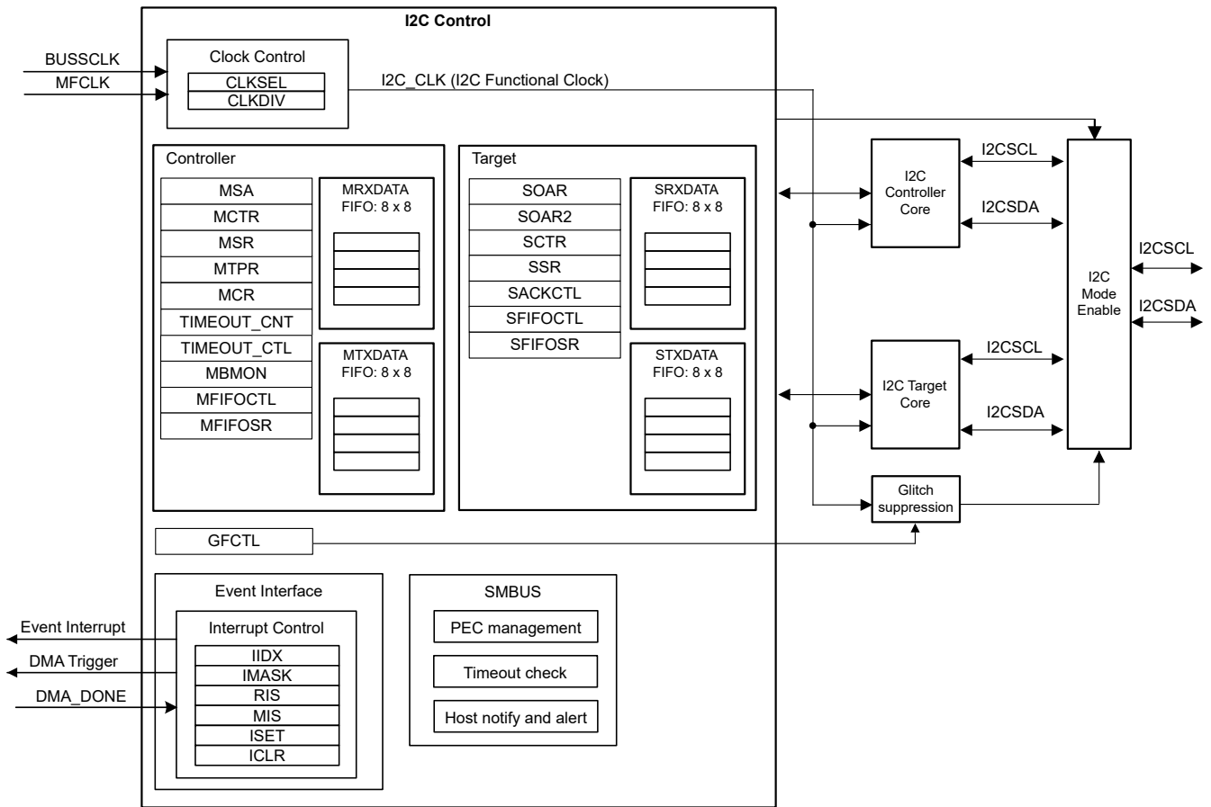
图 21-1. I2C 功能方框图
