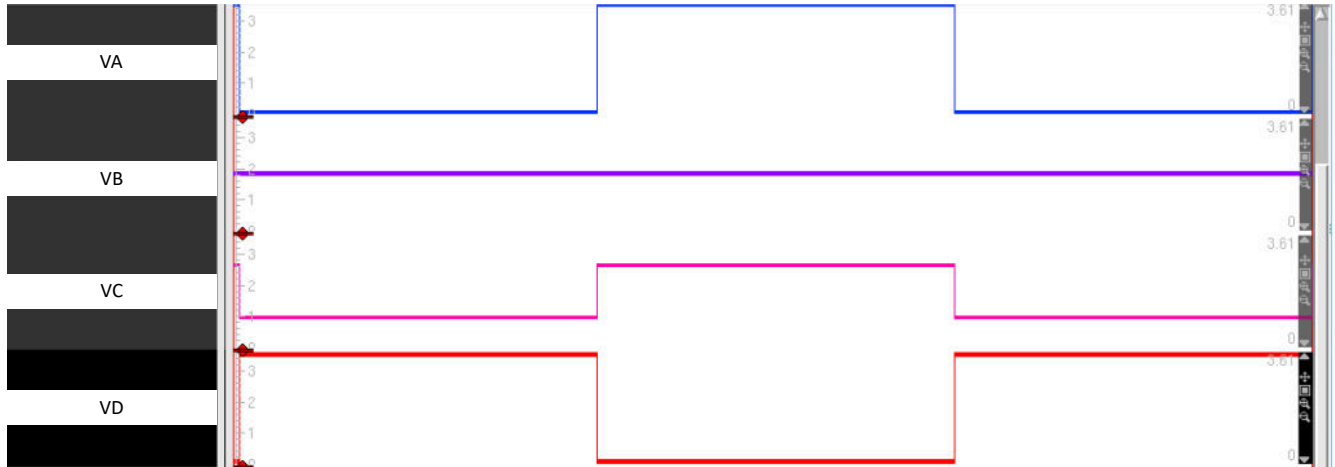
图 24-24. 模拟多路复用器输出 - 1/4 偏置模式
