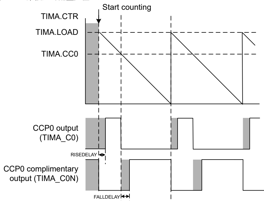
图 23-32. 向下计数模式下的 PWM 的死区插入 ( 模式 0 )
