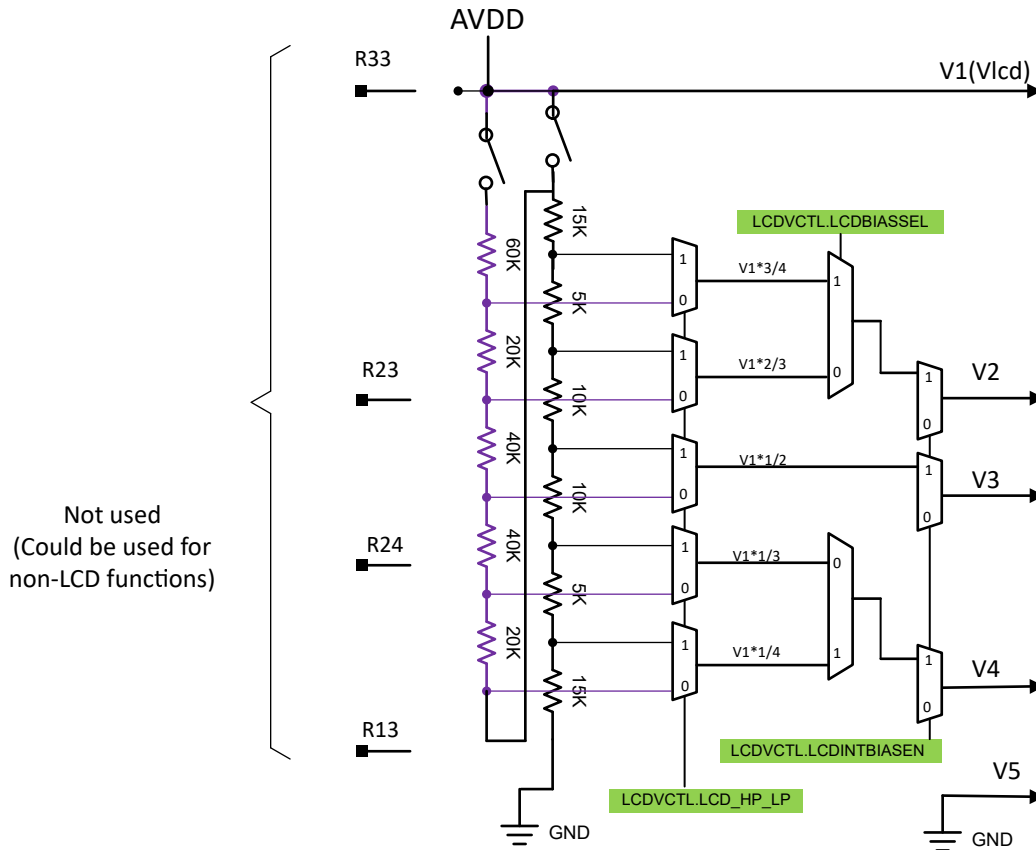
图 24-12. 在模式 3 下生成电压
