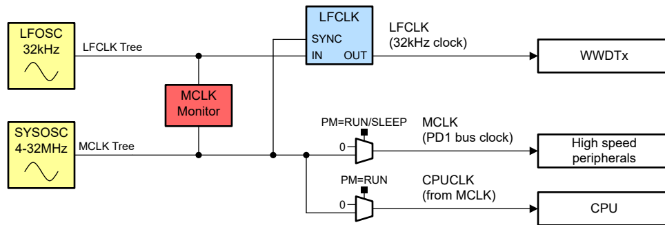
图 27-3. WWDT 简化时钟源树
