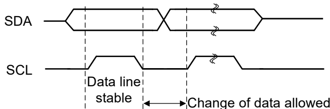
图 21-4. 数据更改周期
