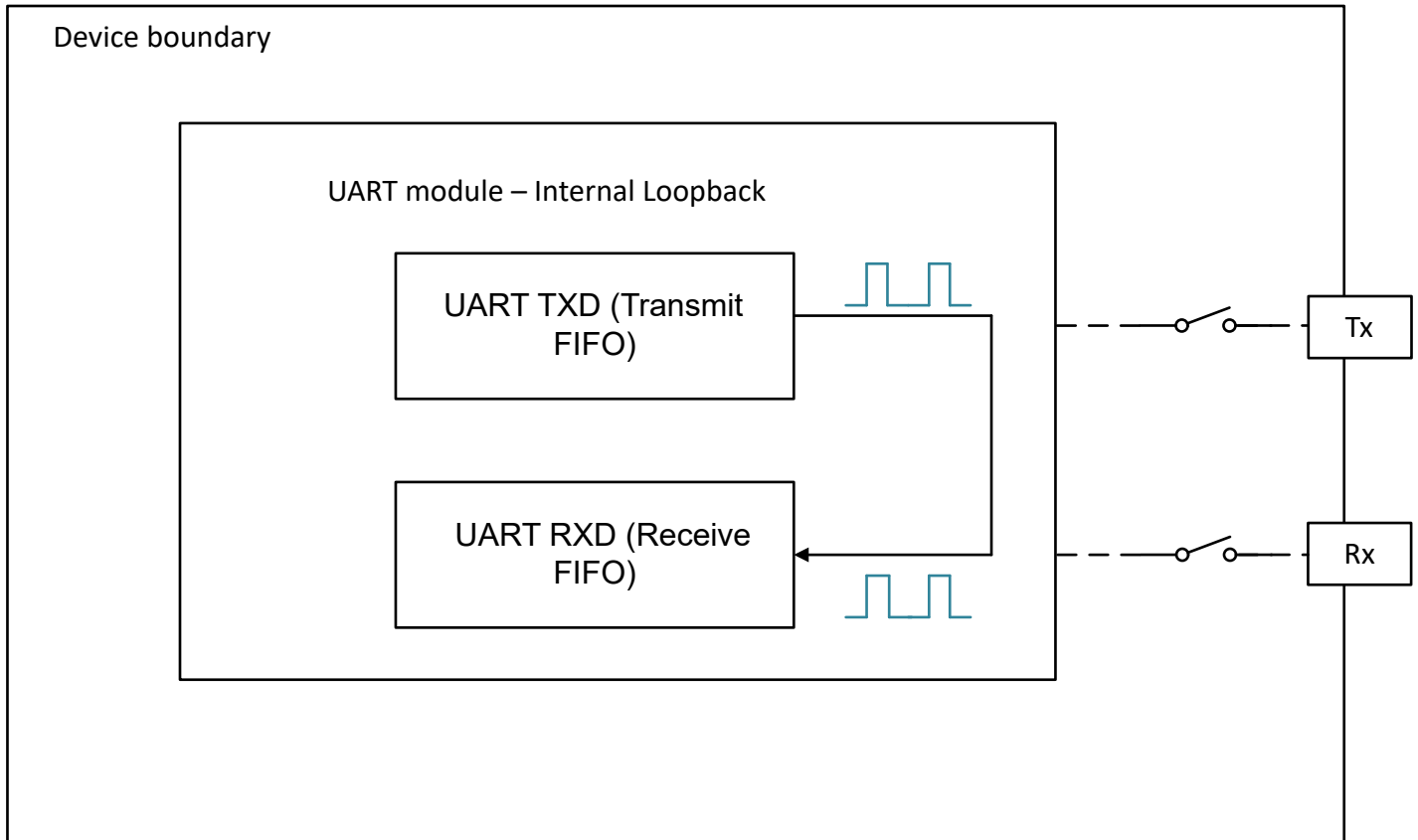
图 19-15. UART 环回模式
