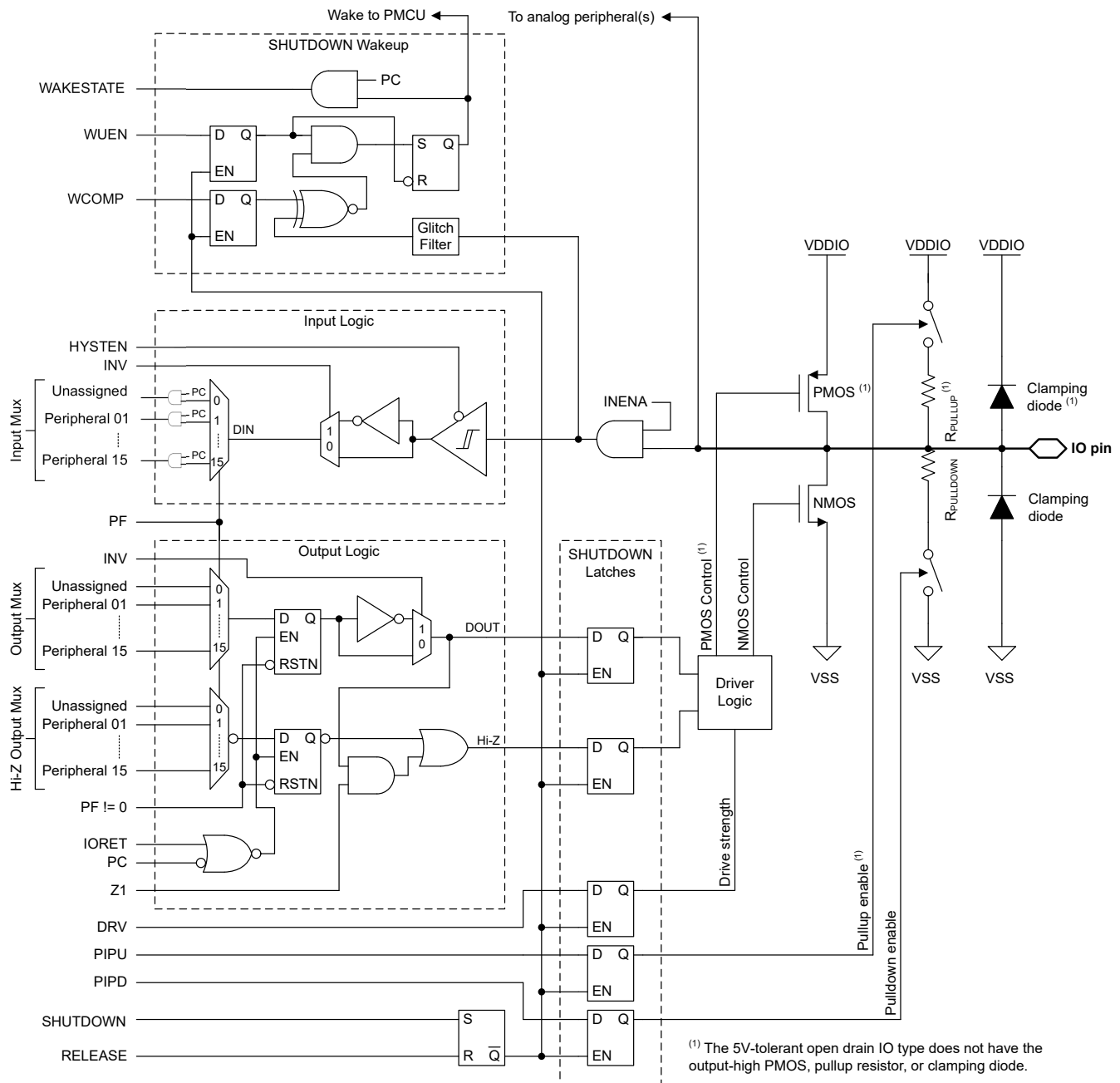
图 9-1. 超集 IO 切片
