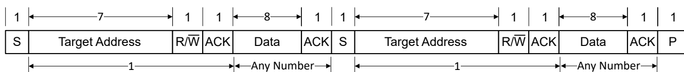
图 21-7. 重复启动条件下的数据格式
