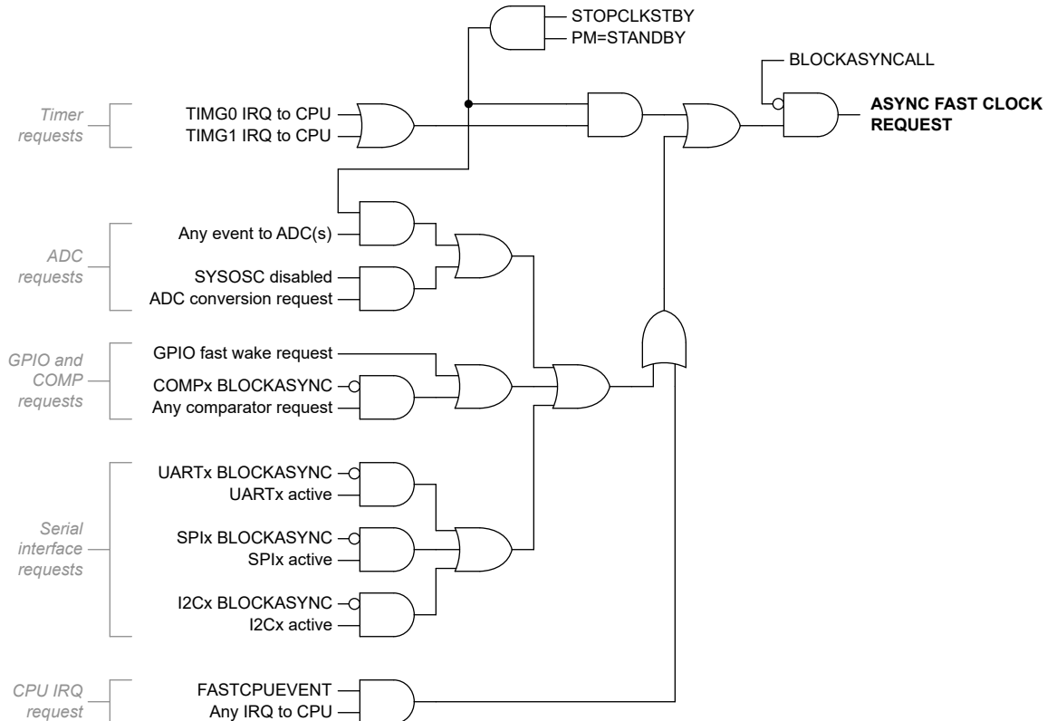
图 2-10. MSPM0Lxx 异步快速时钟请求逻辑
