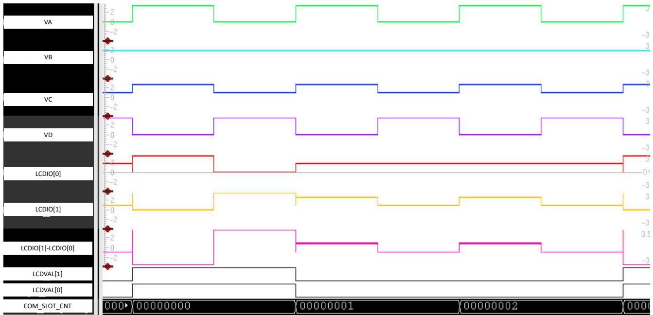
图 24-3. 1/3 偏置段相对于 COM0 开启
