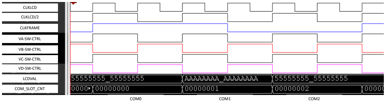
图 24-30. 存储器访问时序 - 低功耗模式
