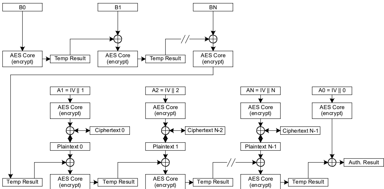
图 11-9. CCM 协议操作
