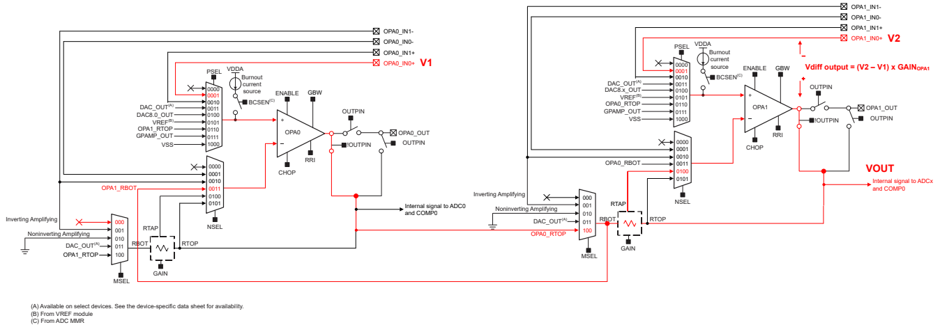
图 16-8. 差分放大器配置中的两个 OPA
