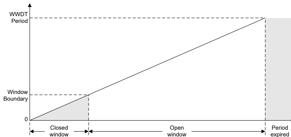
图 27-1. WWDT 功能
