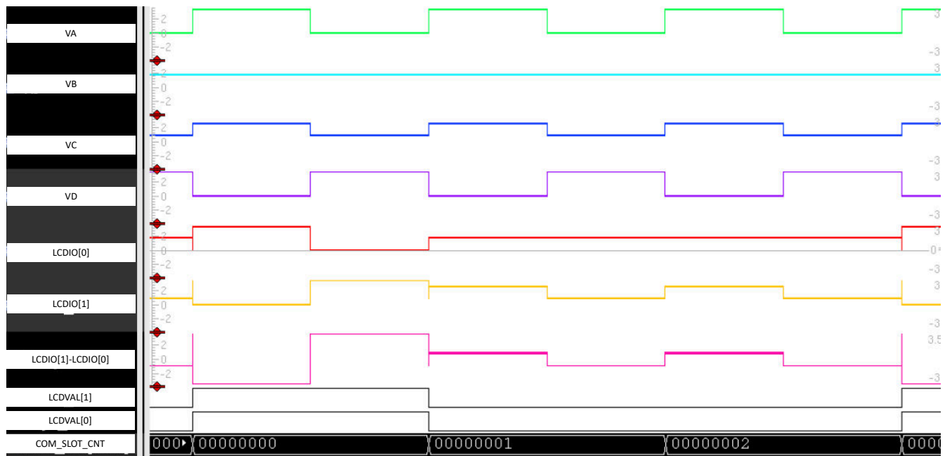
图 24-33. IO 多路复用波形
