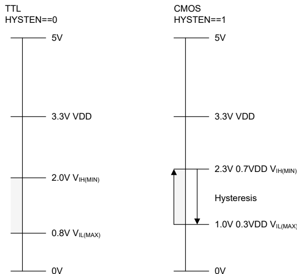
图 9-2. 输入逻辑电平 - 5V 容限开漏数字 IO
