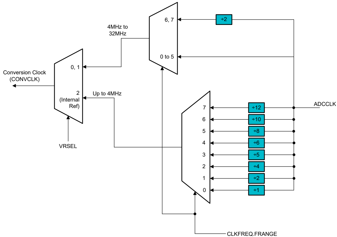
图 14-2. ADC 转换时钟生成逻辑
