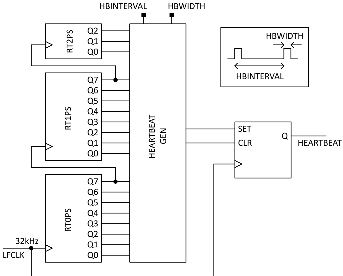
图 8-6. 检测信号发生器电路图
