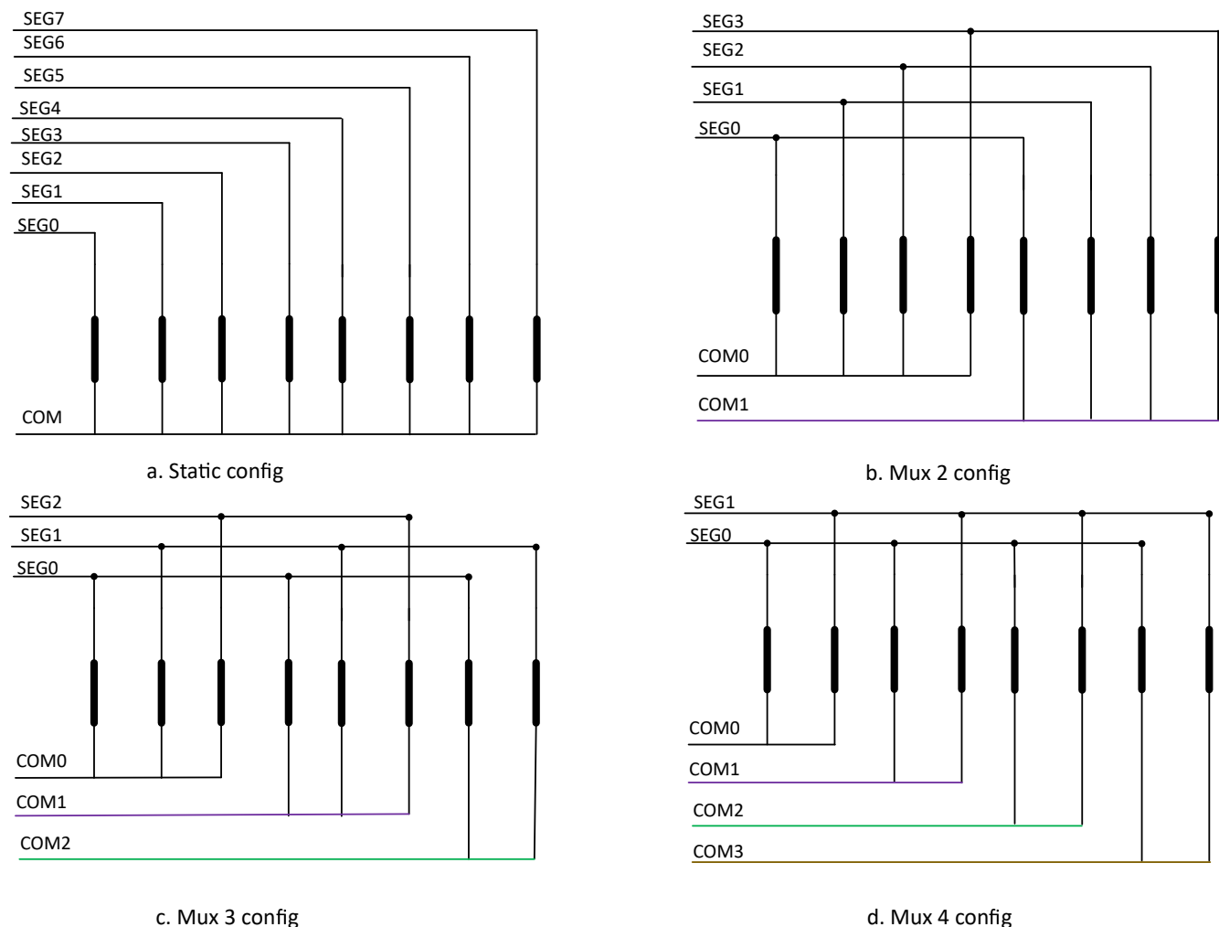
图 24-2. 多路复用配置
