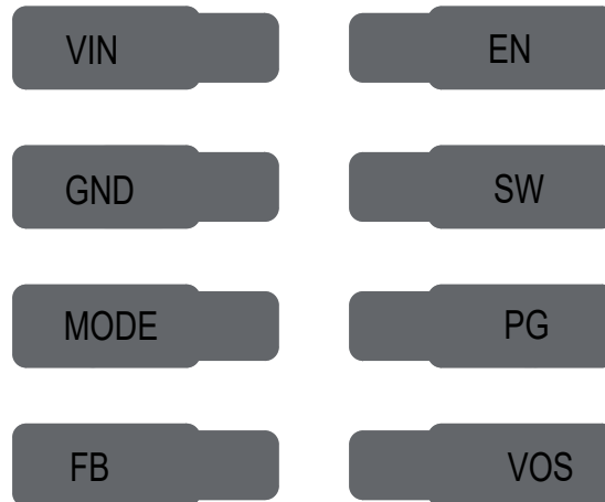
图 2-1. 重叠的 QFN 和 SOT583 封装
