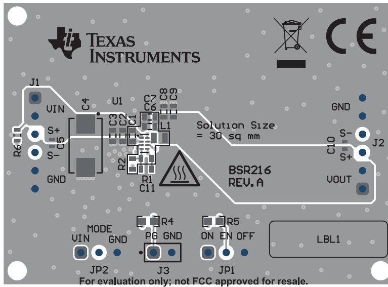
图 5-1. 顶层装配图
