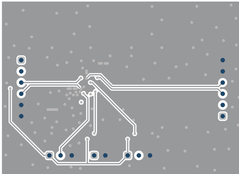
图 5-4. 信号层 2
