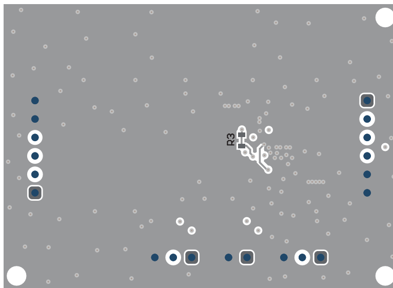
图 5-6. 底层装配图
