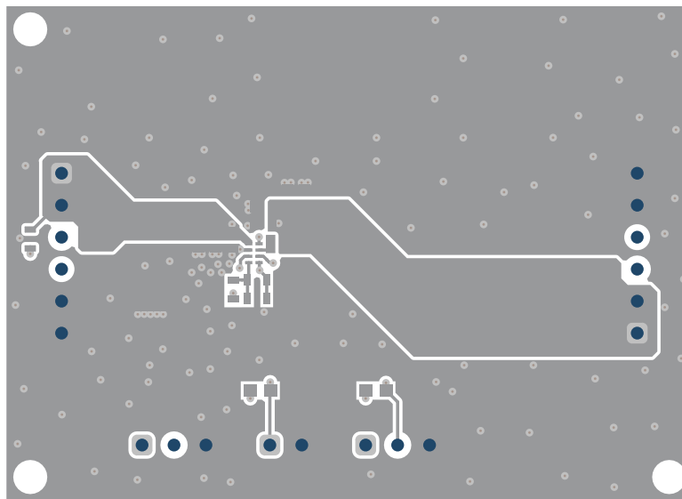
图 5-2. 顶层
