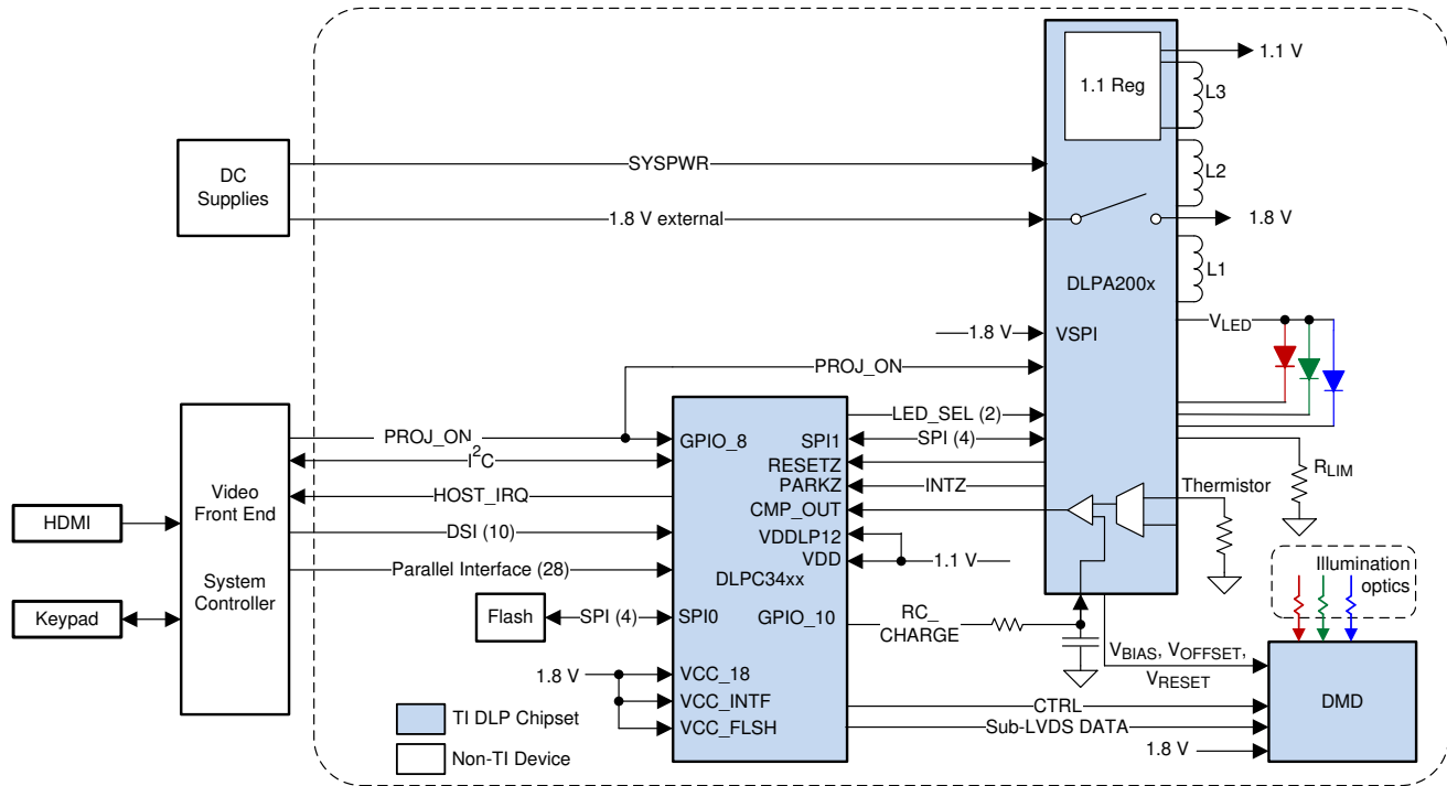
图 1-1. 典型简化应用原理图
