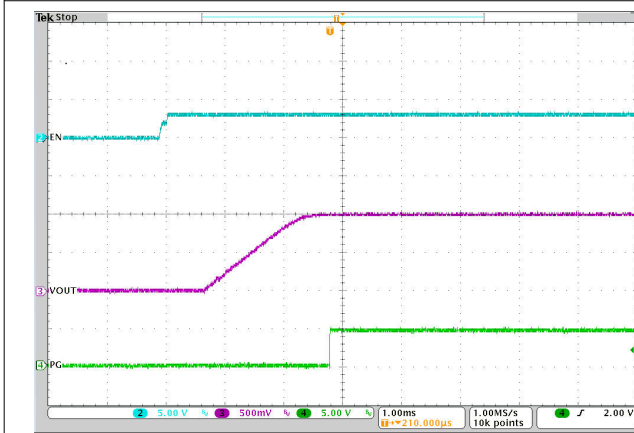
图 3-17. 通过 EN 启动 U1，8A
