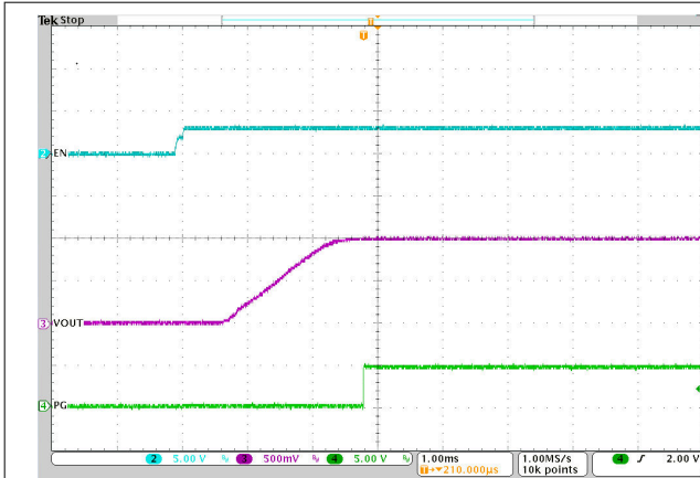
图 3-15. 通过 EN 启动 U1，空载
