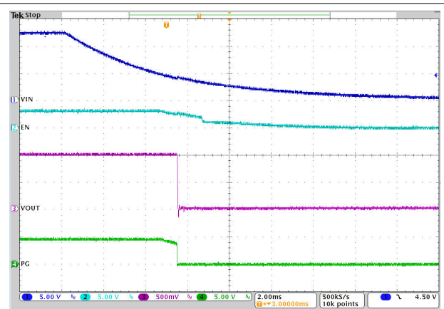
图 3-20. 通过 VIN 关断 U1，8A 负载
