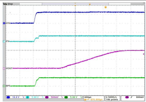
图 3-18. 通过 EN 启动 U1，空载并且测量 BP5
