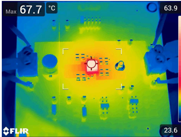
图 3-22. U1 热性能，12A 负载
