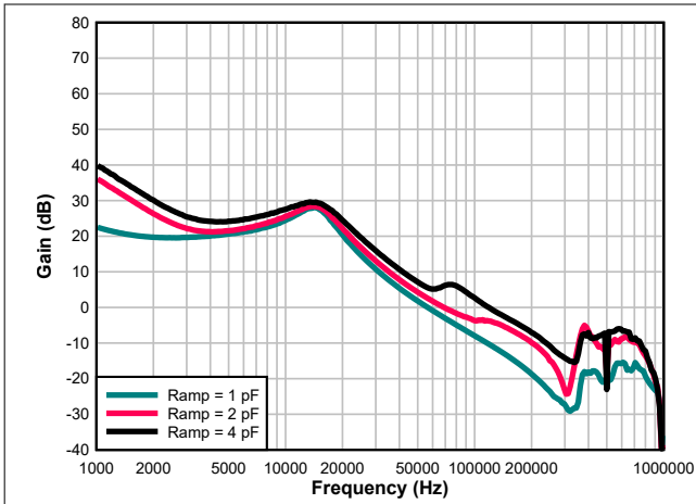
图 3-11. 具有不同斜坡设置的 U1 环路增益
