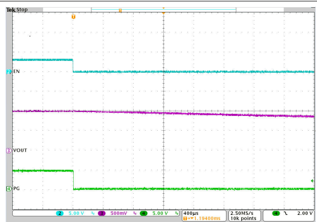
图 3-16. 通过 EN 关断 U1，空载
