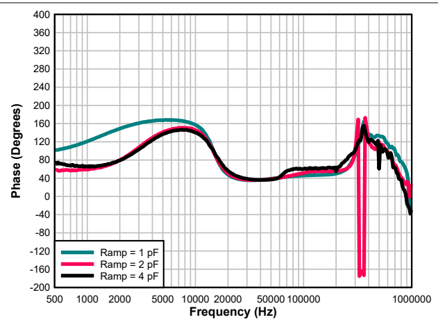
图 3-12. 具有不同斜坡设置的 U1 环路相位
