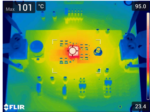
图 3-23. U1 热性能，16A 负载
