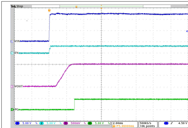
图 3-19. 通过 VIN 启动 U1，空载
