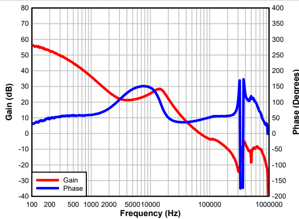
图 3-10. U1 波特图 - 16A 负载
