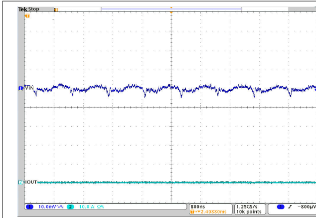
图 3-13. U1 输入纹波，空载
