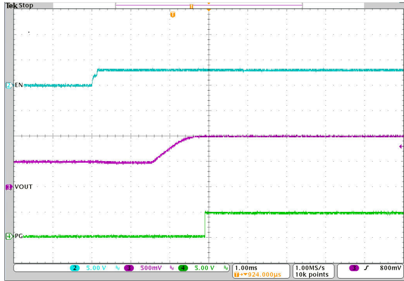
图 3-21. U1 启动至 0.5V 预偏置
