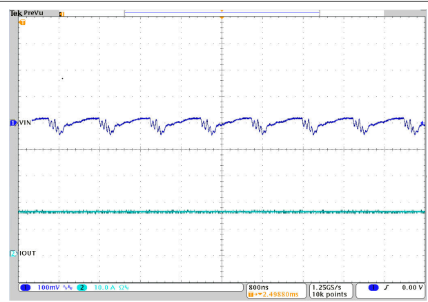
图 3-14. U1 输入纹波，16A 负载
