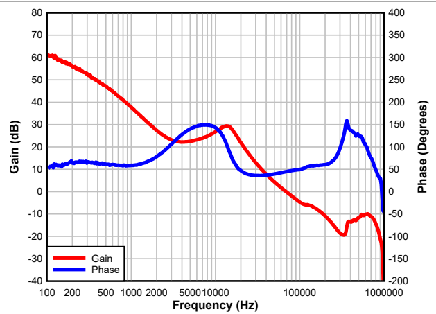
图 3-9. U1 波特图 - 12A 负载
