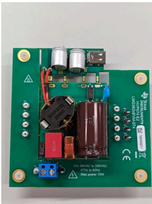
LMG3624EVM-081 (顶视图)
