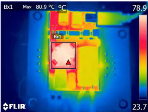
图 3-40. V_{IN} = 230V_{AC} , 顶面
