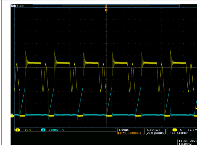
图 3-11. Vin = 230Vac , Vout = 20V
