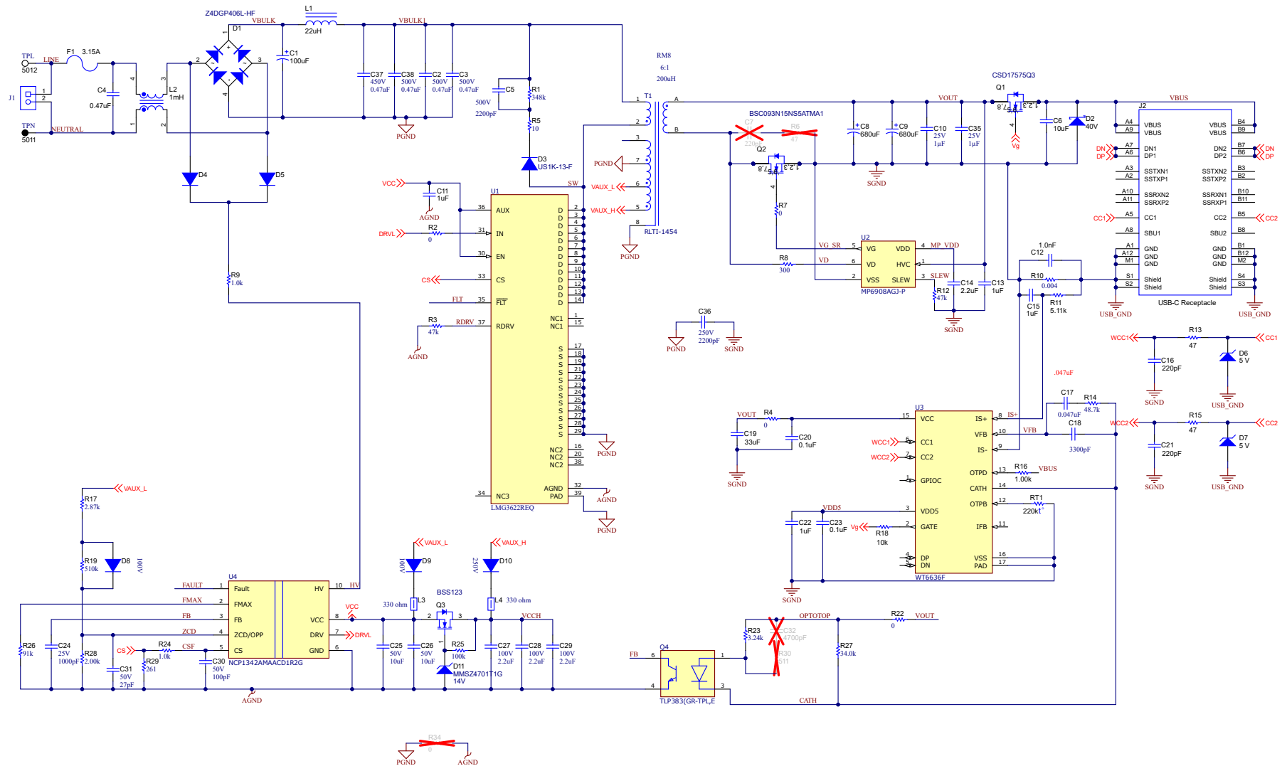
图 4-1. LMG3624EVM-081 原理图
