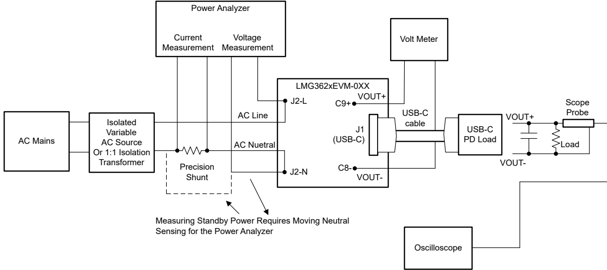
图 3-1. LMG3624EVM-081 测试设置图
