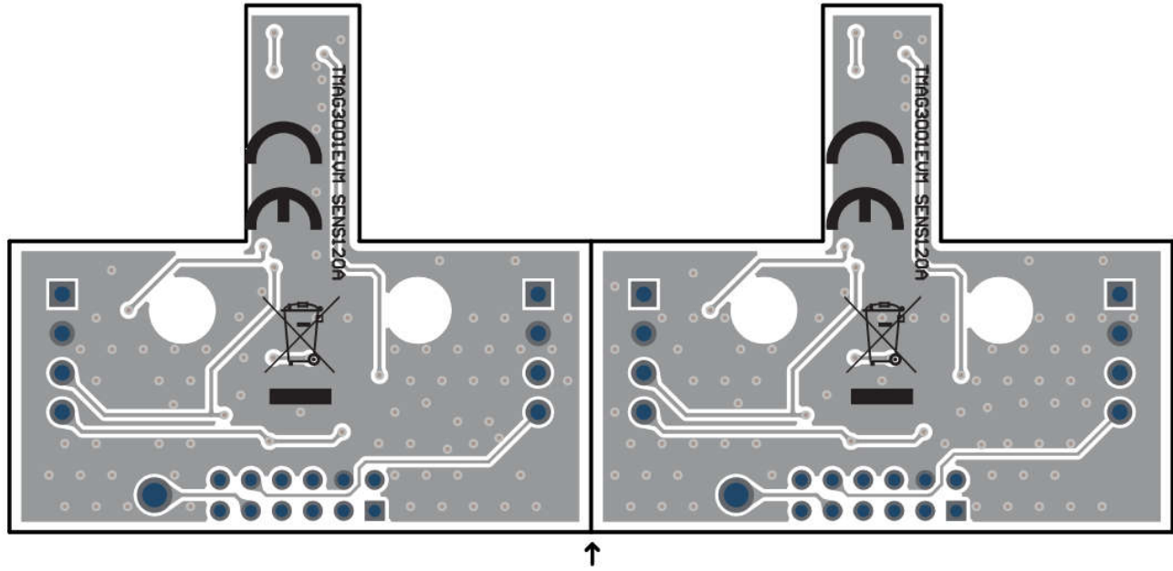
图 4-6. TMAG3001EVM 底视图
