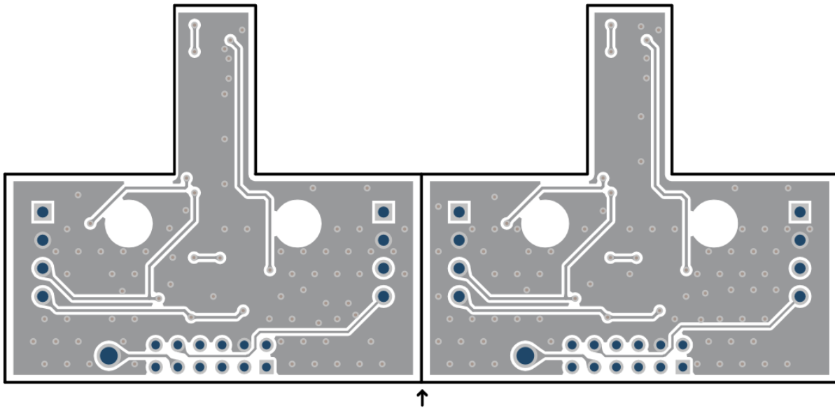
图 4-7. TMAG3001EVM 底层
