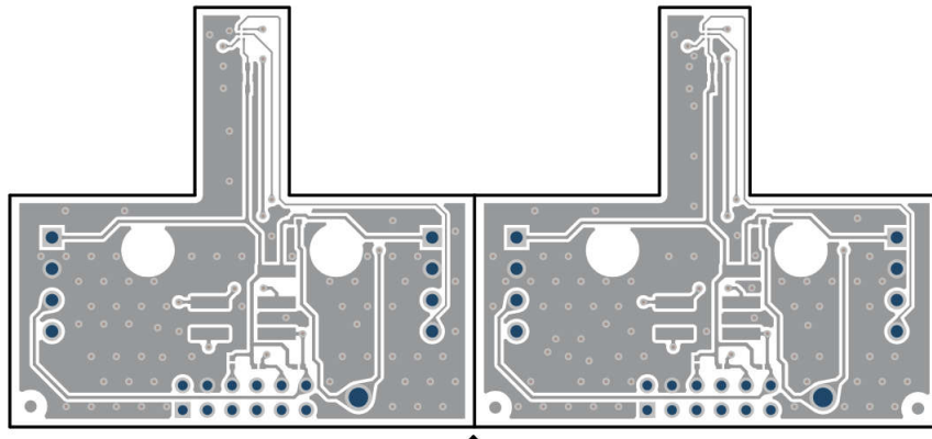
图 4-5. TMAG3001EVM 顶层
