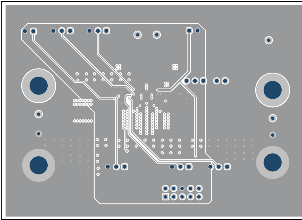
图 4-4. TPS55289Q1EVM-011 内层 2
