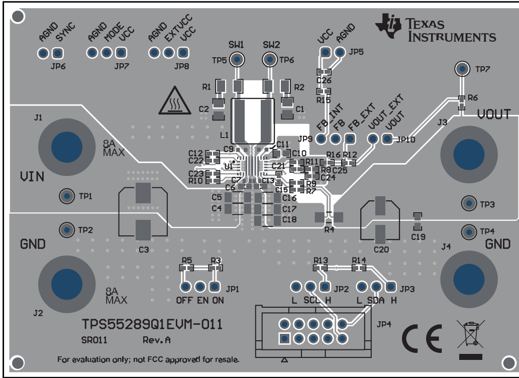
图 4-2. TPS55289Q1EVM-011 顶面布局
