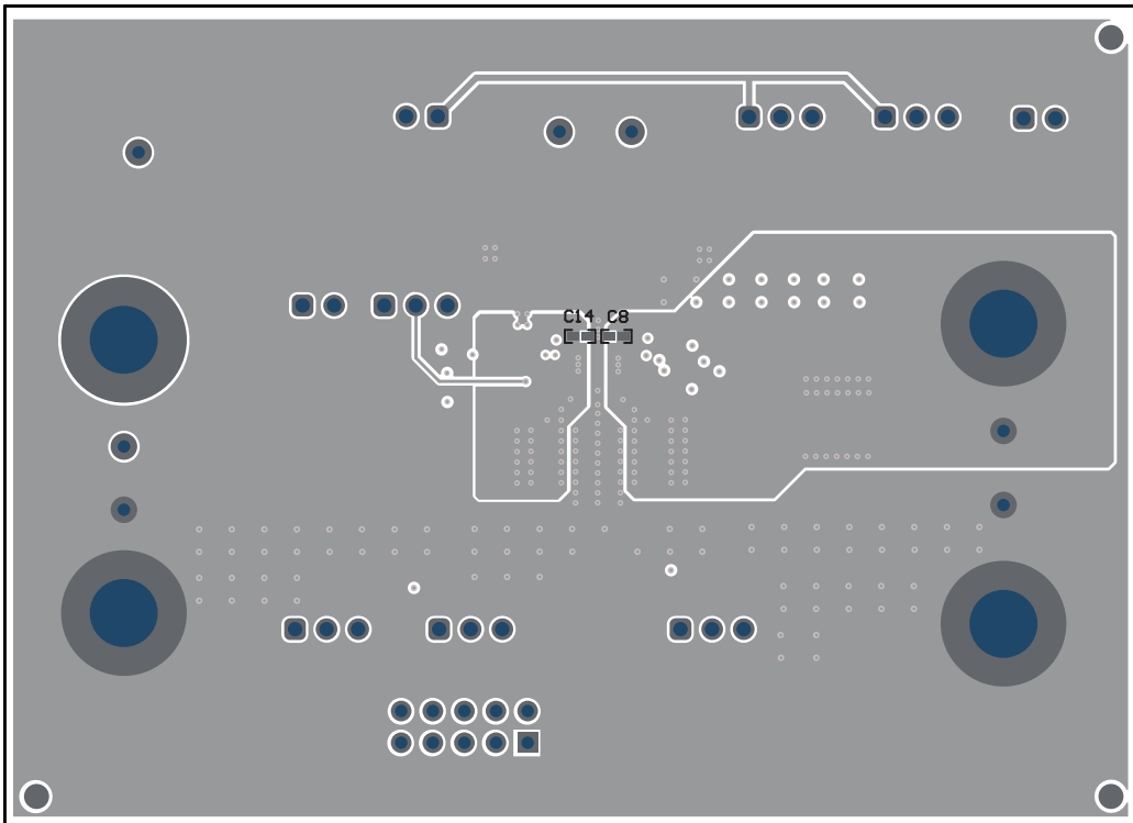
图 4-5. TPS55289Q1EVM-011 底面布局
