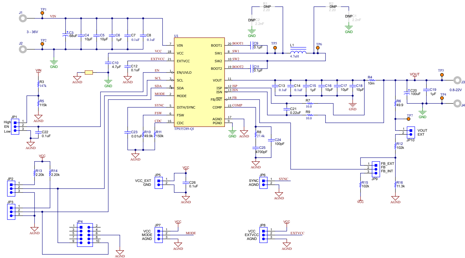
图 4-1. TPS55289Q1EVM-011 原理图
