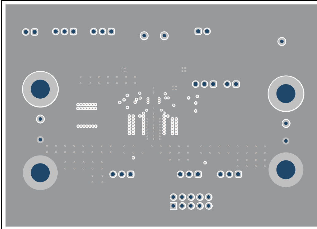
图 4-3. TPS55289Q1EVM-011 内层 1
