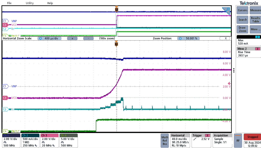
图 3-10. UCC33420-Q1 浪涌电流，序列 VINP=5.0V → EN=5.0V，VCC=5.0V，Iout=0mA
