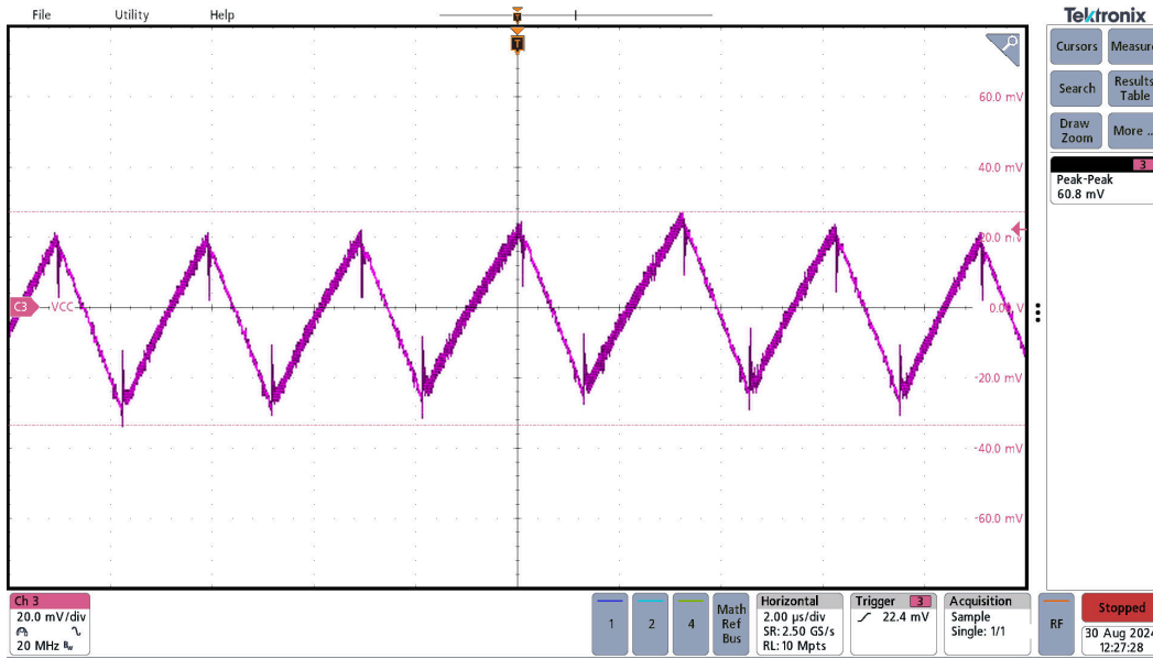
图 3-16. UCC33420-Q1 VCC 交流纹波，VINP=5.0V，VCC=5.0V，IOUT=300mA
