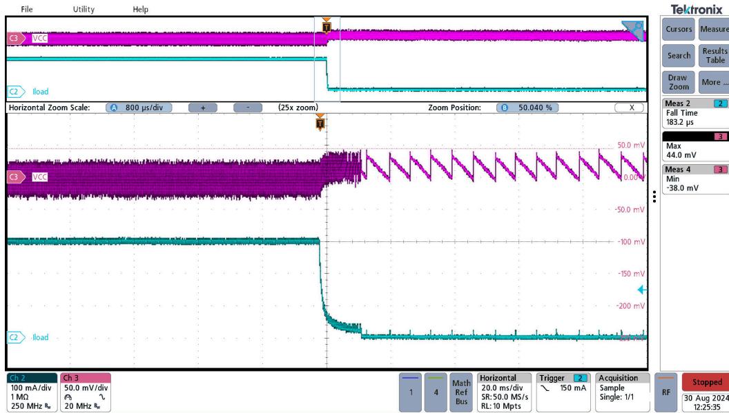
图 3-20. UCC33420-Q1 负载瞬态，VINP=5.0V，VCC=5.0V，满载 (Iout=300mA) 到空载 (Iout=0mA)
