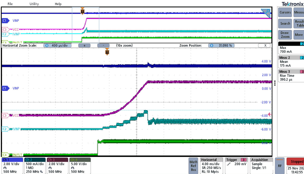
图 3-13. UCC33020-Q1 浪涌电流，序列 VINP=3.3V → EN=5.0V，VCC=5.0V，Rload=50 \Omega
