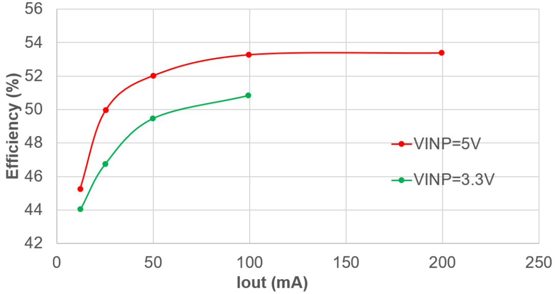
图 3-3. UCC33020-Q1 在 VCC = 5.0V 时的效率
