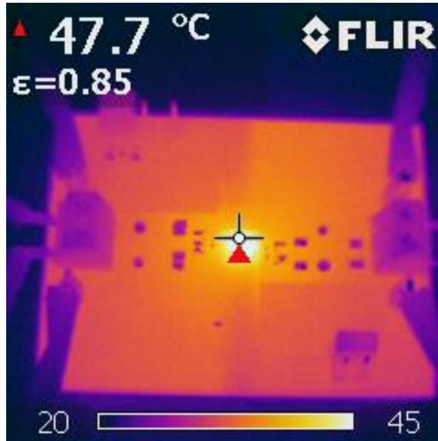
图 3-26. UCC33420-Q1 VINP=5.0V , VCC=5.0V , Iout=150mA , Pout=0.75W , TA=25°C
