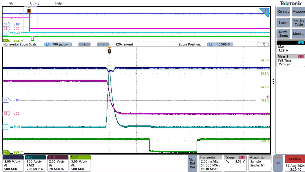
图 3-22. UCC33420-Q1 短路, VINP=5.0V, VCC=5.0V
