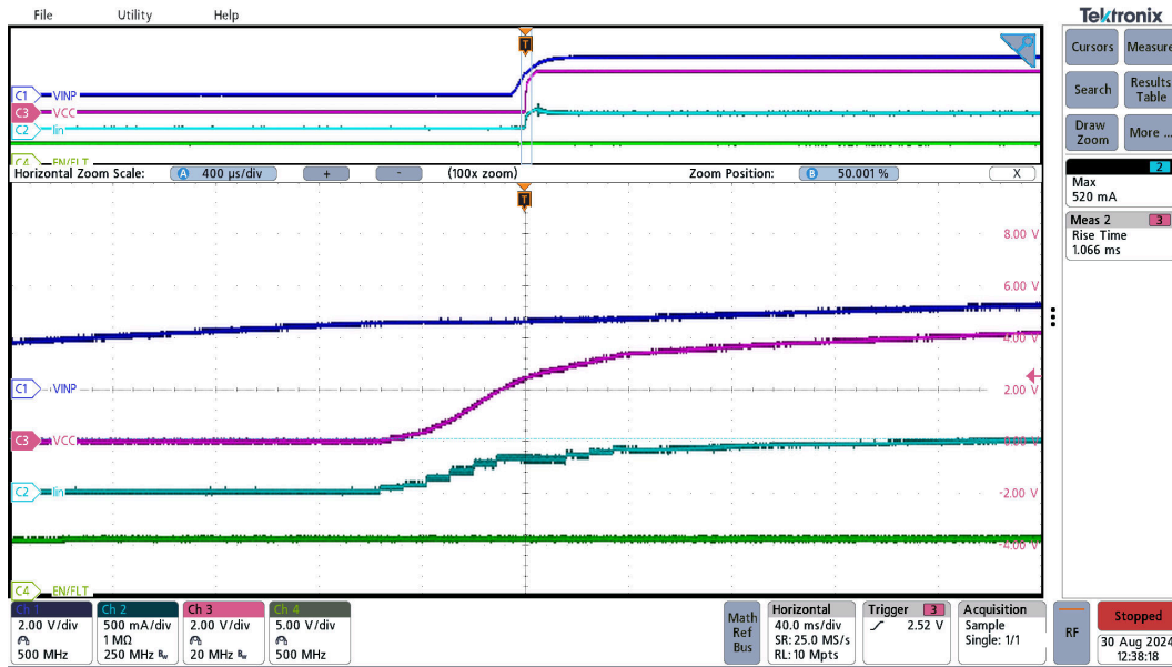
图 3-8. UCC33420-Q1 启动，序列 EN=5.0V → VINP=5.0V，VCC=5.0V，Rload=18 Ω
