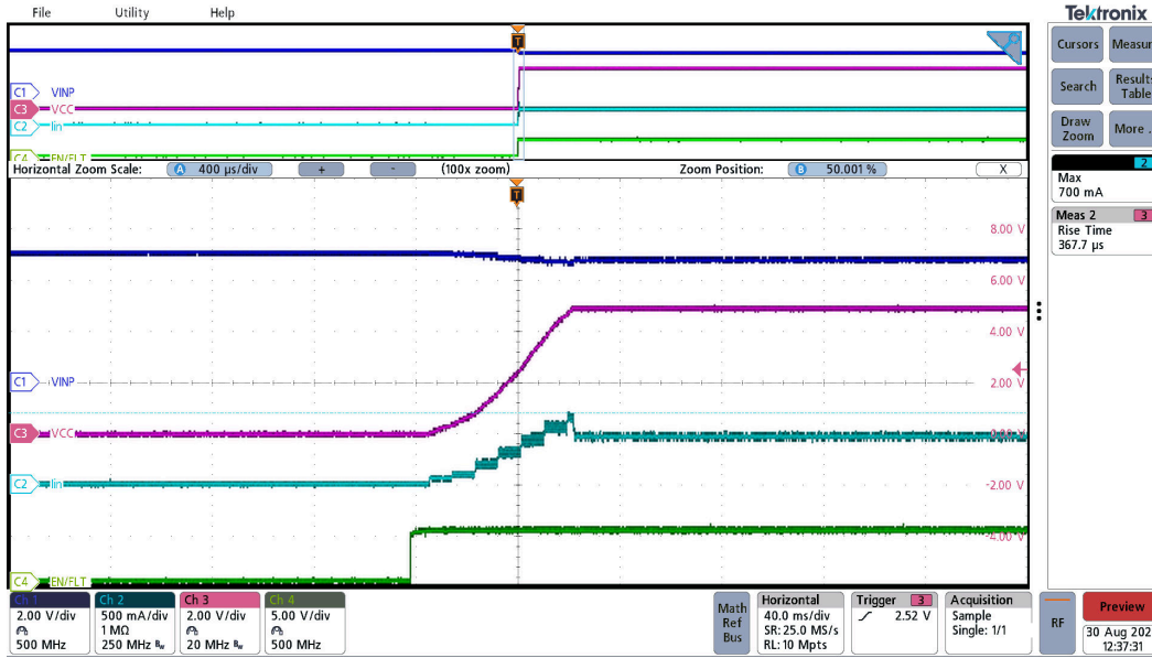
图 3-12. UCC33420-Q1 浪涌电流，序列 VINP=5.0V → EN =5.0V，VCC=5.0V，Rload=18 \Omega
