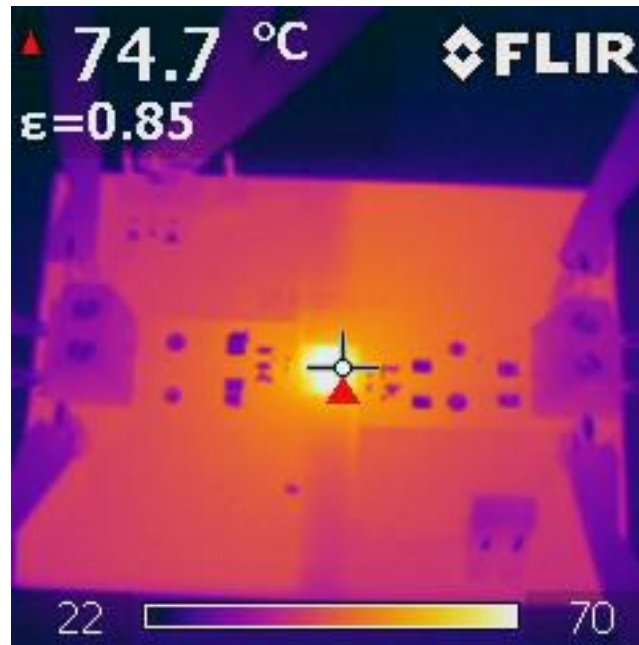
图 3-24. UCC33420-Q1 VINP=5.0V , VCC=5.0V , Iout=300mA , Pout=1.5W , TA=25°C
