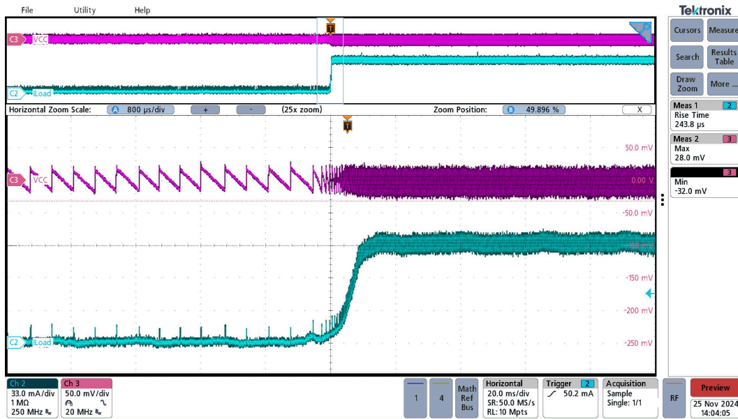
图 3-19. UCC33020-Q1 负载瞬态，VINP=3.3V，VCC=5.0V，空载 (Iout=0mA) 到满载 (Iout=100mA)
