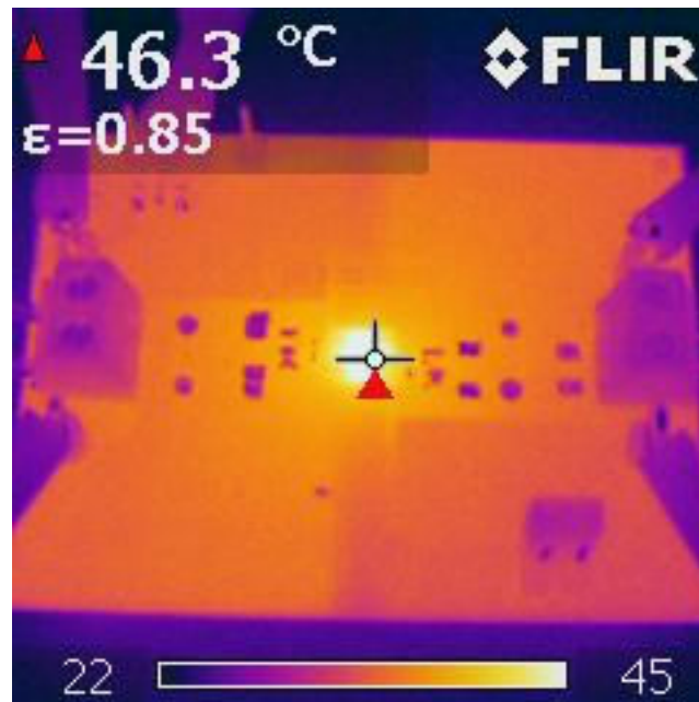
图 3-25. UCC33020-Q1 VINP=3.3V , VCC=5.0V , Iout=100mA , Pout=0.5W , TA=25°C
