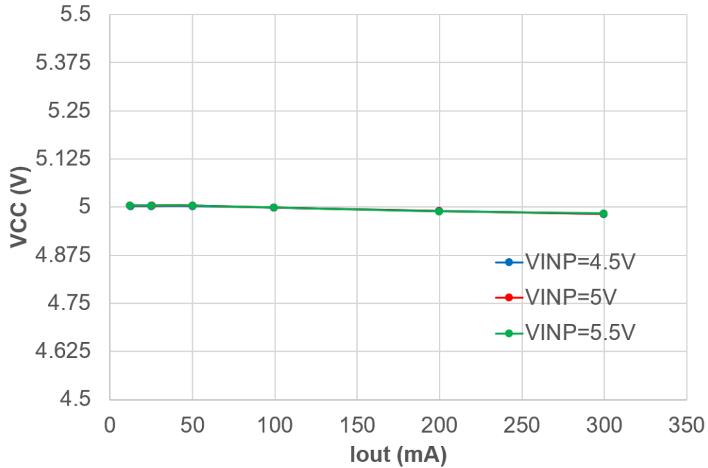
图 3-4. UCC33420-Q1 调节与负载电流间的关系 VCC = 5.0V
