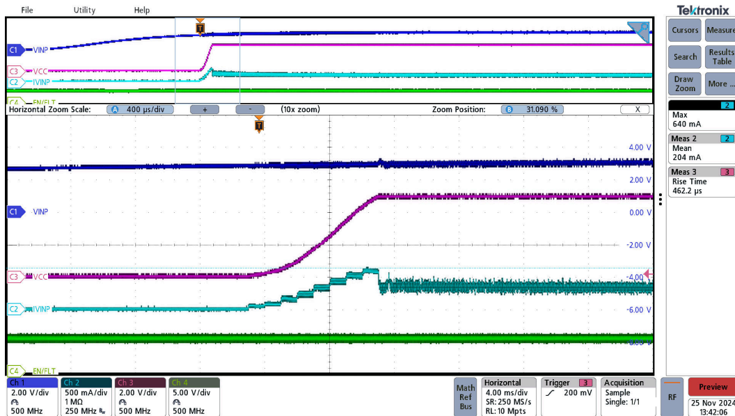
图 3-9. UCC33020-Q1 启动，序列 EN=5.0V → VINP=3.3V，VCC=5.0V，Rload=50 Ω
