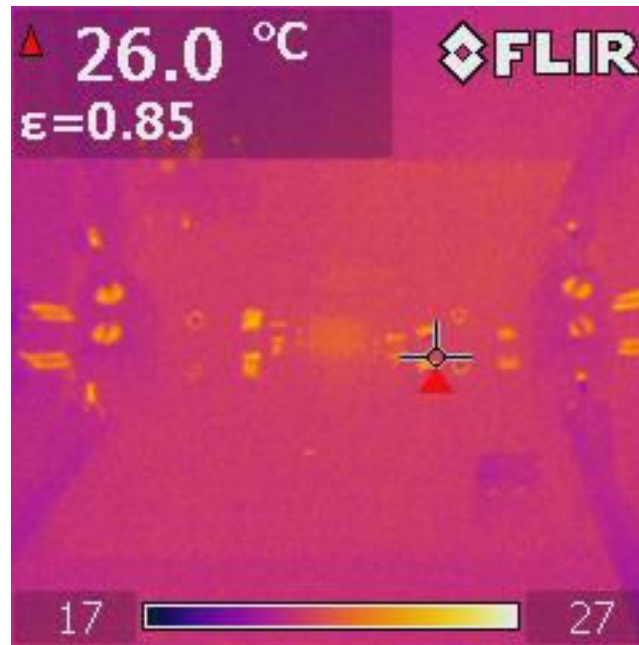
图 3-28. UCC33420-Q1 VINP=5.0V , VCC=5.0V , Iout=0mA , Pout=0W , TA=25°C
