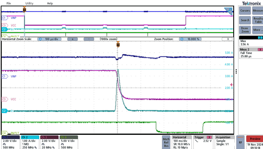
图 3-23. UCC33020-Q1 短路, VINP=3.3V, VCC=5.0V
