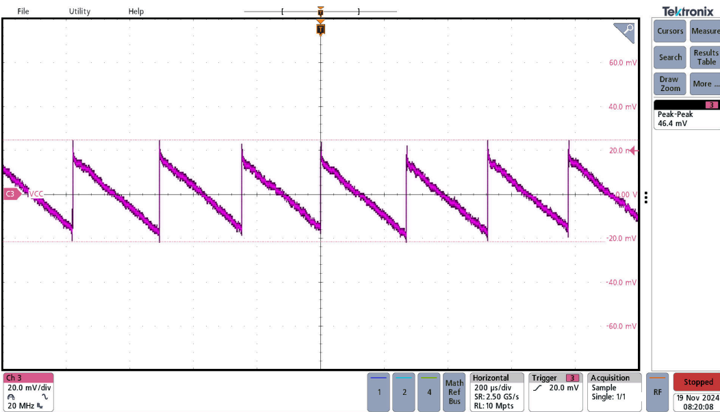
图 3-15. UCC33020-Q1 VCC 交流纹波，VINP=3.3V，VCC=5.0V，IOUT=0mA
