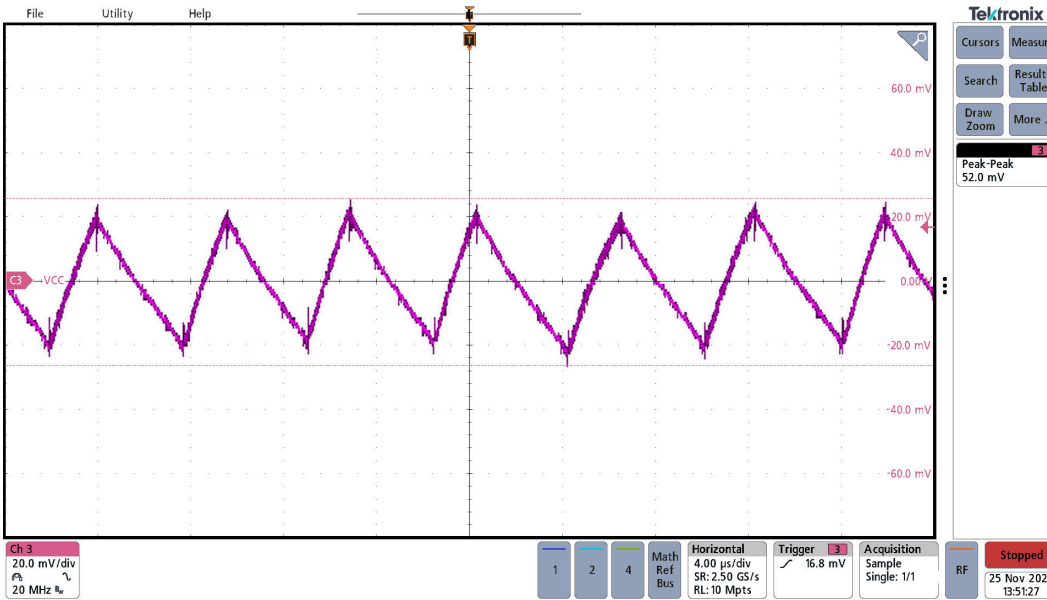
图 3-17. UCC33020-Q1 VCC 交流纹波，VINP=3.3V，VCC=5.0V，IOUT=100mA
