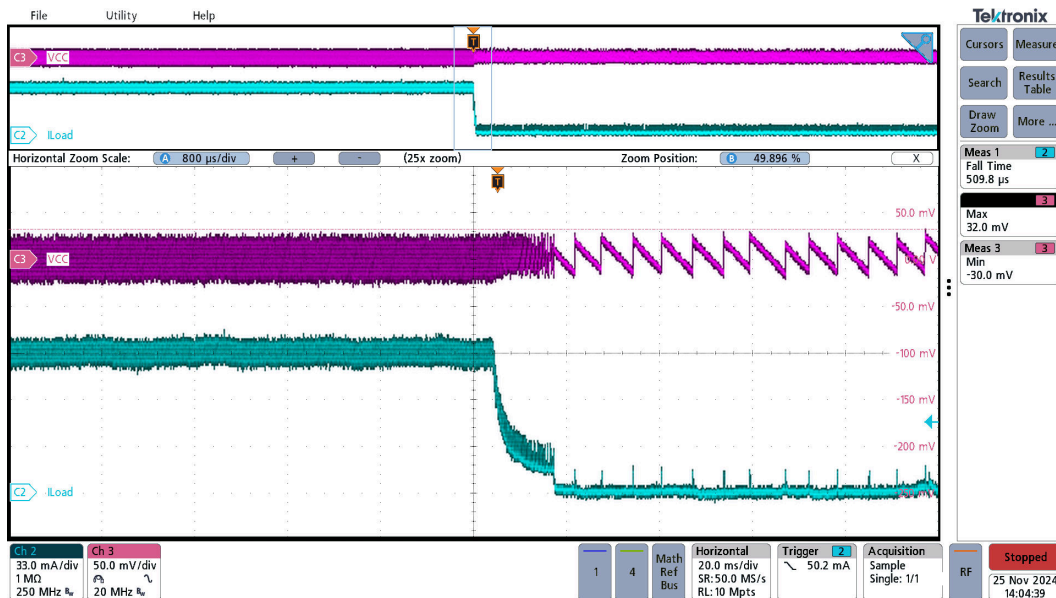
图 3-21. UCC33020-Q1 负载瞬态，VINP=3.3V，VCC=5.0V，满载 (Iout=100mA) 到空载 (Iout=0mA)
