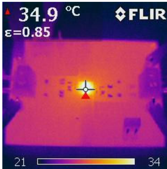
图 3-27. UCC33020-Q1 VINP=3.3V , VCC=5.0V , Iout=50mA , Pout=0.25W , TA=25°C
