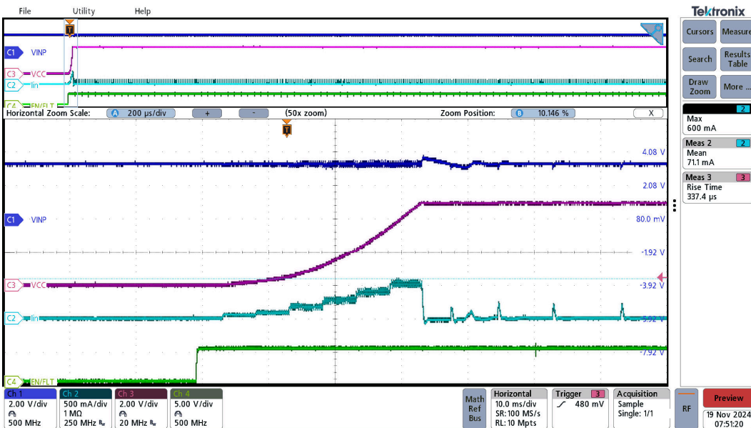
图 3-11. UCC33020-Q1 浪涌电流，序列 VINP=3.3V → EN=5.0V，VCC=5.0V，Iout=0mA
