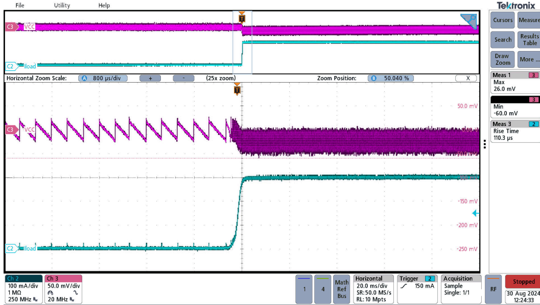
图 3-18. UCC33420-Q1 负载瞬态，VINP=5.0V，VCC=5.0V，空载 (Iout=0mA) 到满载 (Iout=300mA)
