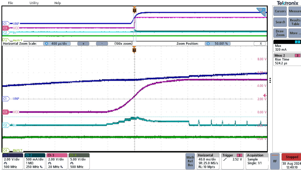
图 3-6. UCC33420-Q1 启动，序列 EN=5.0V → VINP=5.0V，VCC=5.0V，Iout=0mA
