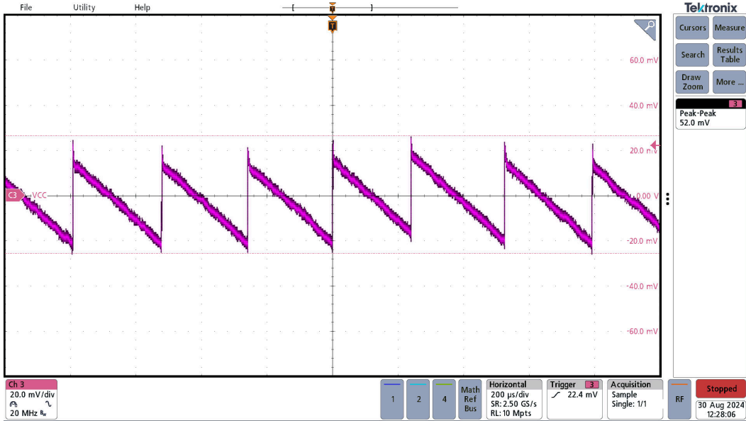
图 3-14. UCC33420-Q1 VCC 交流纹波，VINP=5.0V，VCC=5.0V，IOUT=0mA
