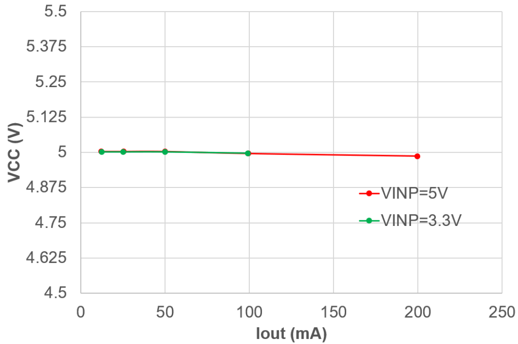
图 3-5. UCC33020-Q1 调节与负载电流间的关系 VCC = 5.0V
