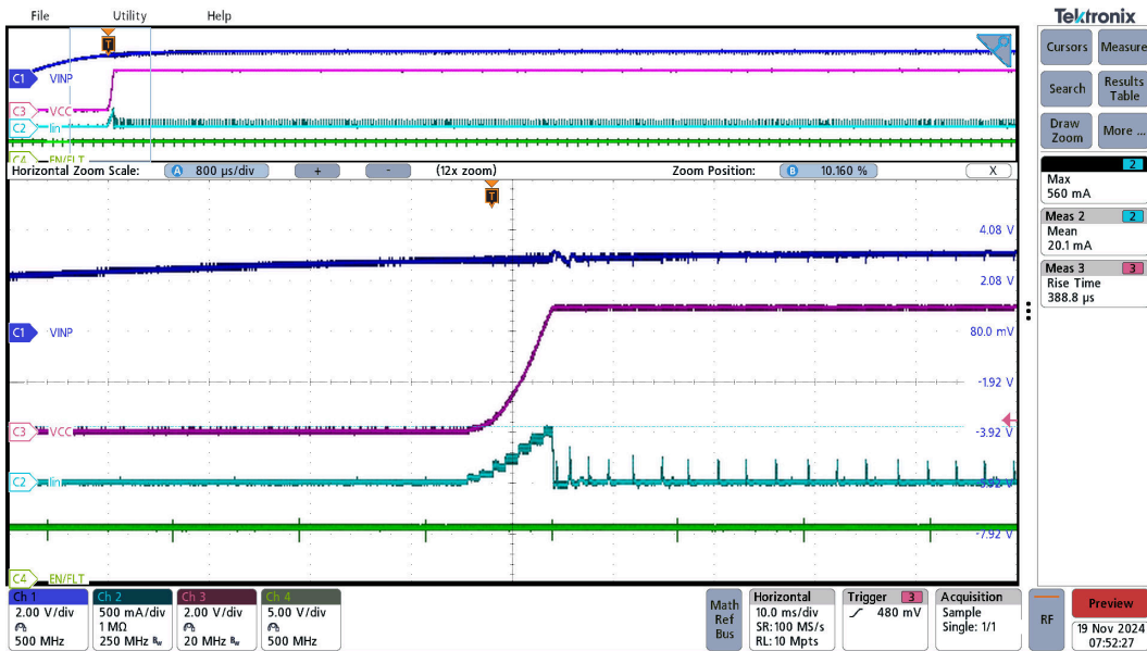
图 3-7. UCC33020-Q1 启动，序列 EN=5.0V → VINP=3.3V，VCC=5.0V，Iout=0mA
