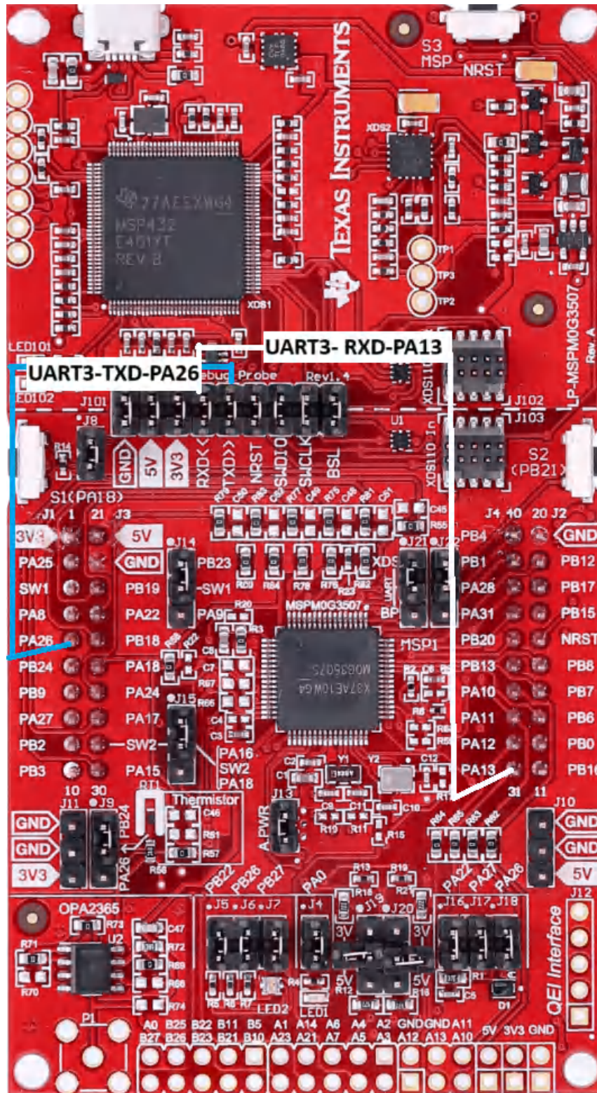
图 2-5. LP-MSPM0G3507 反向通道连接到 UART3
