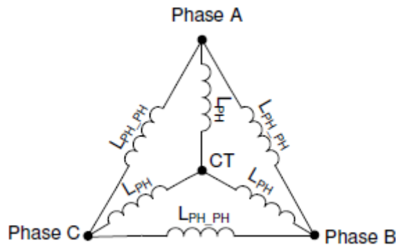
图 6-3. 电感测量
