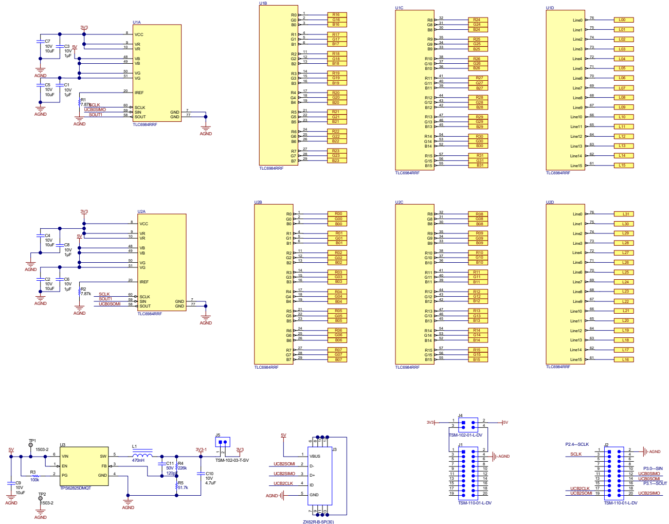
图 5-1. TLC6984EVM 原理图 (第 1 个, 共 3 个)
