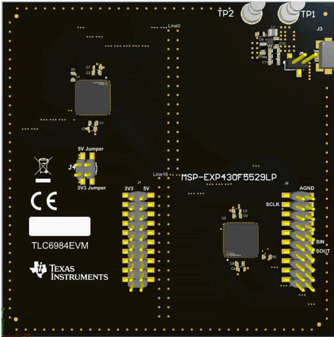
图 2-1. TLC6984EVM 电路板的驱动器 IC 侧
