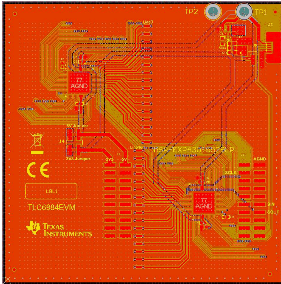
图 5-4. TLC6984EVM 布局
