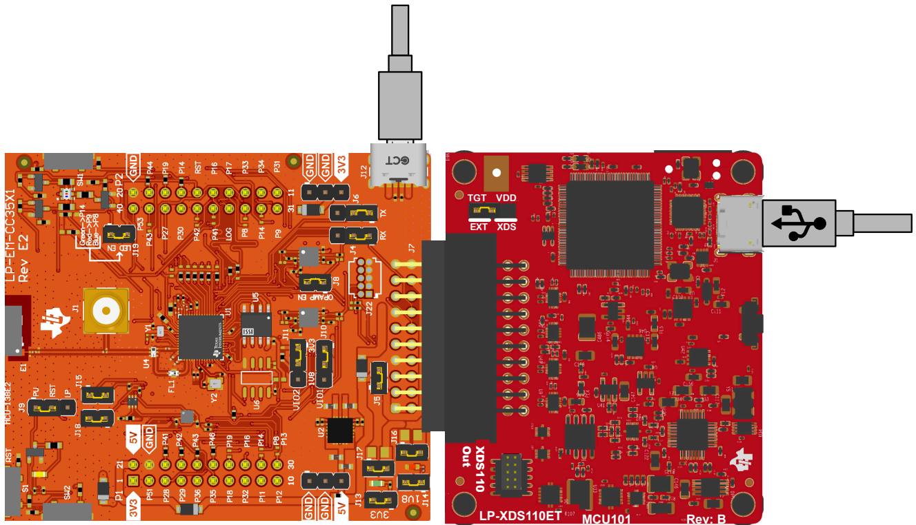
图 2-27. LP-EM-CC35X1 连接到 LP-XDS110 (ET)
