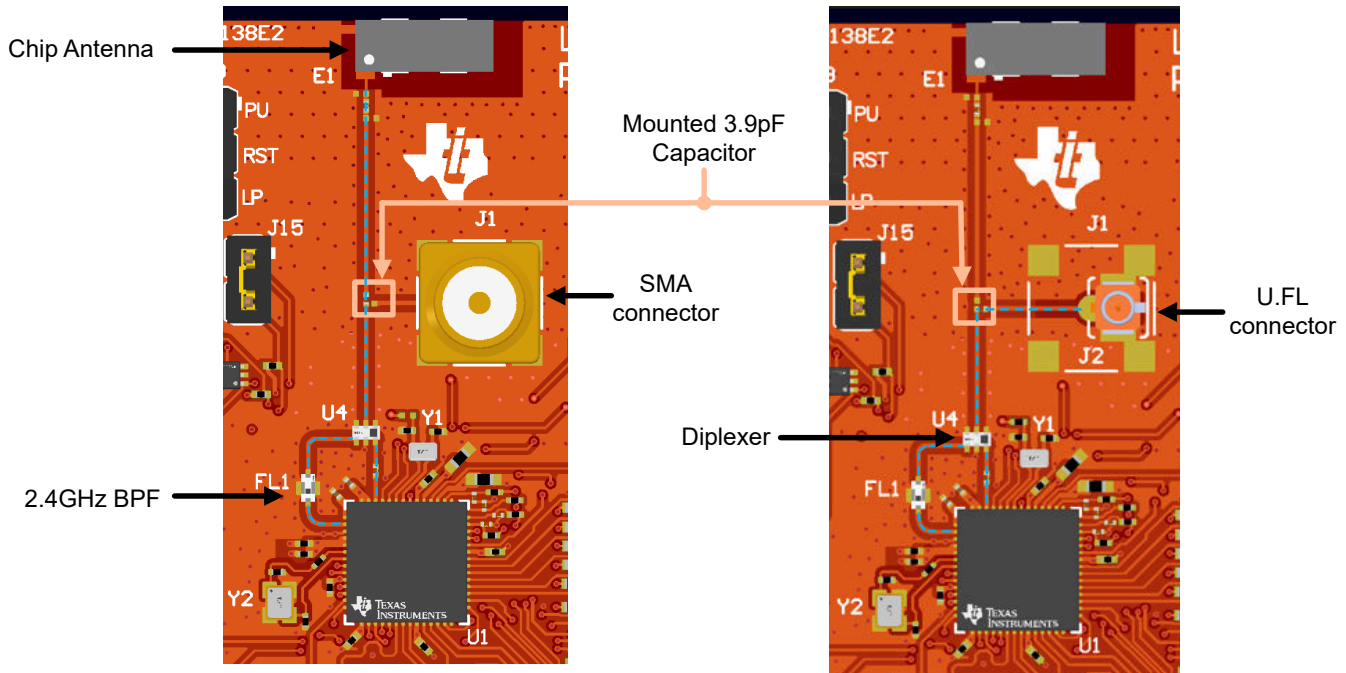
图 2-26. LP-EM-CC35X1 上的射频路径
