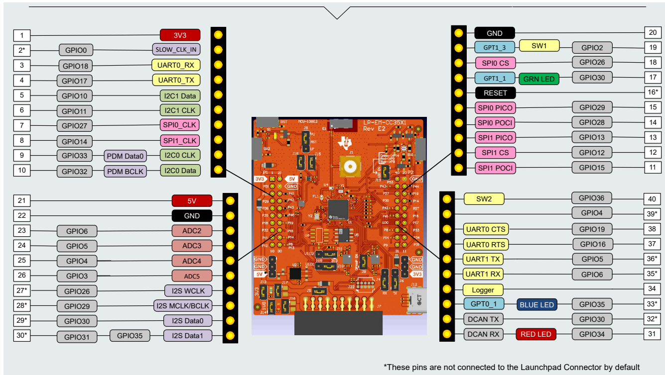
图 2-19. CC35xxE LaunchPad 接头引脚分配
