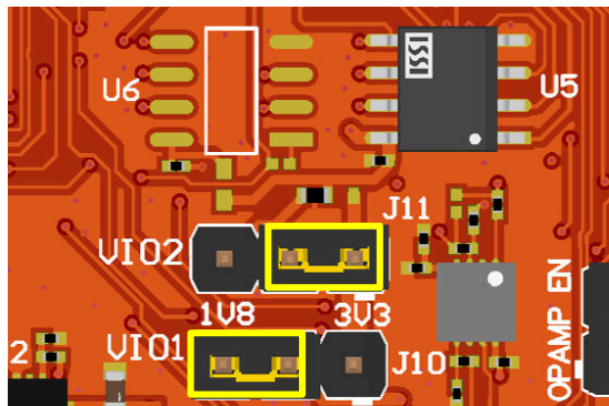
图 2-21. VIO 选择示例
