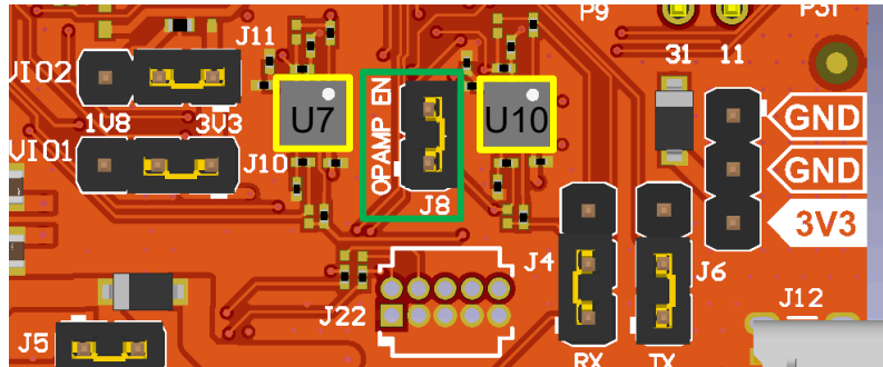
图 2-12. ADC 缓冲器
