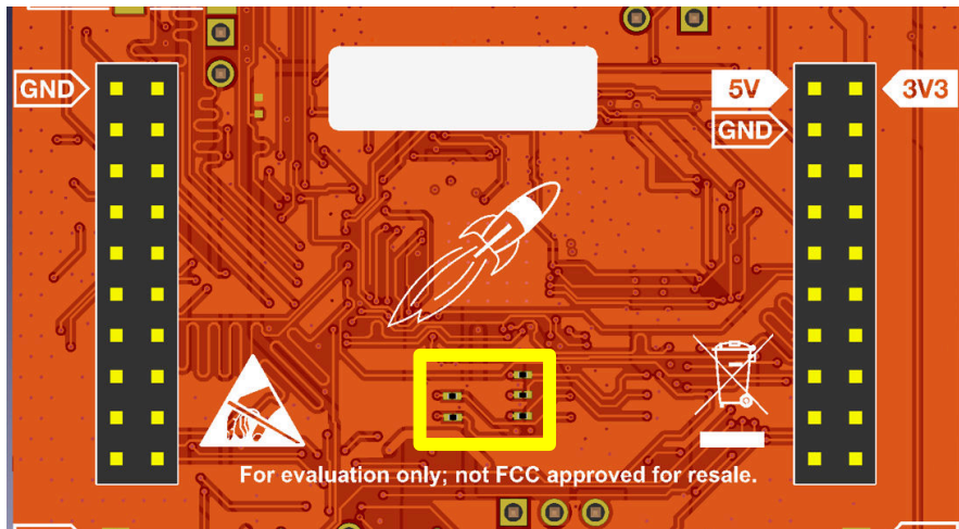
图 2-11. 外部 PSRAM 板 (底视图)
