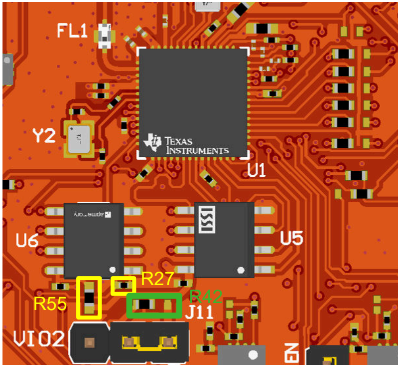
图 2-10. 外部 PSRAM 板 (顶视图)
