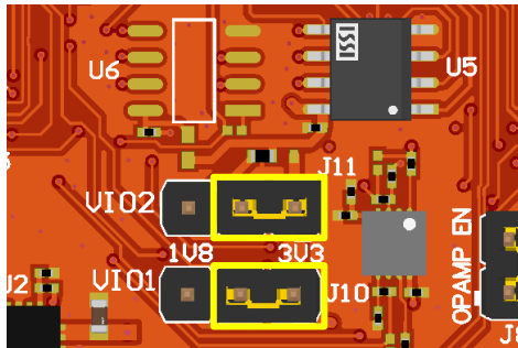
图 2-20. VIO 跳线
