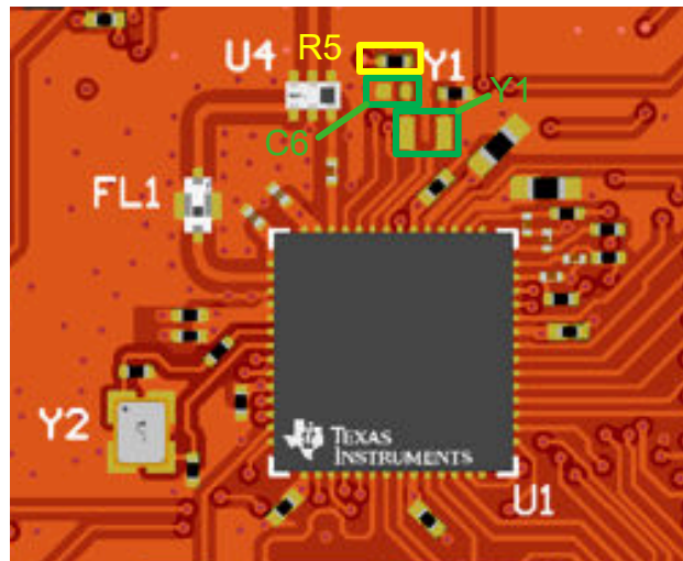
图 2-25. 外部慢速时钟
