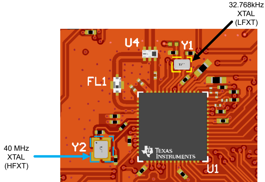
图 2-24. 时钟
