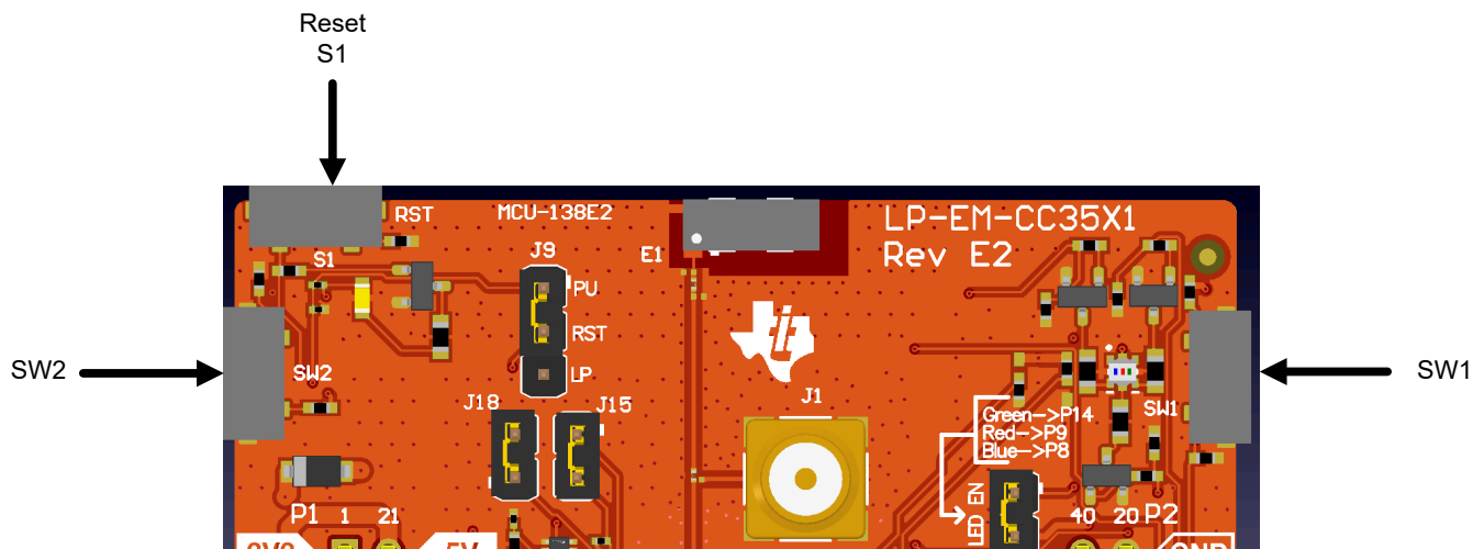
图 2-16. 按钮
