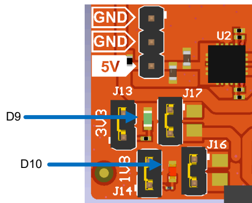
图 2-18. 电源 LED
