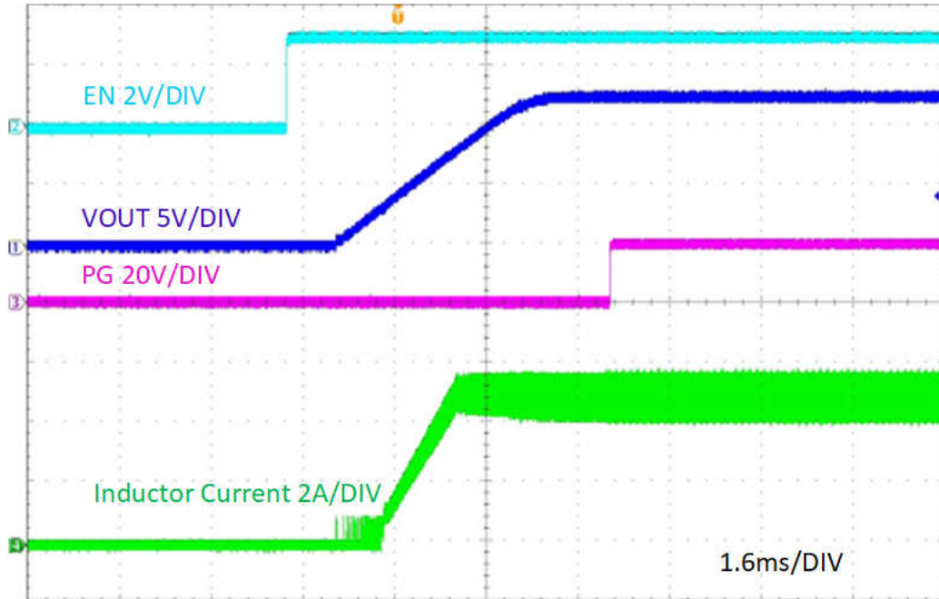
图 3-2. 相对于 EN 的启动, V_{IN} = 24V , I_{OUT} = 5A
