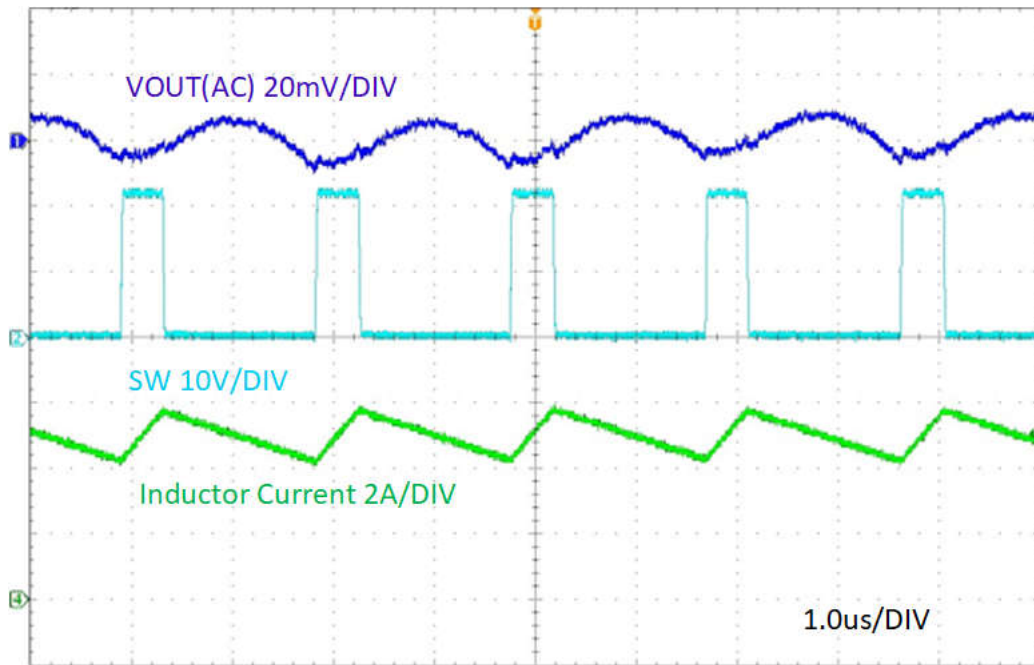
图 3-7. TPS54538EVM 输出电压纹波, I_{OUT} = 5A
