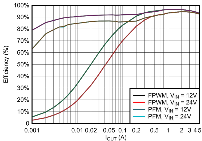
图 3-1. 效率，ECO 模式， V_{OUT} = 5.0V ，500kHz
