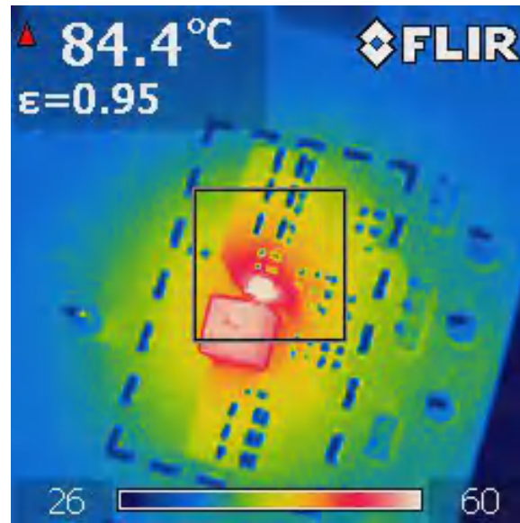
图 3-8. 热性能， V_{IN} = 24V ， I_{OUT} = 5A ， T_{amb} = 25^{\circ}C ，无气流
