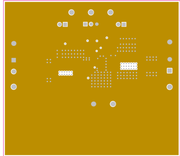
图 4-3. 第 2 层覆铜 (顶视图)
