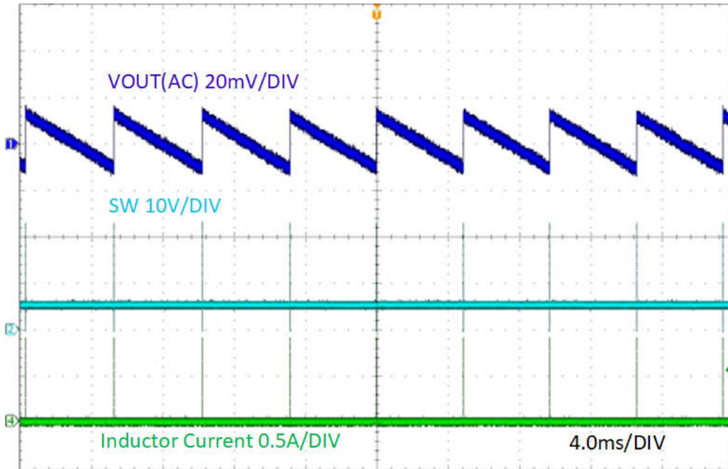
图 3-6. TPS54538EVM 输出电压纹波, I_{OUT} = 0A , Eco-mode
