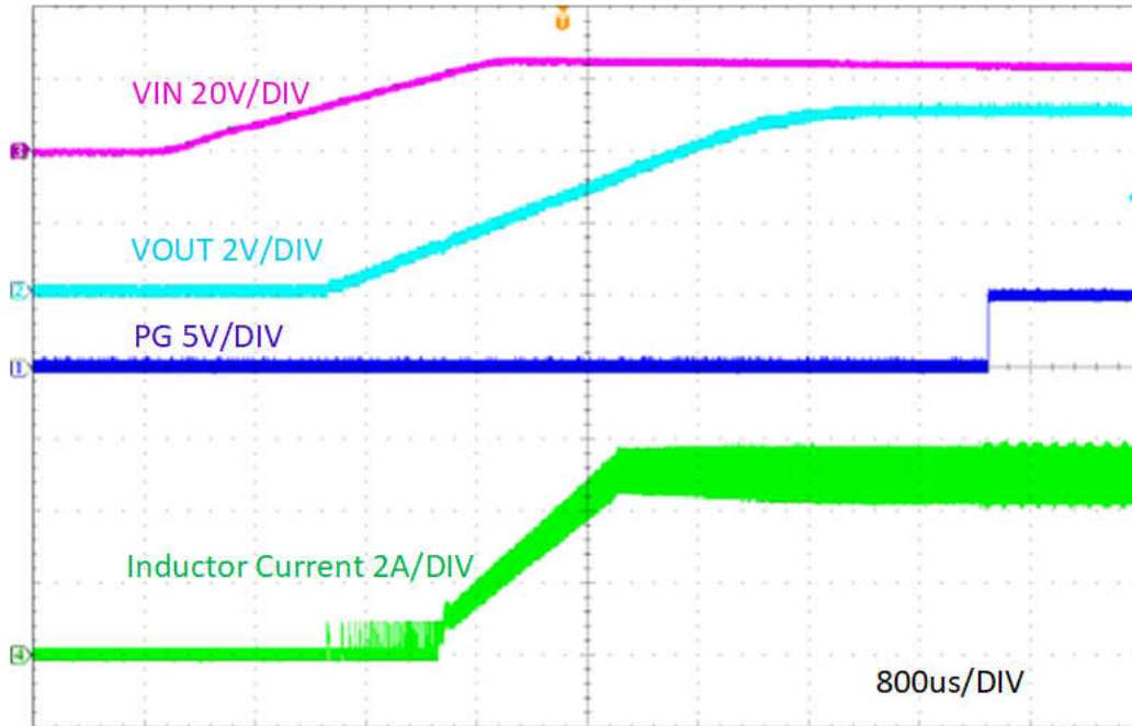
图 3-4. 相对于 VIN 的启动，EN 悬空， I_{OUT} = 5A
