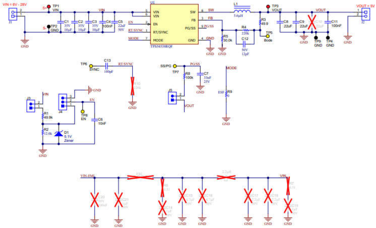
图 4-1. TPS54538EVM 原理图
