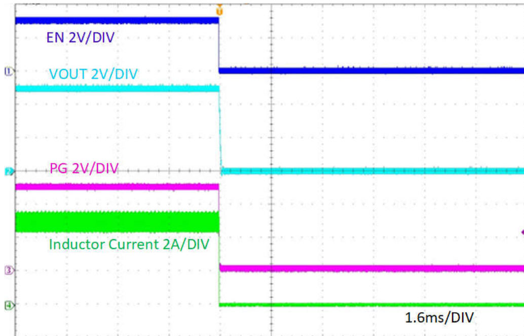
图 3-3. 相对于 EN 的关断, V_{IN} = 24V , I_{OUT} = 5A
