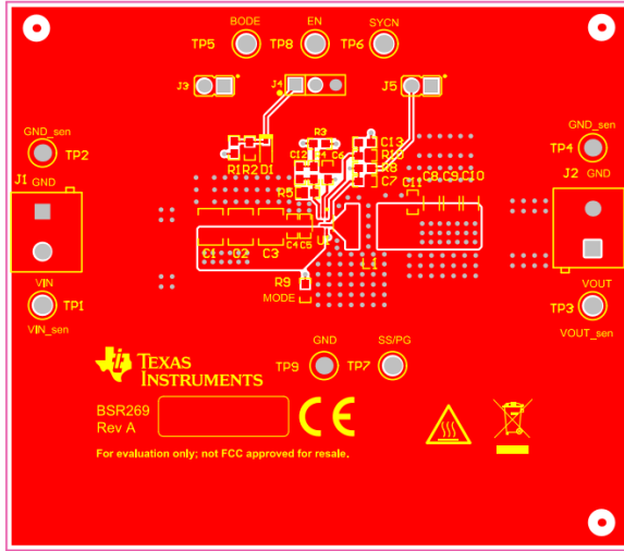
图 4-2. 顶层铜 (顶视图)
