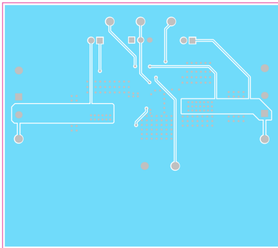
图 4-4. 第 3 层覆铜 (顶视图)
