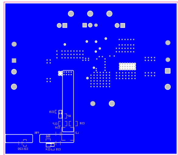
图 4-5. 底层覆铜 (顶视图)
