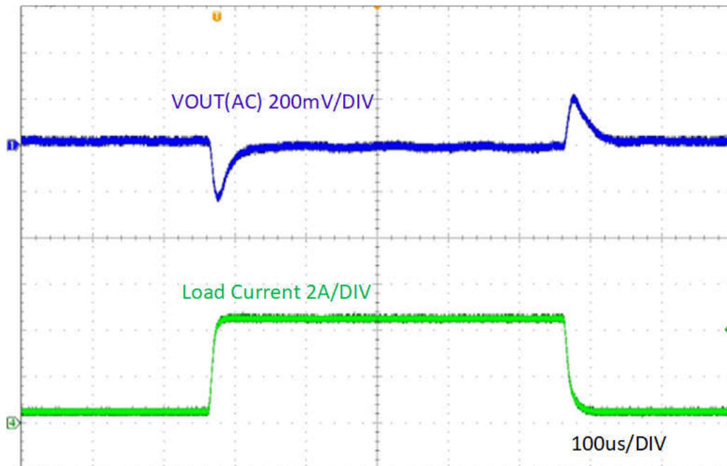
图 3-5. V_{IN} = 24V 、以 1.6A/\mu s 的速度从 0.5A 变为 4.5A 时的负载瞬态响应
