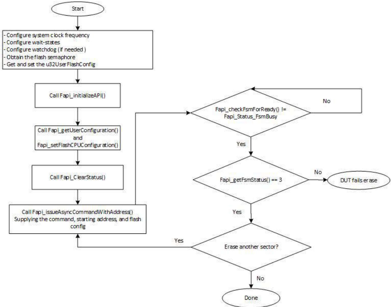
图 5-1. 推荐的擦除流程
