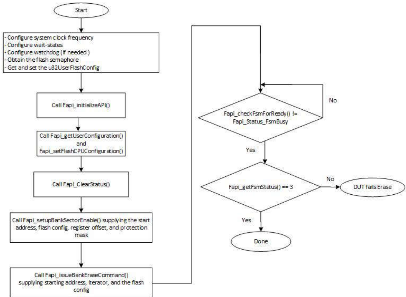
图 5-2. 推荐的闪存组擦除流程
