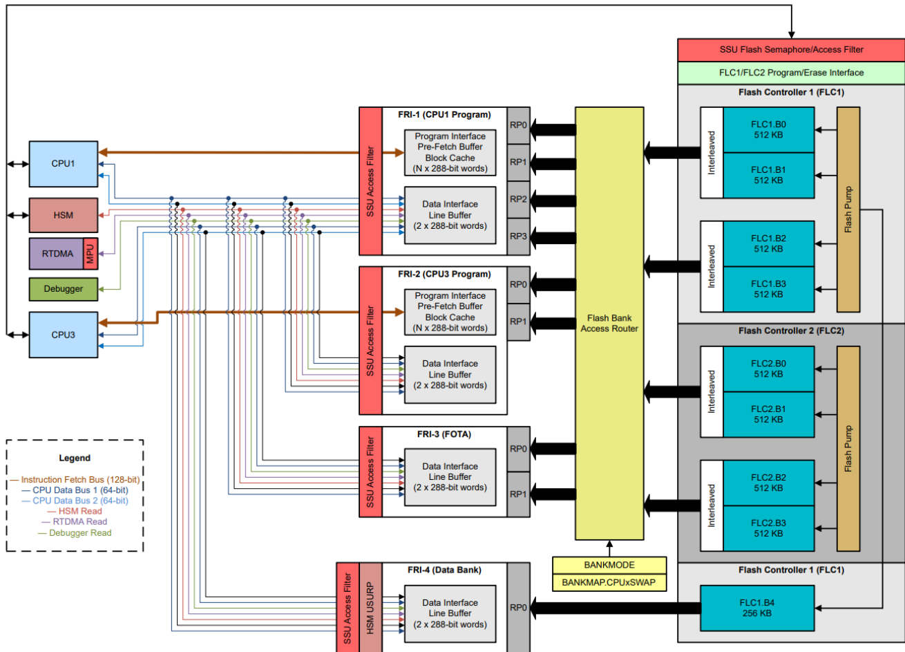
图 1-1. F29H85x 闪存架构
