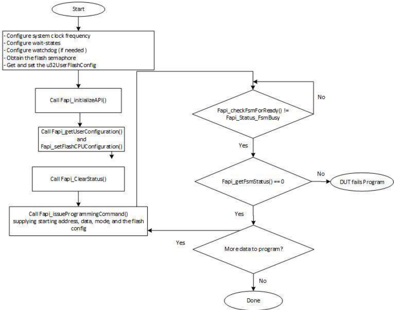
图 5-3. 推荐的编程流程
