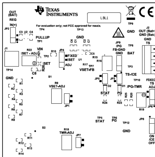
图 3-2. 顶层丝印层
