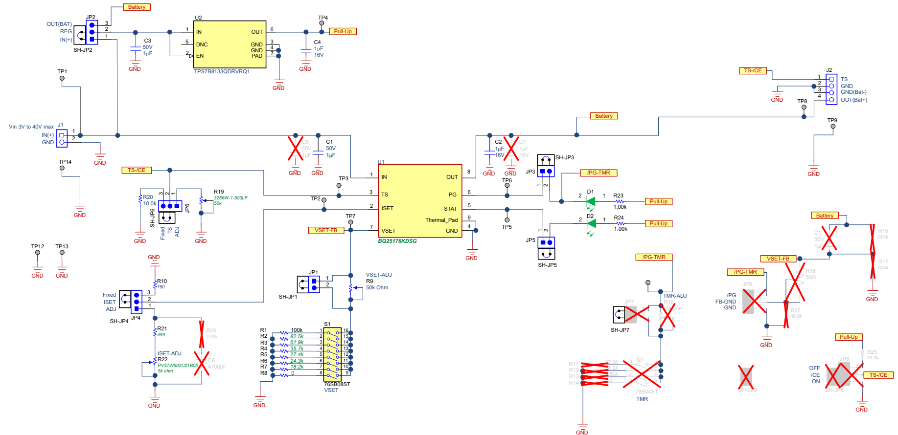
图 3-1. BQ25176KEVM 原理图
