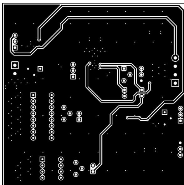
图 3-5. 底层
