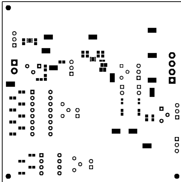
图 3-3. 顶部焊锡层
