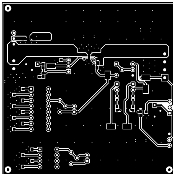
图 3-4. 顶层
