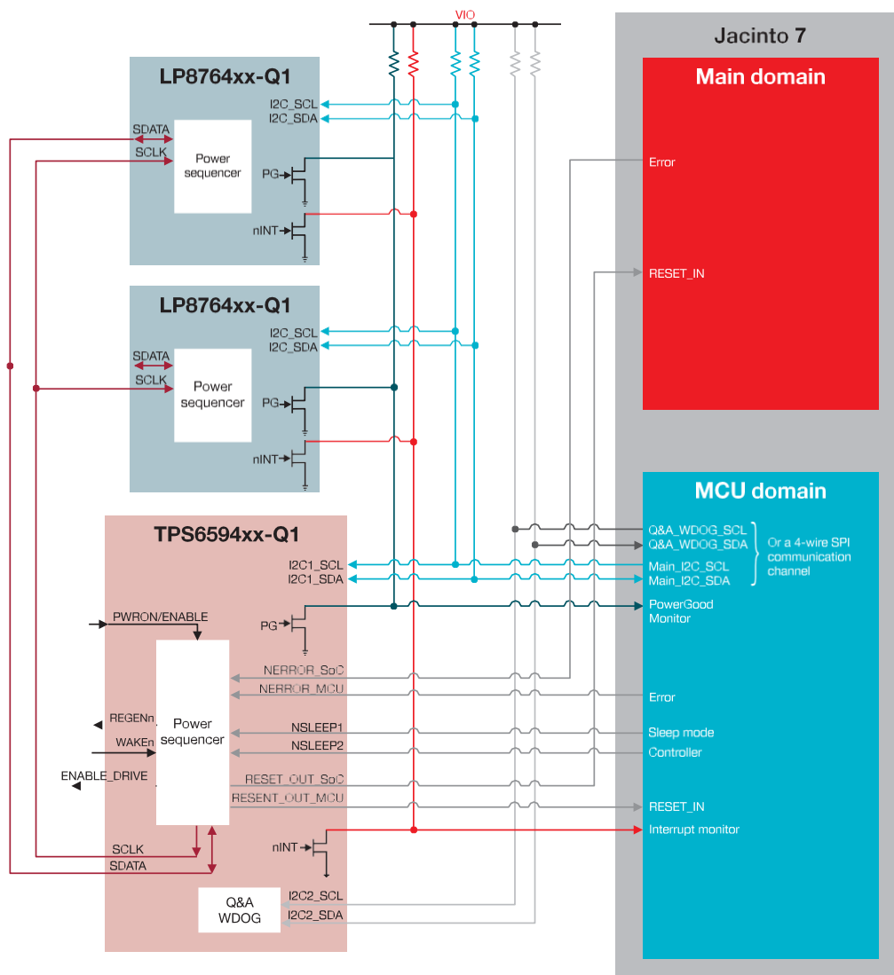
图 2. 作为“虚拟”PMIC 的 TPS6594-Q1 + LP8764-Q1 + LP8764-Q1 通信
