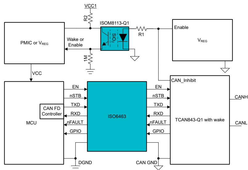
图 1. 基于 ISOM8113-Q1 且具有隔离式唤醒检测功能的继电器分立式 CAN 电路
