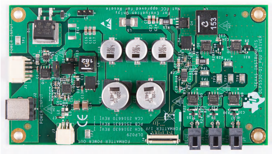
图 1-2. DLP5530PROJQ1EVM 照明驱动器 PCB
