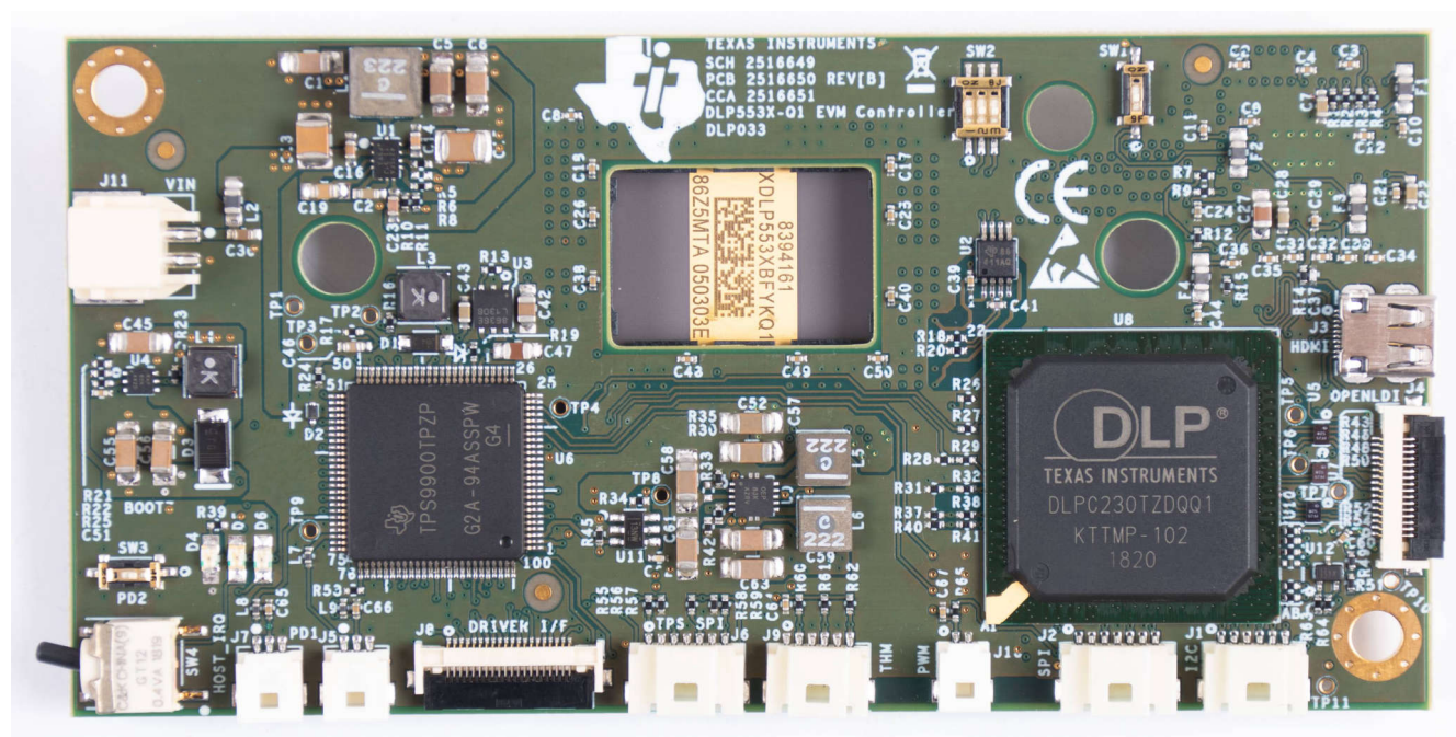
图 1-1. DLP5530PROJQ1EVM 控制器 PCB
