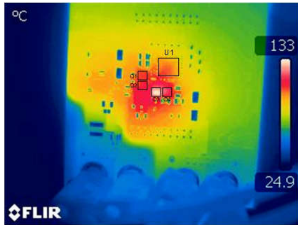
图 3-6. 热像图 : V_{IN} = 9.0V , V_{OUT} = 28.0V , I_{OUT} = 1.8A , 无强制空气冷却
