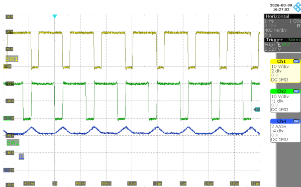
图 3-13. SW1、SW2、 I_L ( V_{IN} = 20V , V_{OUT} = 20V , I_{OUT} = 3A )
