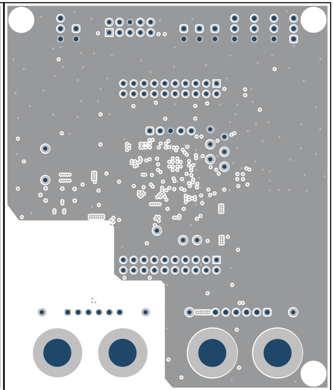
图 4-7. 中间层 3
