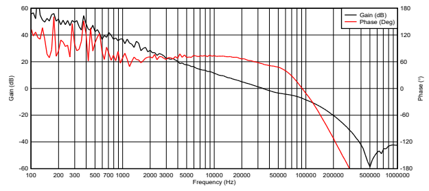
图 3-22. 控制环路响应, V_{IN} = 20V , V_{OUT} = 28V , I_{OUT} = 1.8A
