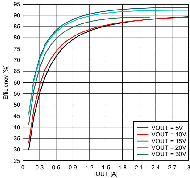
图 3-7. 效率与输出电流间的关系曲线 ( V_{IN} = 12V 时)
