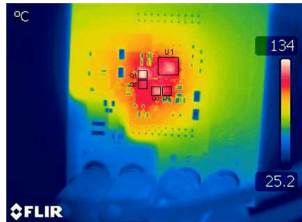
图 3-5. 热像图 : V_{IN} = 38.0V , V_{OUT} = 28.0V , I_{OUT} = 3.0A , 无强制空气冷却
