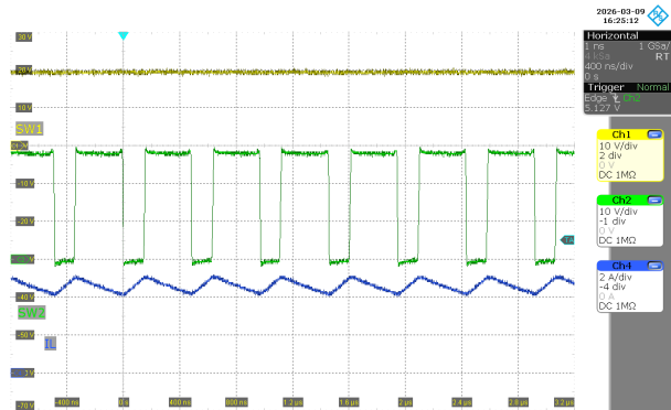
图 3-14. SW1、SW2、 I_L ( V_{IN} = 20V , V_{OUT} = 28V , I_{OUT} = 3A )
