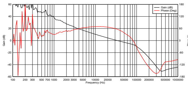
图 3-19. 控制环路响应, V_{IN} = 12V , V_{OUT} = 5V , I_{OUT} = 3.0A
