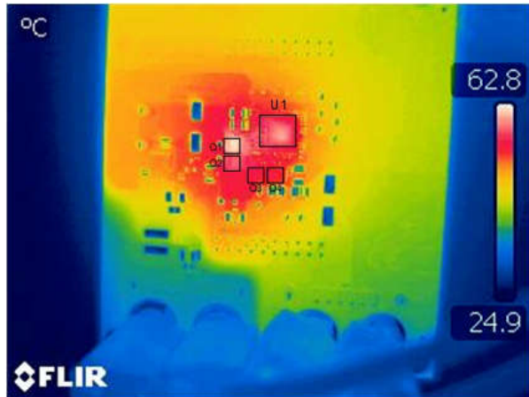
图 3-2. 热像图 : V_{IN} = 20.0V , V_{OUT} = 5.0V , I_{OUT} = 3.0A , 无强制空气冷却
