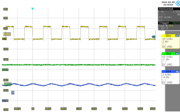
图 3-9. SW1、SW2、 I_L ( V_{IN} = 12V , V_{OUT} = 5V , I_{OUT} = 3A )
