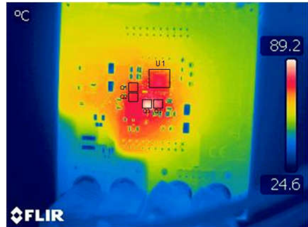
图 3-3. 热像图 : V_{IN} = 20.0V , V_{OUT} = 28.0V , I_{OUT} = 1.8A , 无强制空气冷却
