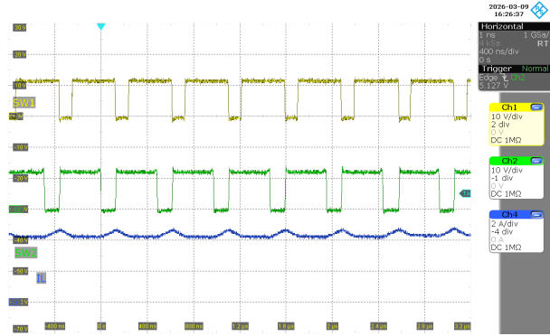
图 3-10. SW1、SW2、 I_L ( V_{IN} = 12V , V_{OUT} = 12V , I_{OUT} = 3A )
