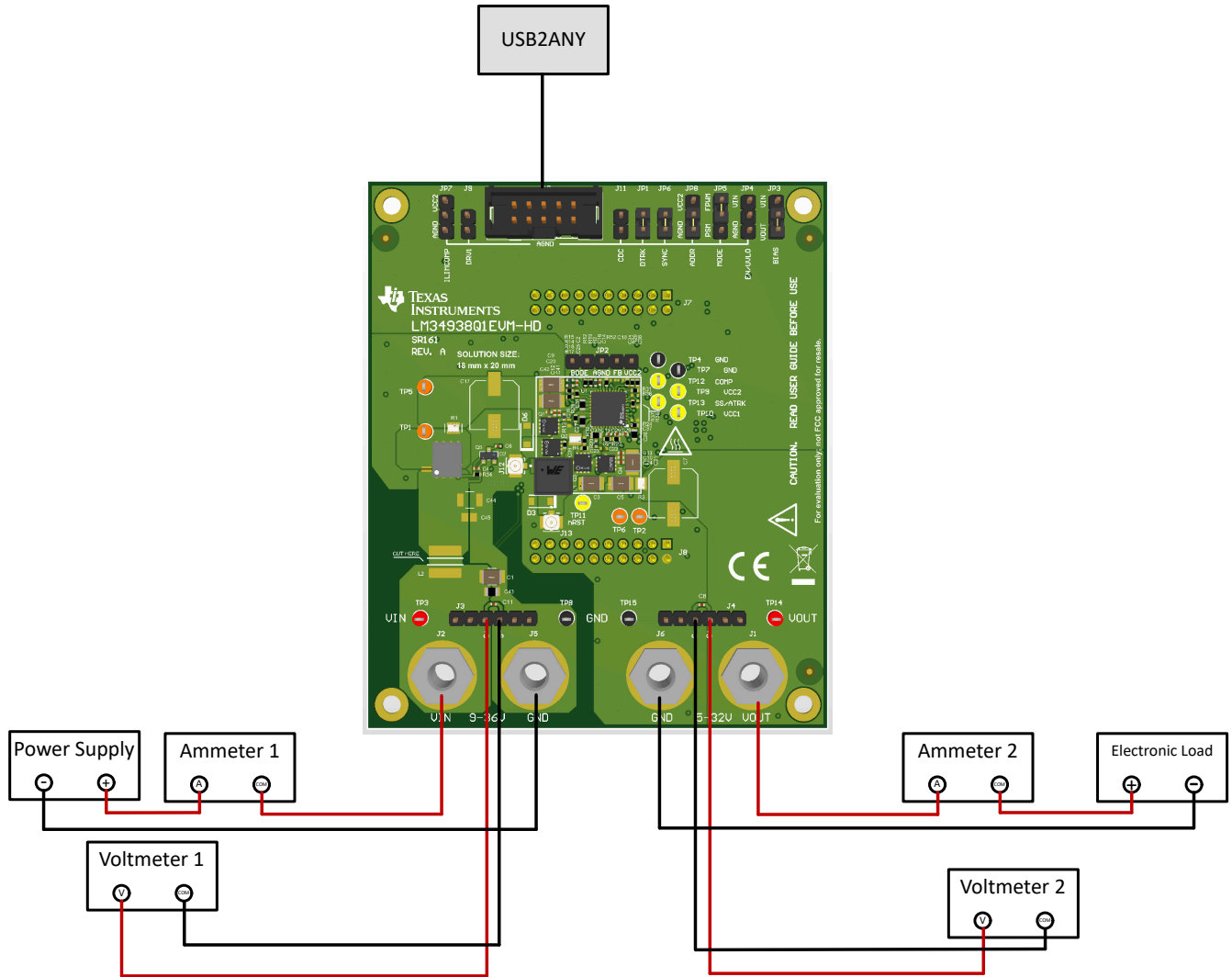
图 3-1. 典型的 EVM 连接图
