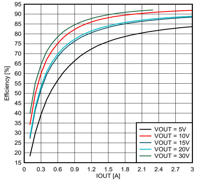
图 3-8. 效率与输出电流间的关系曲线 ( V_{IN} = 20V 时)
