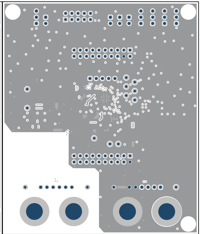
图 4-5. 中间层 1
