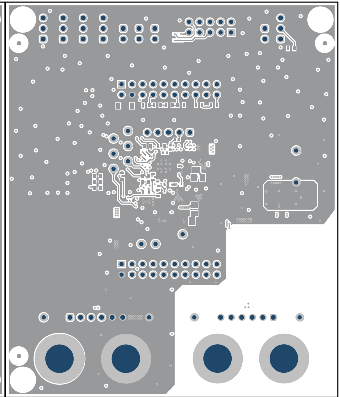
图 4-9. 底层
