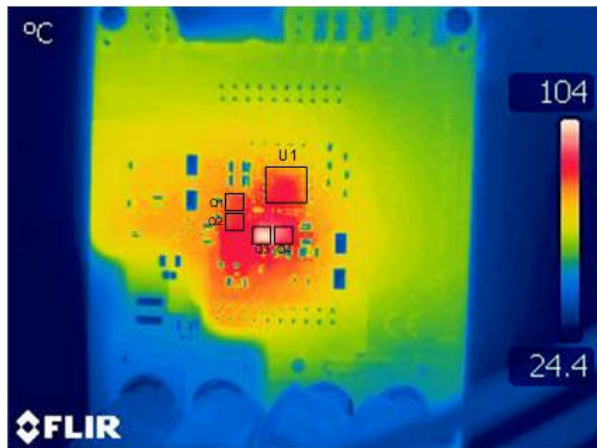
图 3-4. 热像图 : V_{IN} = 20.0V , V_{OUT} = 28.0V , I_{OUT} = 3.0A , 无强制空气冷却
