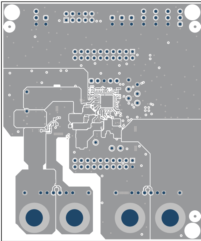
图 4-4. 顶层
