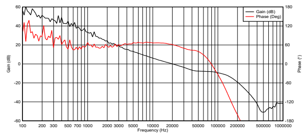
图 3-20. 控制环路响应, V_{IN} = 12V , V_{OUT} = 28V , I_{OUT} = 1.8A
