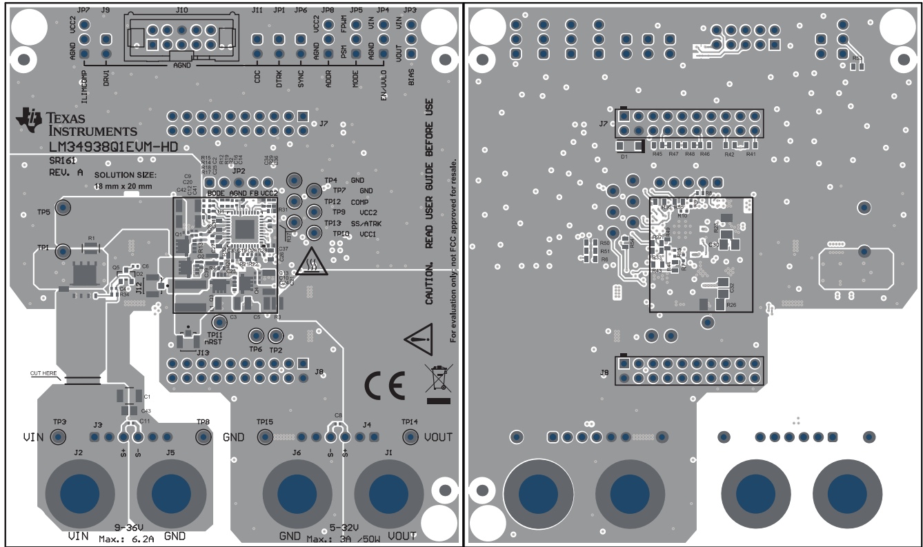
图 4-2. 顶部丝印
