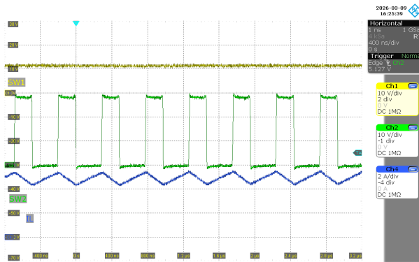
图 3-11. SW1、SW2、 I_L ( V_{IN} = 12V , V_{OUT} = 28V , I_{OUT} = 1.8A )
