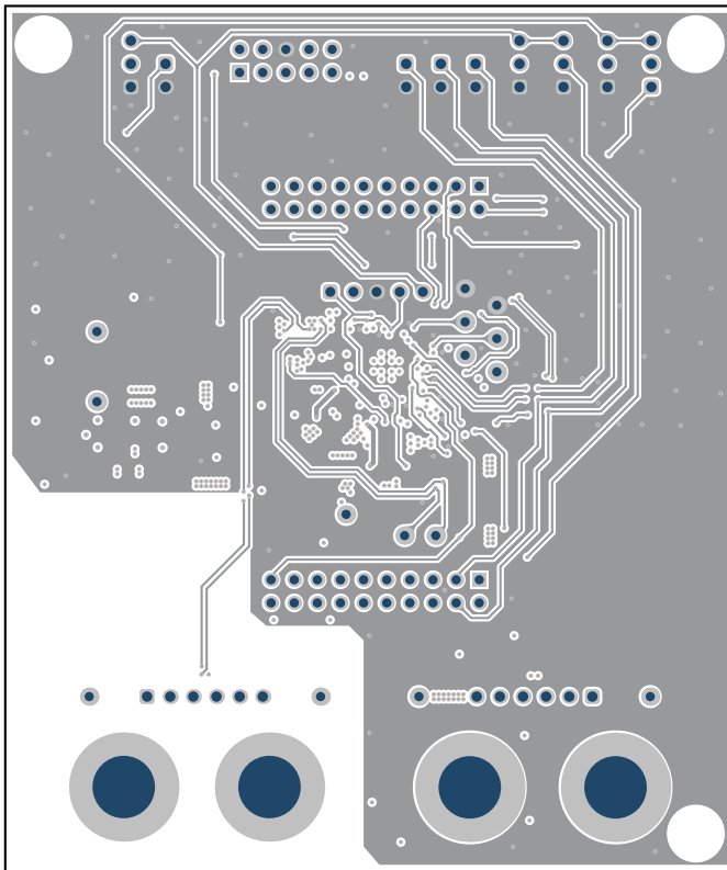
图 4-6. 中间层 2
