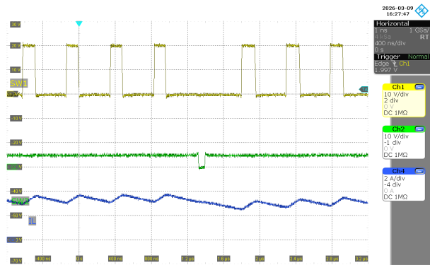
图 3-12. SW1、SW2、 I_L ( V_{IN} = 20V , V_{OUT} = 5V , I_{OUT} = 3A )
