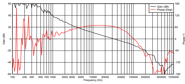
图 3-21. 控制环路响应, V_{IN} = 20V , V_{OUT} = 5V , I_{OUT} = 3A
