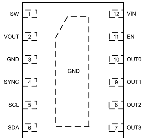
図 5-2. LP5813 DRR パッケージ、12 ピン WSON (上面図)
