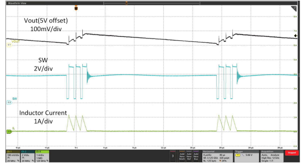
図 9-12. 軽負荷時のスイッチング波形
