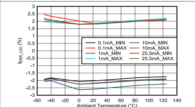
図 6-6. チャンネル間の電流精度と温度との関係 (MC = 0)
