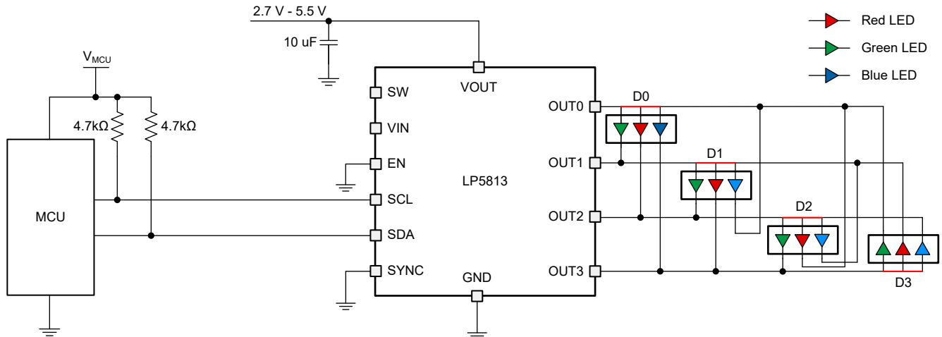
図 9-2. 代表的なアプリケーション - 昇圧コンバータをバイパスした LP5813
