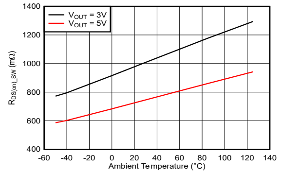
図 6-10. スキャンラインスイッチ MOSFET R_{DS(on)}
