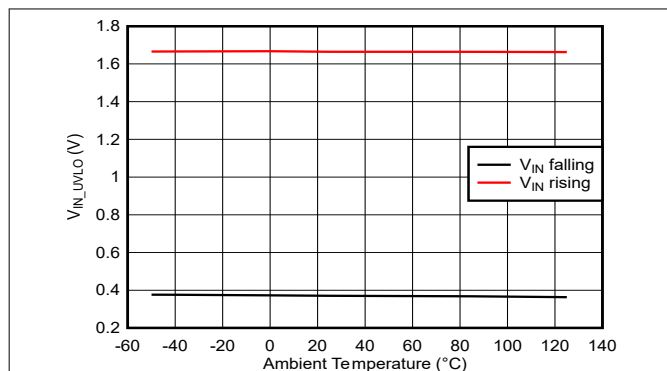
図 6-1. VIN UVLO の立ち上がりおよび立ち下がりスレッシュホールド
