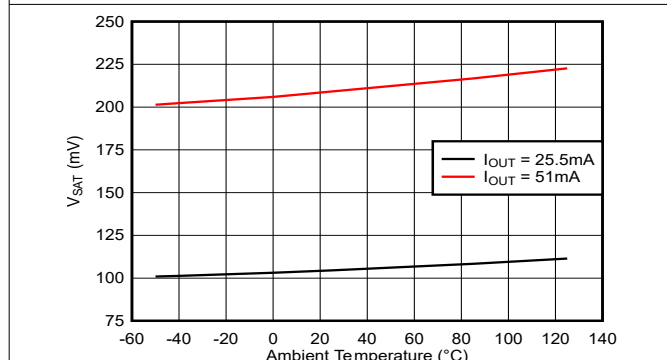
図 6-5. V SAT と温度との関係
