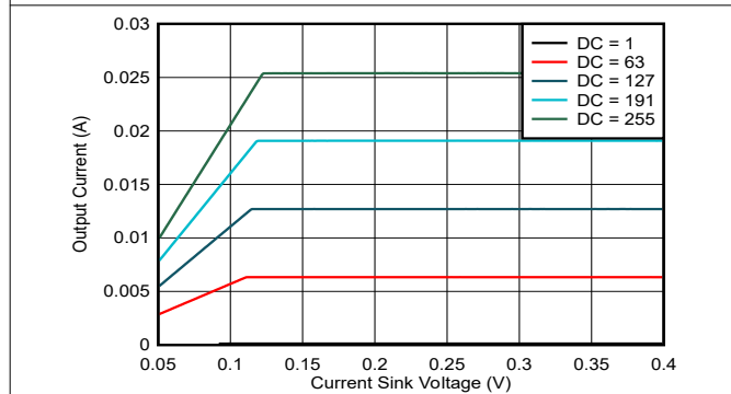
図 6-3. 電流シンク電圧と電流との関係 (MC = 0)
