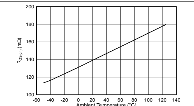
図 6-8. 昇圧ハイサイド MOSFET R DS(on)
