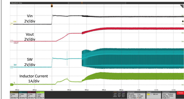
図 9-11. 重負荷時のスイッチング波形
