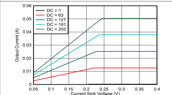
図 6-4. 電流シンク電圧と電流との関係 (MC = 1)
