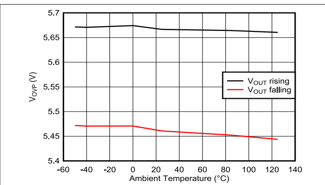
図 6-2. VOUT OVP スレッシュホールド
