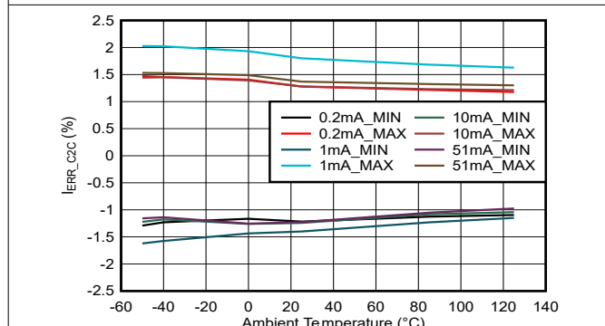
図 6-7. チャンネル間の電流精度と温度との関係 (MC = 1)
