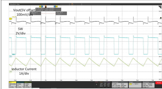
図 9-11. 重負荷時のスイッチング波形
