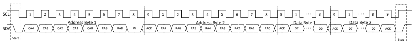
図 7-22. I 2 C 書き込みタイミング
