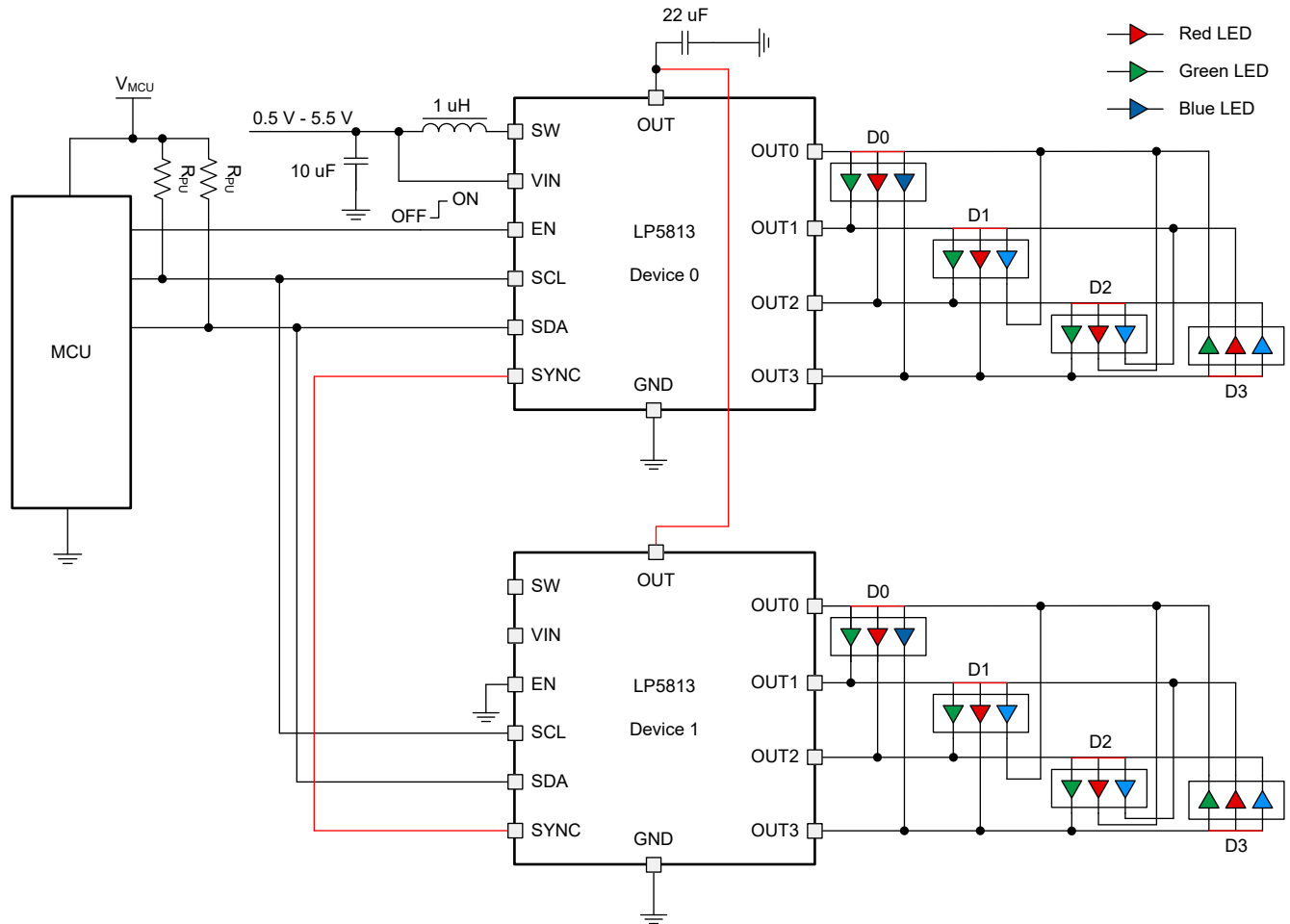
図 9-3. 代表的なアプリケーション - デュアル LP5813 アプリケーションの例
