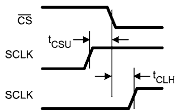
SCLK and \overline{CS} Timing Parameters
