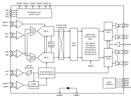
ADC12DJ5200-EP ブロック図
