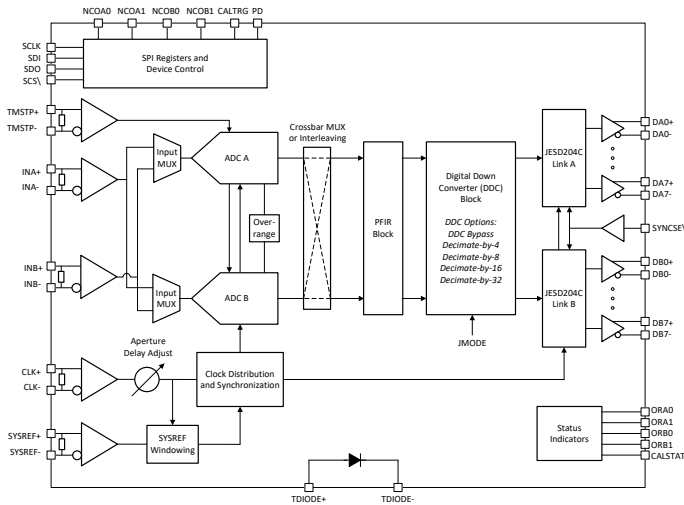
ADC12DJ5200-SP ブロック図
