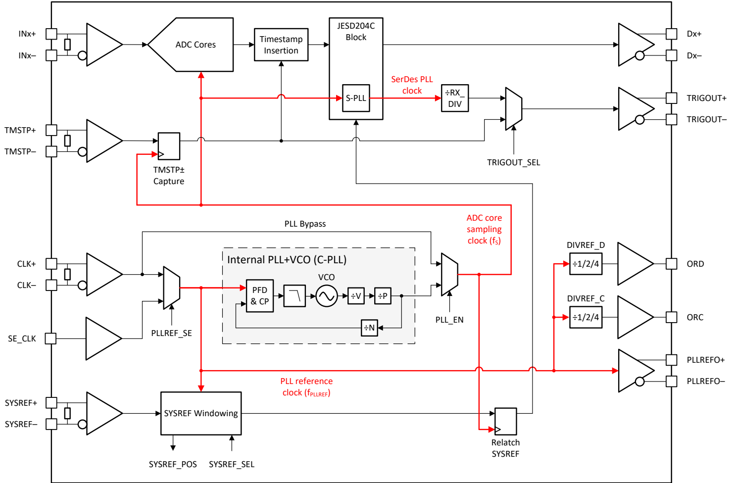
図 6-3. Clocking Subsystem
