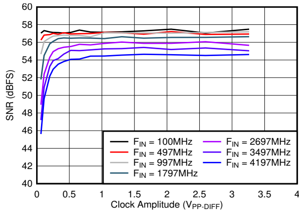
5-37. SNR vs A CLK
