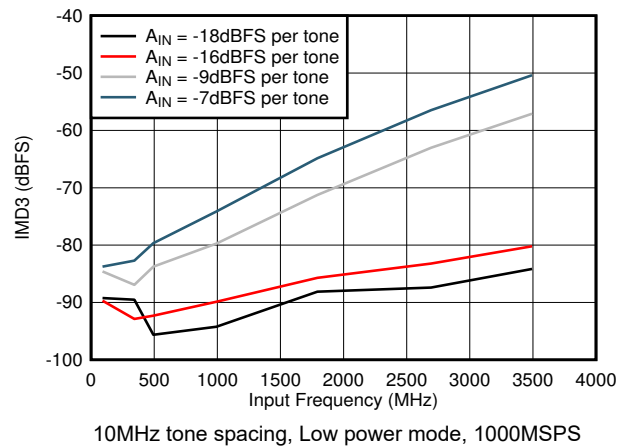
5-76. IMD3 vs F_{IN}
