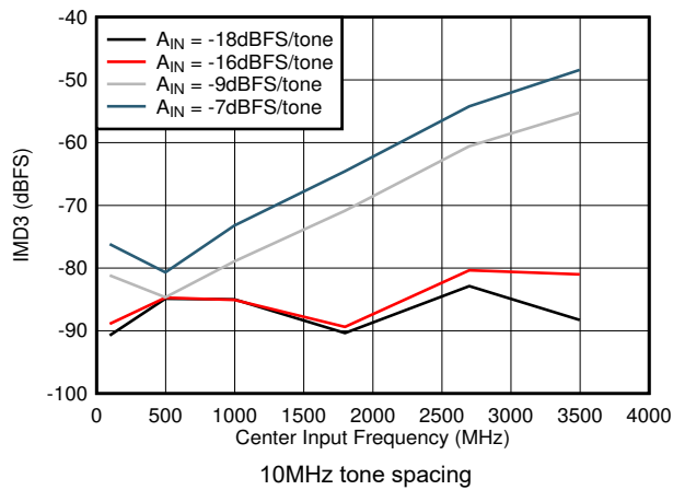
5-75. IMD3 vs F_{IN}
