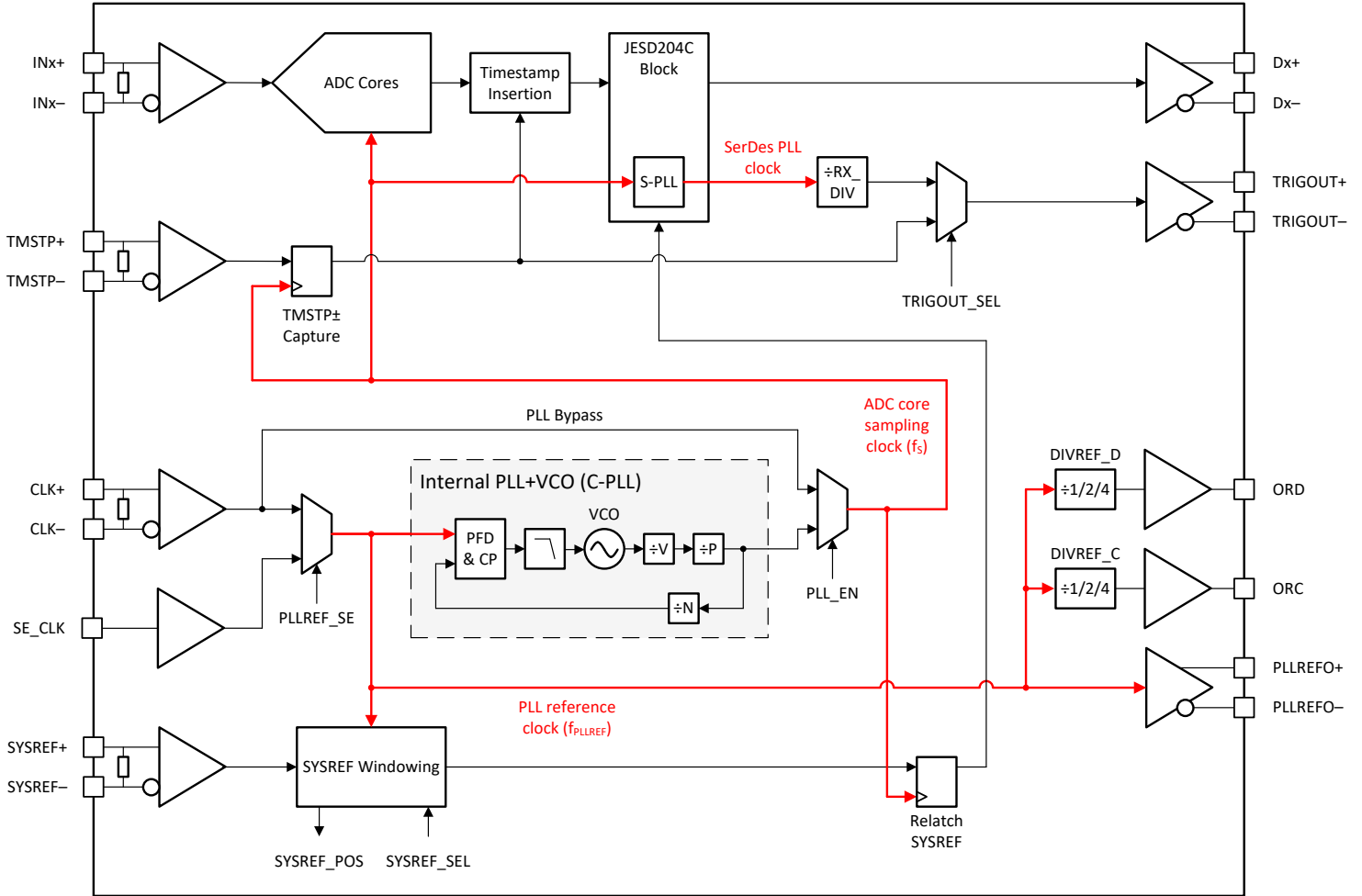
8-3. Clocking Subsystem
