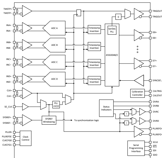
クワッド・チャネルのブロック図
