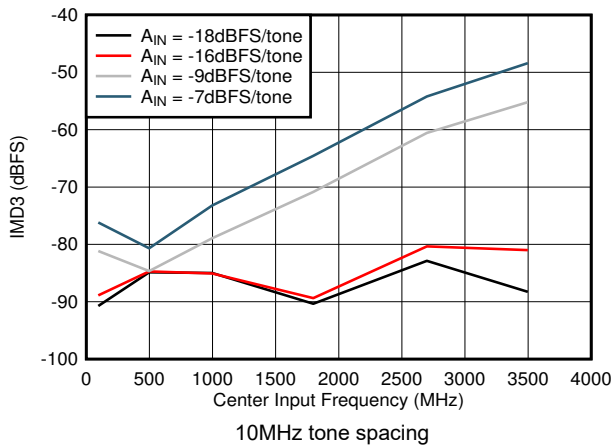
7-75. IMD3 vs F_{IN}
