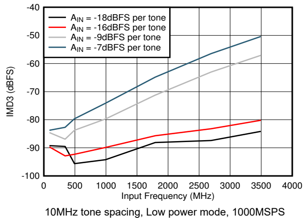
7-76. IMD3 vs F_{IN}
