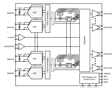
ブロック図
