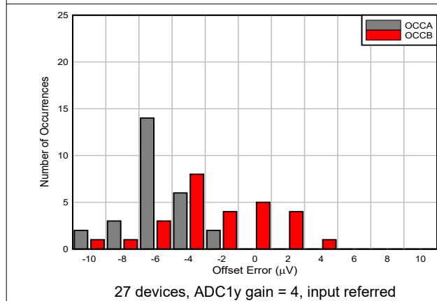
7-16. OCCy Offset Error Histogram
