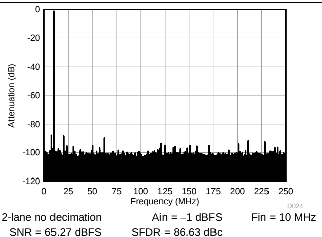
FIG 28. FFT 10 MHz
