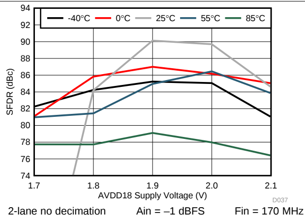
图 41. SFDR vs AVDD18 Supply Voltage
