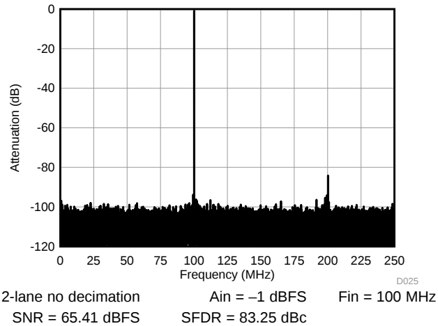
图 29. FFT 100 MHz
