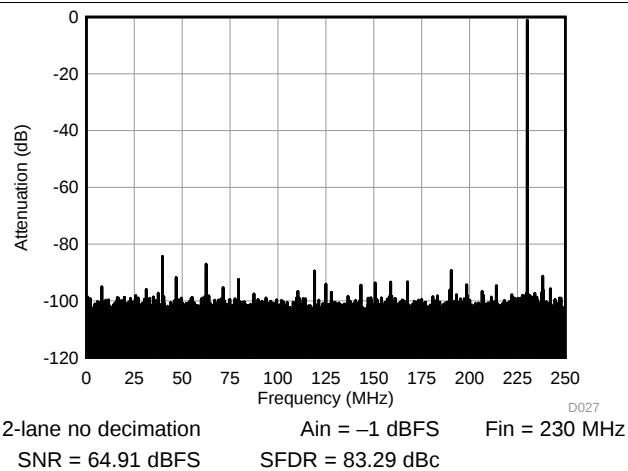
图 31. FFT 230 MHz
