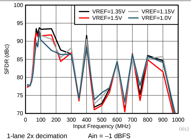
FIG 16. SFDR vs. VREF
