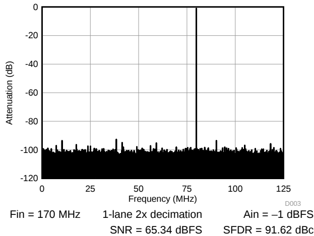
图 7. FFT 170 MHz
