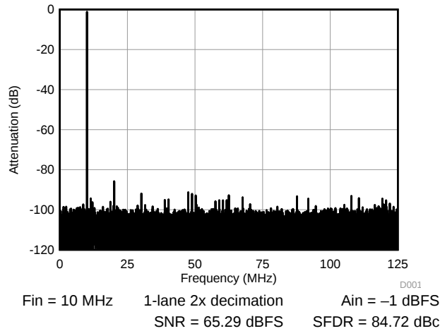
图 5. FFT 10 MHz
