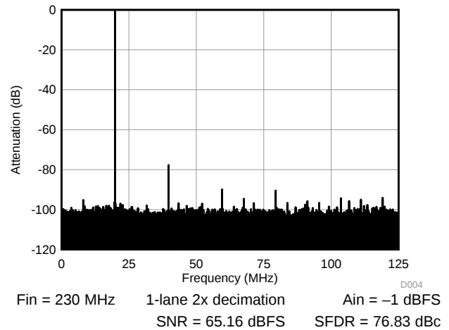
图 8. FFT 230 MHz
