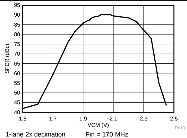
FIG 14. SFDR vs. VCM
