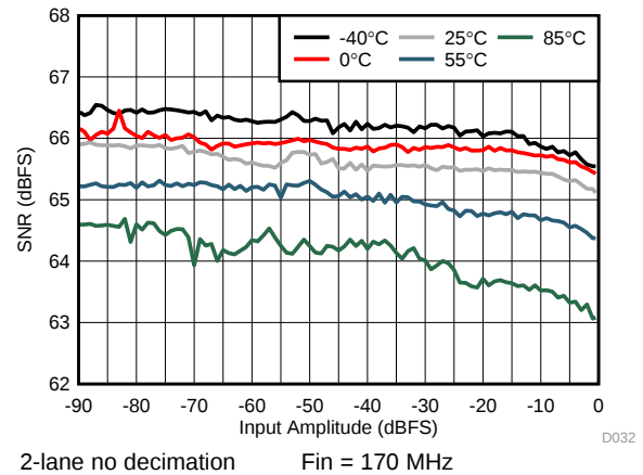
图 36. SNR vs Amplitude
