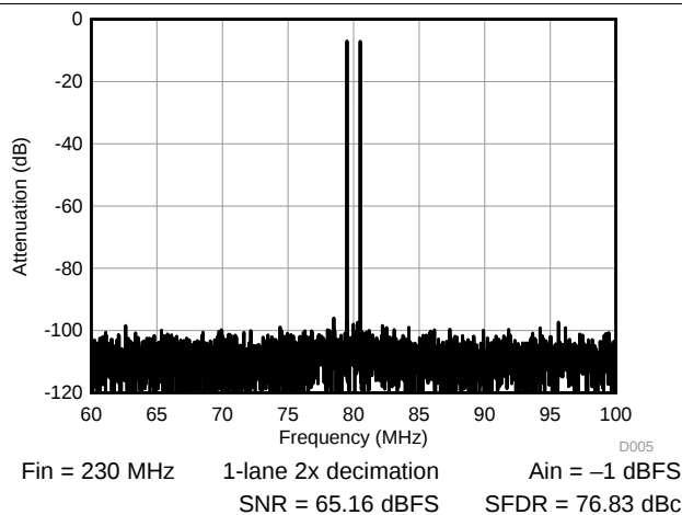
图 9. 2-Tone FFT
