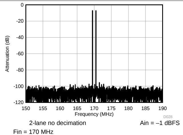
图 32. 2-Tone FFT
