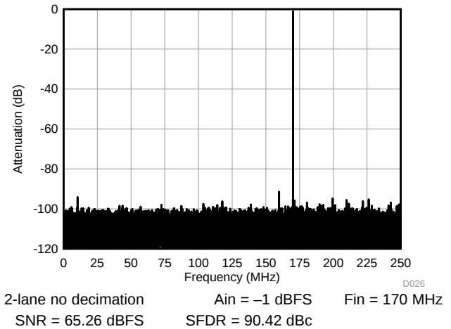
图 30. FFT 170 MHz
