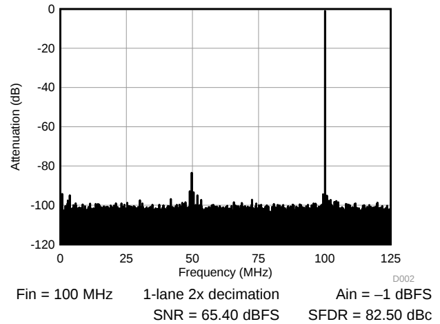
图 6. FFT 100 MHz
