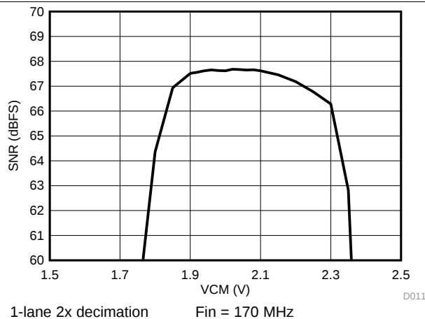
FIG 15. SNR vs VCM
