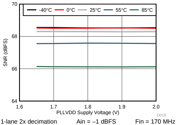
FIG 23. SNR vs PLLVDD
