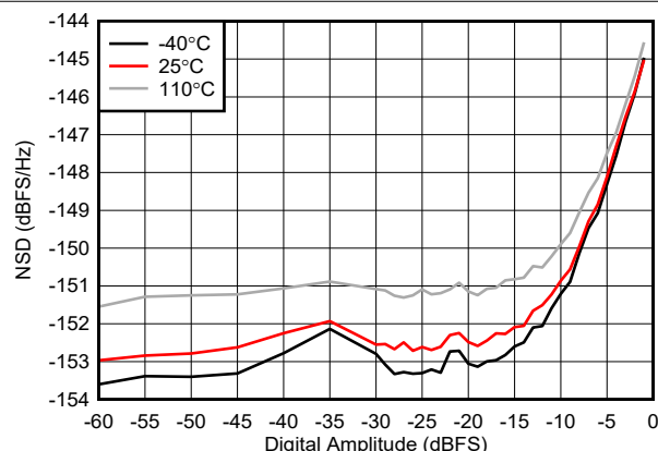
図 4-261. TX NSD とデジタル振幅との関係 (9.61GHz)
