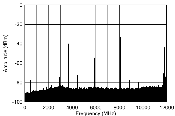
図 4-213. TX デュアル トーン出力スペクトル (8.1GHz)
