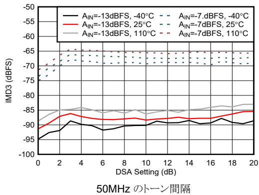
図 4-446. RX IMD3 と DSA 設定との関係 (8.11GHz)
