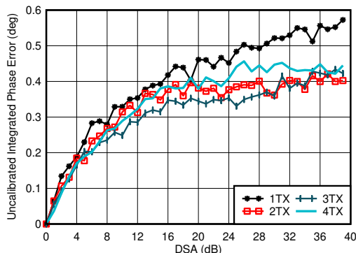
図 4-126. TX 未校正積分位相誤差と DSA 設定との関係 (チャンネル 1、3.5GHz)
