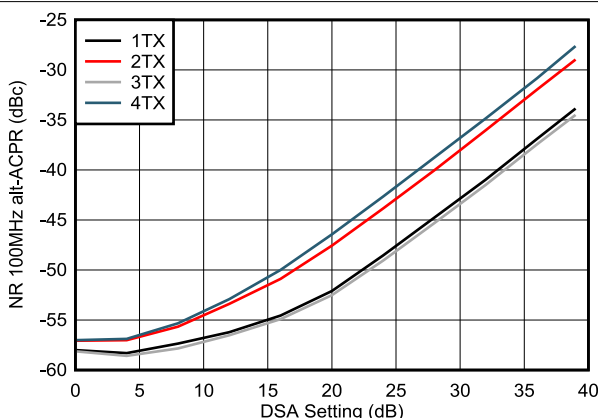
図 4-282. TX NR100MHz alt-ACPR と DSA 設定との関係 (9.61GHz)
