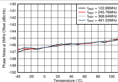
図 4-503. 5MHz オフセット時の 12GHz VCO の位相ノイズと温度の関係 ( f_{OUT} = 2.6\text{GHz} のとき f_{REF} )
