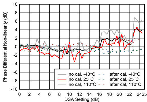
図 4-470. RX 位相の積分非線形性 (9.6GHz)
