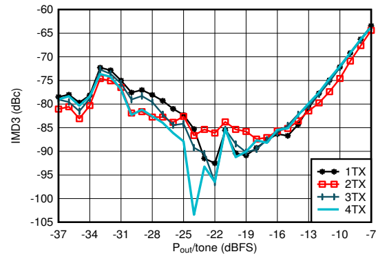
図 4-28. TX IMD3 とデジタル レベルとの関係 (0.85GHz)
