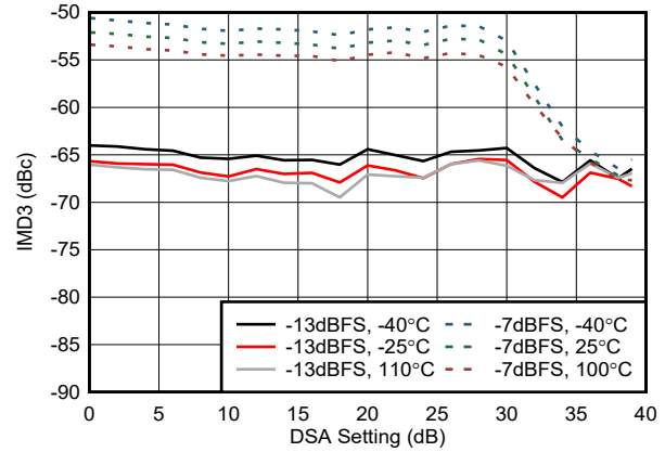
図 4-256. TX IMD3 と DSA 設定との関係 (9.61GHz)
