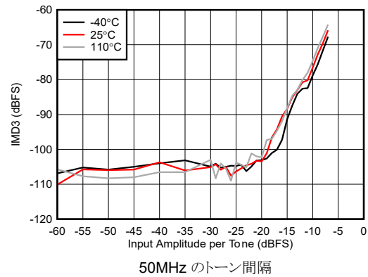
図 4-445. RX IMD3 と入力振幅との関係 (8.11GHz)
