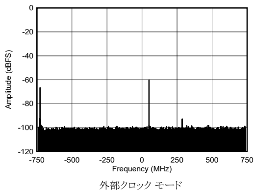
図 4-460. RX シングル トーン出力 FFT (8.11GHz、-60dBFS)
