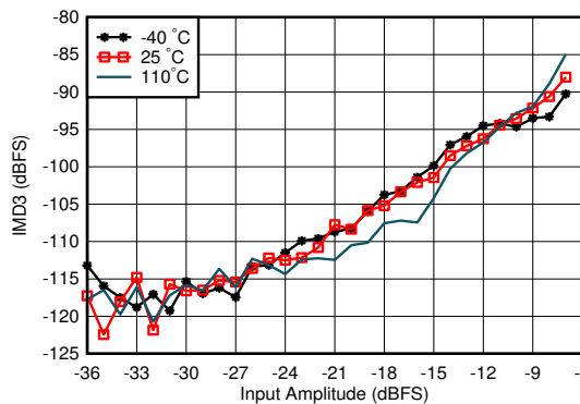
図 4-335. RX IMD3 と入力レベルとの関係 (各種温度、1.75GHz)
