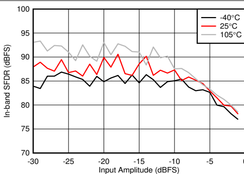
2.6GHz 整合あり、1/4 にデシメーション
