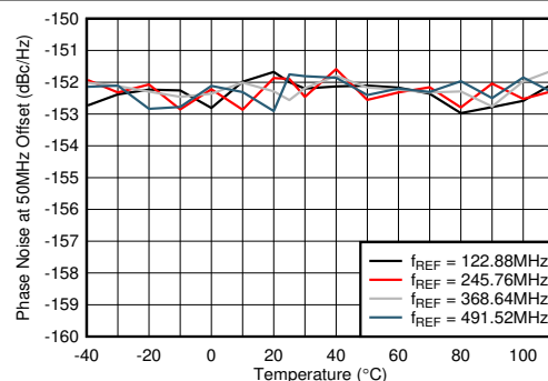
図 4-504. 50MHz オフセット時の 12GHz VCO の位相ノイズと温度の関係 ( f_{OUT} = 2.6\text{GHz} のとき f_{REF} )
