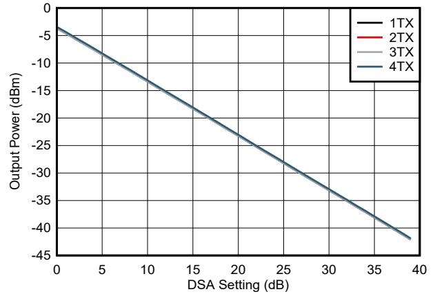
図 4-185. TX 出力電力と DSA 設定との関係 (8.1GHz)
