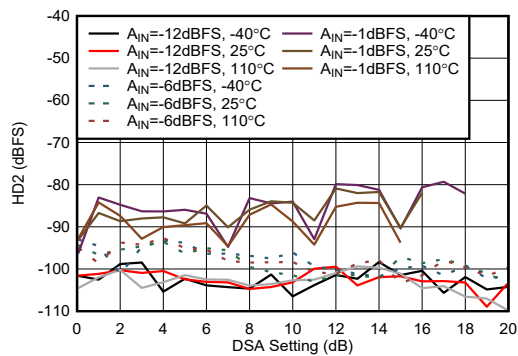
図 4-453. RX HD2 と DSA 設定との関係 (8.11GHz)
