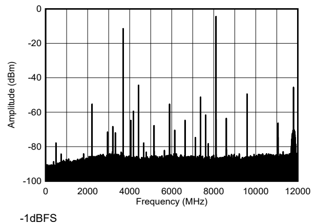
図 4-203. TX シングル トーン出力スペクトル (8.11GHz)
