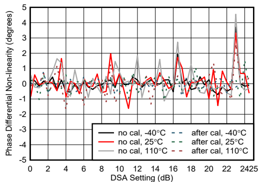
図 4-469. RX 位相の微分非直線性 (9.6GHz)
