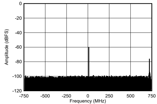
図 4-486. RX シングル トーン出力 FFT (9.61GHz)
