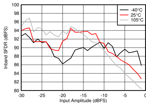
2.6GHz 整合あり、8 倍にデシメーション、DSA 設定 = 12dB
