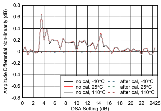
図 4-467. RX 振幅の微分非直線性 (9.6GHz)
