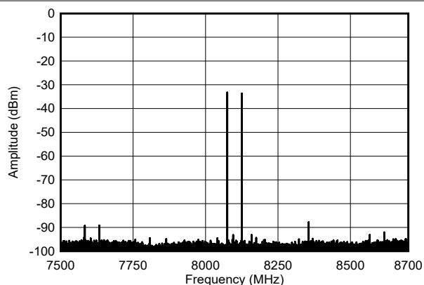
図 4-212. TX デュアル トーン出力スペクトル (8.1GHz)
