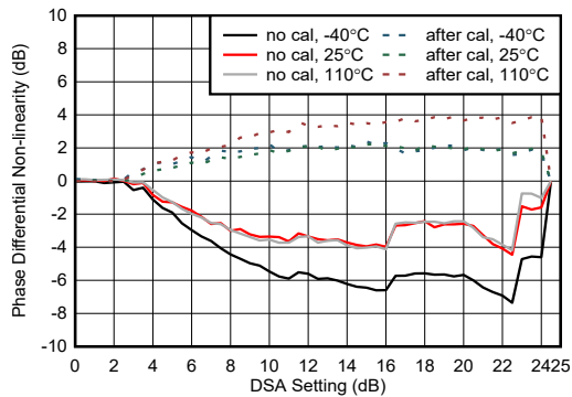
図 4-444. RX 位相の微分非直線性 (8.11GHz)
