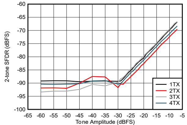
図 4-221. TX 2 トーン SFDR とデジタル振幅との関係 (8.1GHz)
