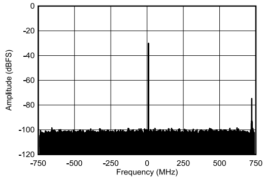
図 4-485. RX シングル トーン出力 FFT (9.61GHz)
