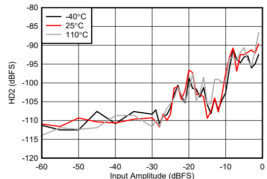
図 4-478. RX HD2 とデジタル レベルとの関係 (9.6GHz)
