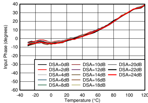
2.6GHz 整合あり、25°Cの位相で正規化
