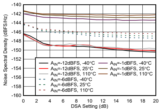
図 4-477. RX NSD と DSA 設定との関係 (9.6GHz)
