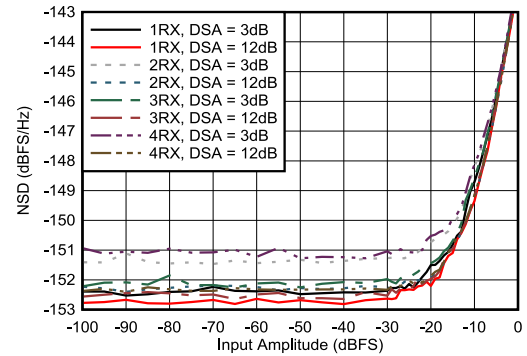
図 4-476. RX NSD とデジタル振幅との関係 (9.6GHz)
