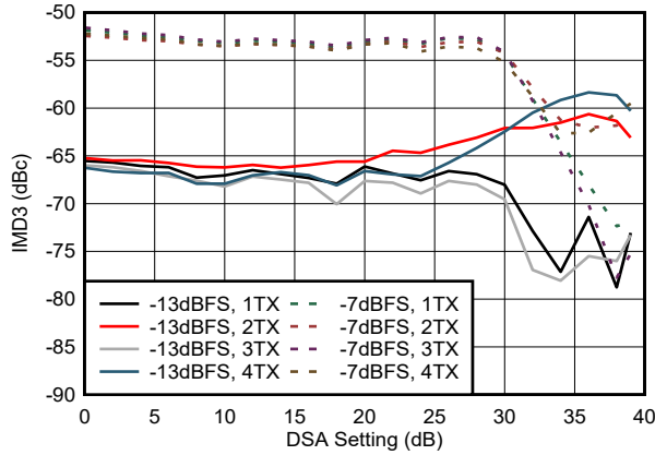
図 4-255. TX IMD3 と DSA 設定との関係 (9.61GHz)
