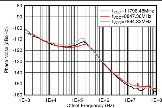
図 4-492. 位相ノイズとオフセット周波数との関係 (各種 f_{\text{VCO}} 、 f_{\text{OUT}} = 2610\text{MHz} )
