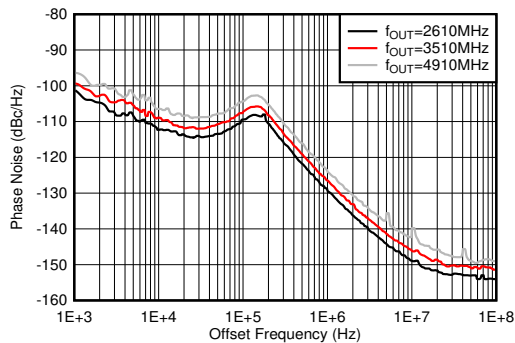
図 4-517. 9GHz VCO の位相ノイズとオフセット周波数との関係 (各種 f_{OUT} 、25°C)
