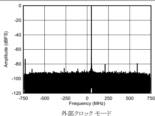
図 4-457. RX シングル トーン出力 FFT (8.11GHz、-1dBFS)
