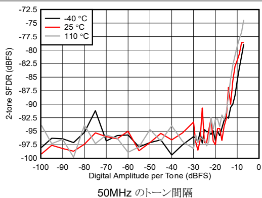
図 4-456. RX 2 トーン SFDR とデジタル振幅との関係 (8.11GHz)
