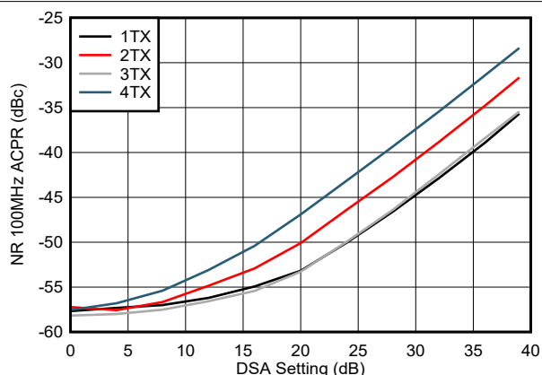
図 4-281. TX NR100MHz ACPR と DSA 設定との関係 (9.61GHz)
