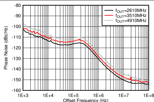
図 4-506. 10GHz VCO の位相ノイズとオフセット周波数との関係 (各種 f_{OUT} 、25°C)
