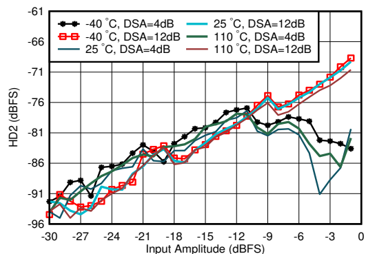
図 4-307. RX HD2 と DSA 設定との関係 (各種チャネル、0.8GHz)
