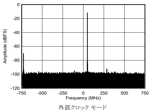
図 4-458. RX シングル トーン出力 FFT (8.11GHz、-12dBFS)
