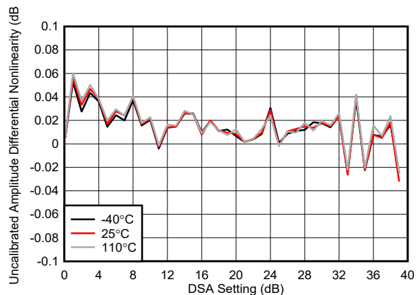
図 4-189. TX DSA 未校正振幅の微分非直線性 (8.11GHz)
