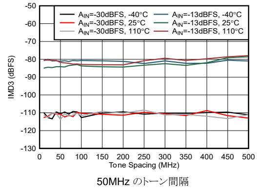
図 4-474. RX IMD3 と トーン間隔との関係 (9.6GHz)
