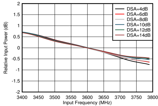
図 4-382. RX 帯域内ゲイン平坦性 ( f_{\text{IN}} = 3600\text{MHz} )
