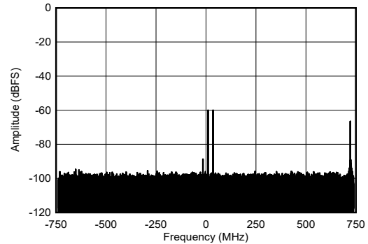
図 4-488. RX ツー トーン出力 FFT (9.61GHz)
