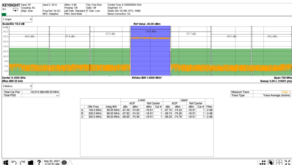
図 4-229. TX 100MHz NR 出カスペクトル (8.11GHz)
