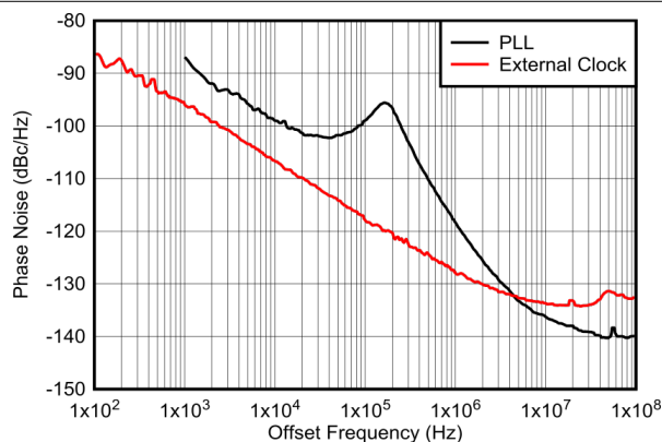
図 4-491. 位相ノイズとオフセット周波数との関係 (PLL、外部クロック、 12\text{GHz} )
