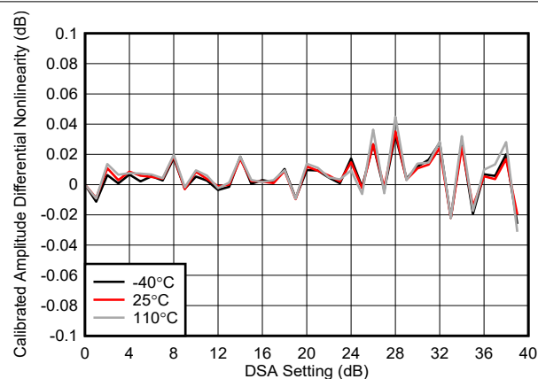
図 4-188. TX DSA 校正済み振幅の微分非直線性 (8.11GHz)
