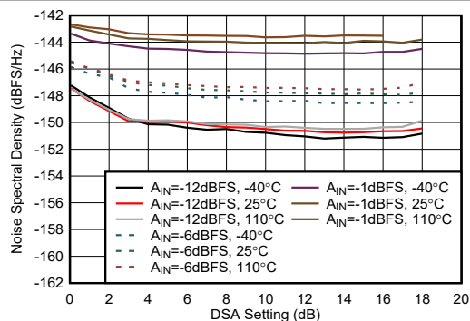
図 4-451. RX NSD と DSA 設定との関係 (8.11GHz)
