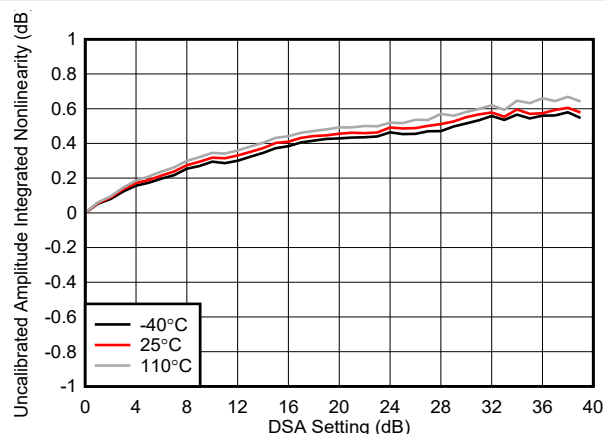
図 4-193. TX DSA 未校正振幅の積分非直線性 (8.11GHz)
