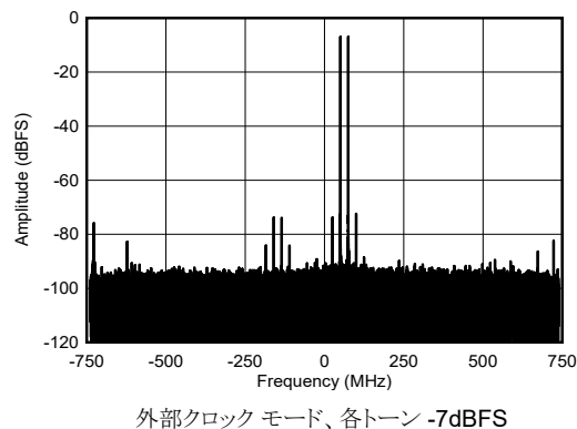
図 4-461. RX デュアル トーン出力 FFT (8.11GHz)
