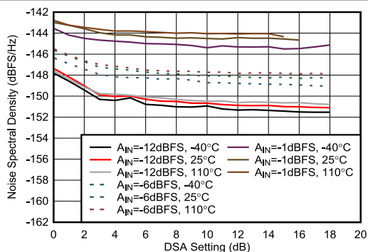
図 4-450. RX NSD と DSA 設定との関係 (8.11GHz)
