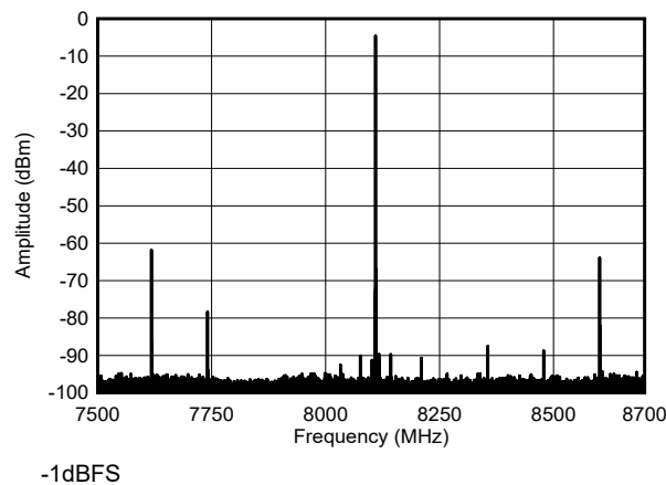
図 4-204. TX シングル トーン出力スペクトル (8.11GHz)
