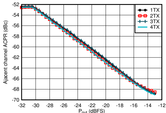
図 4-33. TX 20MHz LTE ACPR とデジタル レベルとの関係 (0.85GHz)
