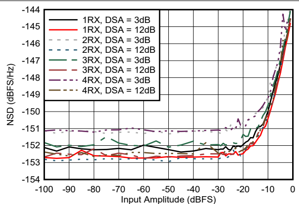
図 4-449. RX NSD とデジタル振幅との関係 (8.11GHz)
