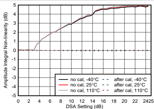
図 4-468. RX 振幅の積分非線形性 (9.6GHz)
