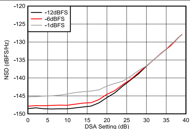
図 4-262. TX NSD と DSA 設定との関係 (9.61GHz)
