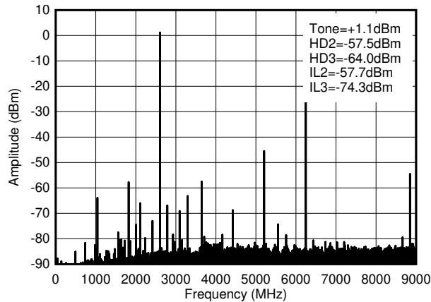
図 4-114. TX シングル トーン (-12dBFS) 出力スペクトル (0~ f_{\text{DAC}} 、2.6GHz)
