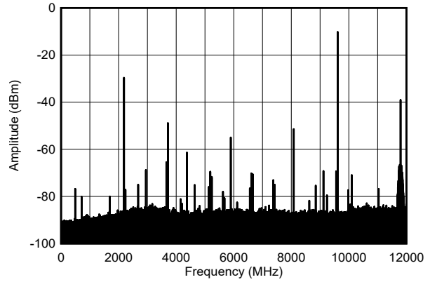
図 4-268. TX シングル トーン スペクトル (9.61GHz、-6dBFS、広帯域)
