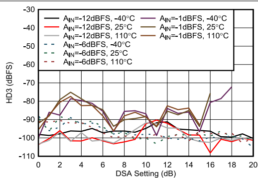
図 4-455. RX HD3 と DSA 設定との関係 (8.11GHz)
