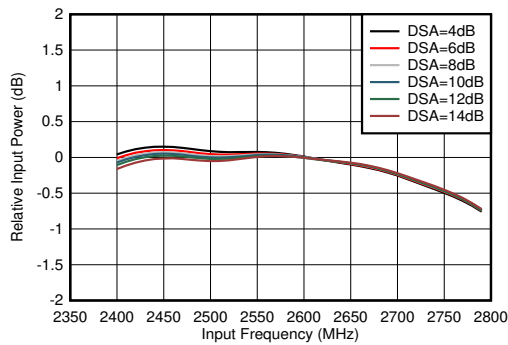
図 4-348. RX 帯域内ゲイン平坦性 ( f_{\text{IN}} = 2600\text{MHz} )
