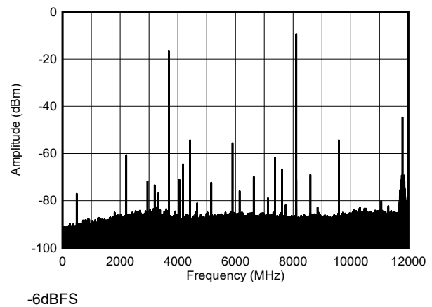
図 4-205. TX シングル トーン出力スペクトル (8.11GHz)
