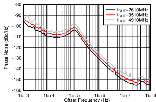
図 4-494. 12\text{GHz} VCO の位相ノイズとオフセット周波数との関係 (各種 f_{\text{OUT}} 、 25^\circ\text{C} )
