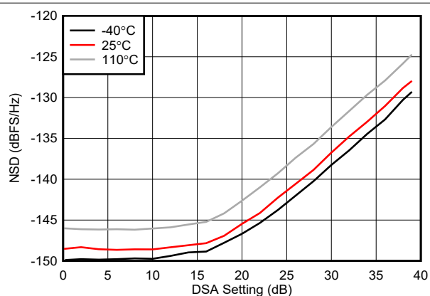
図 4-264. TX NSD と DSA 設定との関係 (9.61GHz)
