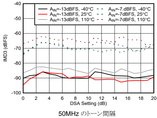
図 4-473. RX IMD3 と DSA 設定との関係 (9.6GHz)
