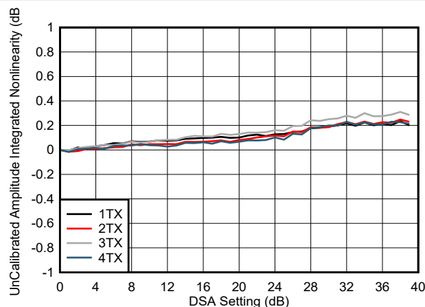
図 4-192. TX DSA 校正済み振幅の積分非直線性 (8.11GHz)
