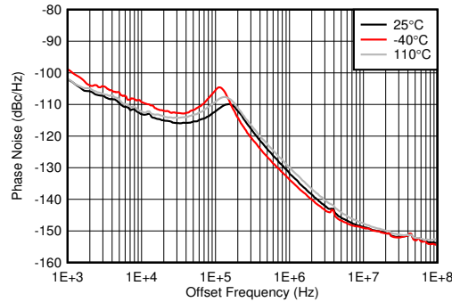
図 4-521. 8GHz VCO の位相ノイズとオフセット周波数との関係 (各種温度、 f_{OUT} = 1910\text{MHz} )
