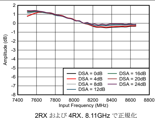
図 4-440. RX 振幅と周波数との関係 (各種 DSA 設定)
