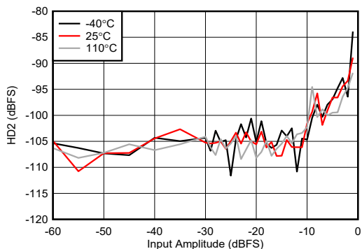
図 4-452. RX HD2 とデジタル振幅との関係 (8.11GHz)
