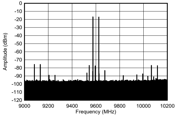
図 4-275. TX 2 トーン スペクトル (9.61GHz、-13dBFS、1.2GHz BW)
