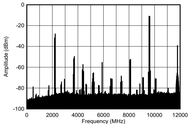
図 4-272. TX 2 トーン スペクトル (9.61GHz、-7dBFS、広帯域)
