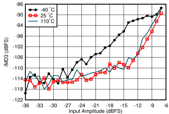
0.8GHz 整合あり、トーン間隔 = 20MHz、DSA = 4dB
