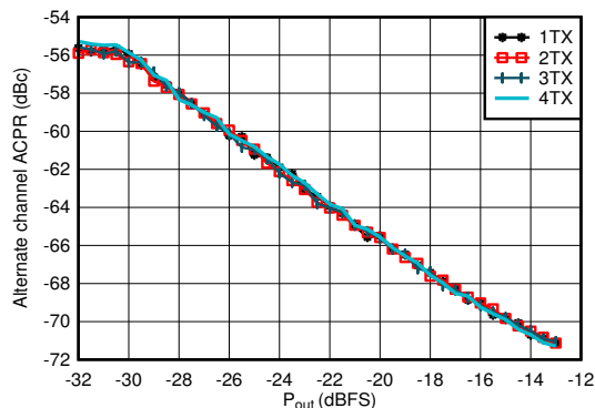
図 4-176. TX 20MHz LTE alt-ACPR とデジタルレベルとの関係 (4.9GHz)
