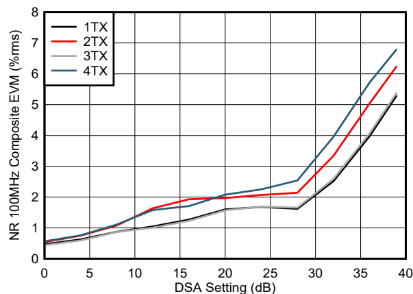
図 4-283. TX NR100MHz EVM と DSA 設定との関係 (9.61GHz)
