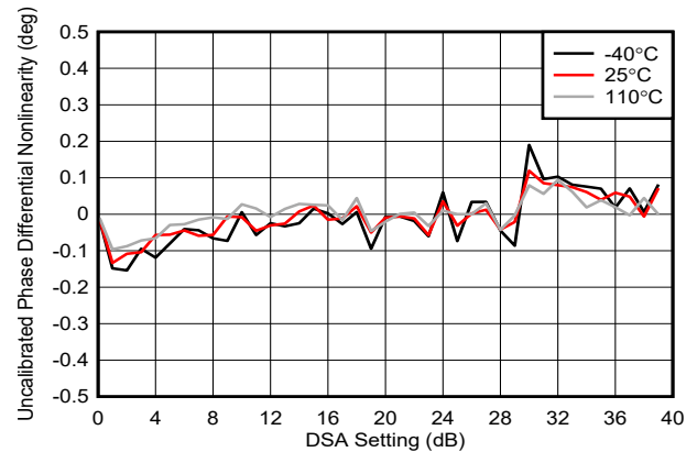
図 4-195. TX DSA 未較正位相の微分非直線性 (8.11GHz)
