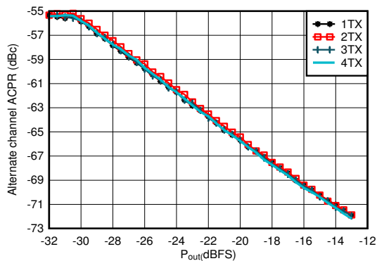
図 4-70. TX 20MHz LTE alt-ACPR とデジタル レベルとの関係 (1.8425GHz)
