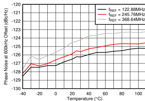
図 4-510. 10GHz VCO の位相ノイズと温度との関係 (各種 f_{REF} 、 f_{OUT} = 2.6\text{GHz} 、600kHz オフセット)
