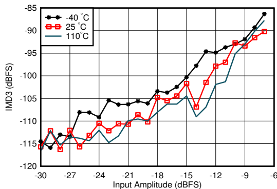
0.8GHz 整合あり、トーン間隔 = 20MHz、DSA = 12dB
