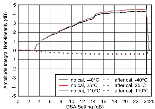
図 4-442. RX 振幅の積分非直線性 (8.1GHz)
