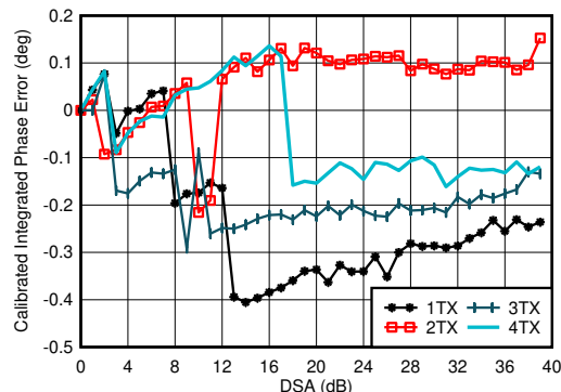
図 4-127. TX 校正済み積分位相誤差と DSA 設定との関係 (各種チャンネル、3.5GHz)
