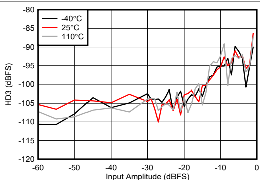
図 4-454. RX HD3 とデジタル振幅との関係 (8.11GHz)
