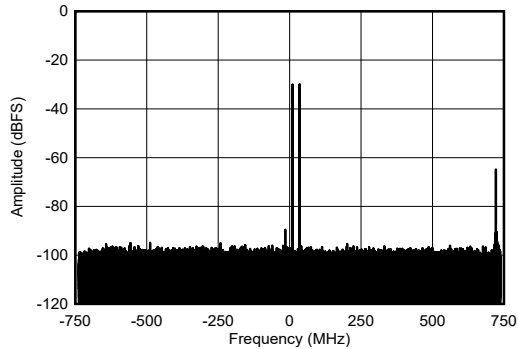
図 4-487. RX ツー トーン出力 FFT (9.61GHz)
