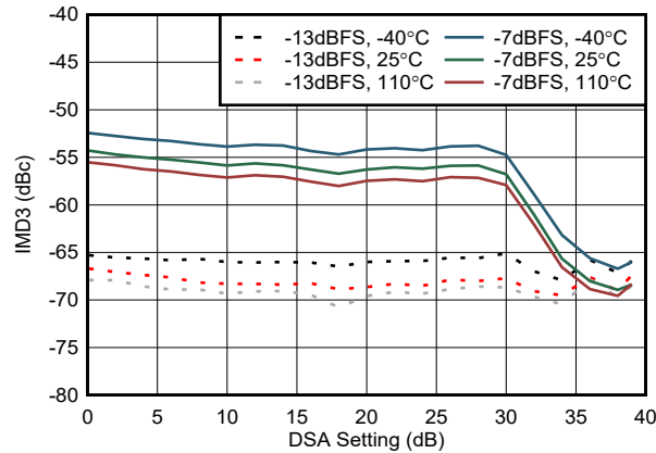
図 4-220. TX IMD3 と DSA 設定との関係 (8.1GHz)
