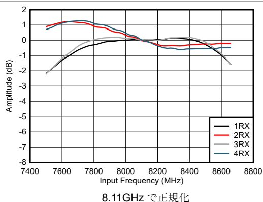
図 4-438. RX 振幅と周波数との関係 (各種チャネル)
