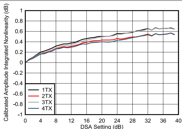
図 4-191. TX DSA 未校正振幅の積分非直線性 (8.11GHz)
