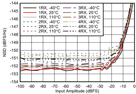
図 4-475. RX NSD とデジタル振幅との関係 (9.6GHz)
