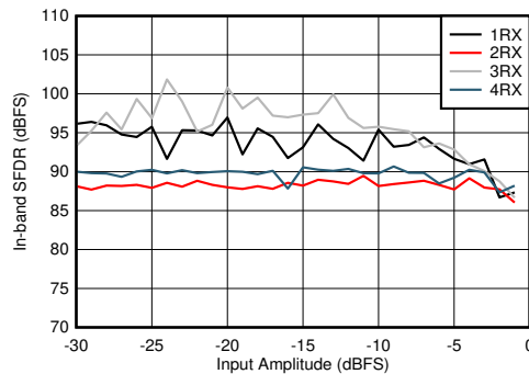
図 4-404. RX 帯域内 SFDR ( \pm 200\text{MHz} ) と入力レベルとの関係 (各種チャネル、3.6GHz)
