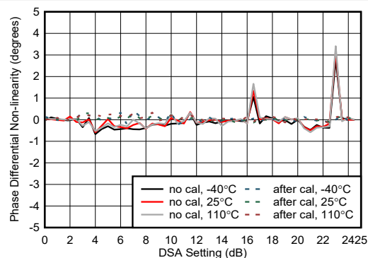
図 4-443. RX 位相の微分非直線性 (8.1GHz)
