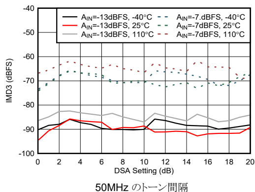
図 4-472. RX IMD3 と DSA 設定との関係 (9.6GHz)
