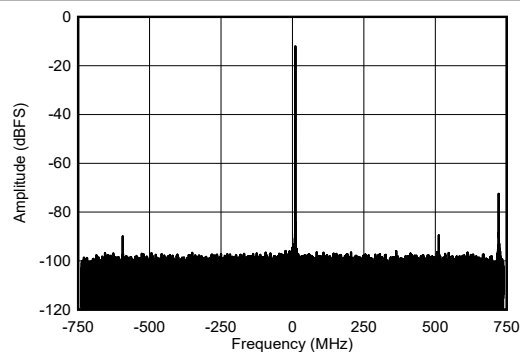
図 4-482. RX シングル トーン出力 FFT (9.6GHz)
