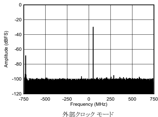
図 4-459. RX シングル トーン出力 FFT (8.11GHz、-30dBFS)
