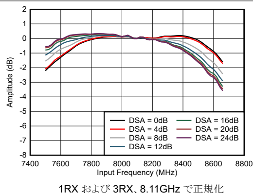
図 4-439. RX 振幅と周波数との関係 (各種 DSA 設定)
