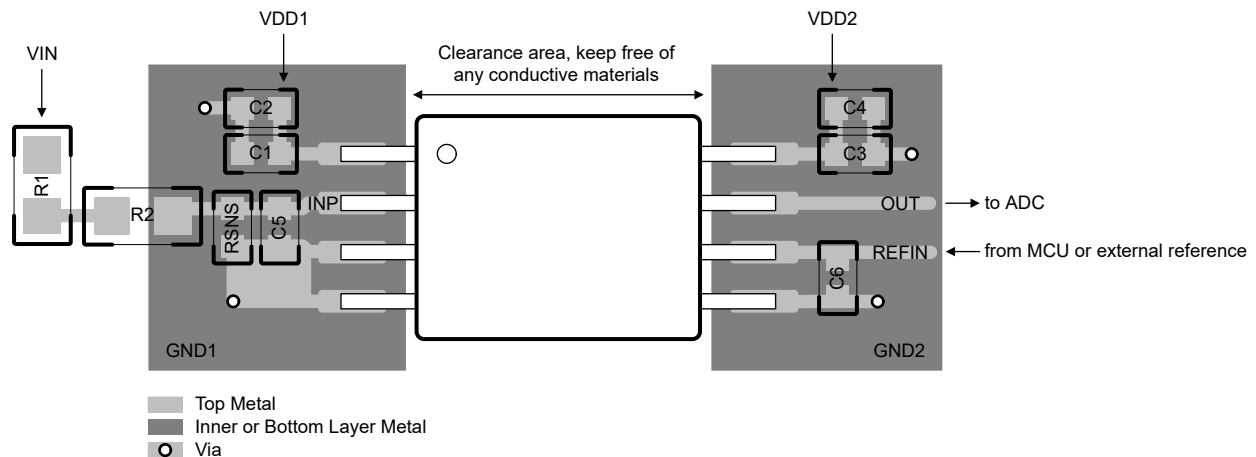
図 8-6. AMC0x11R の推奨レイアウト
