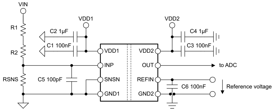
図 8-5. AMC0x11R のデカップリング
