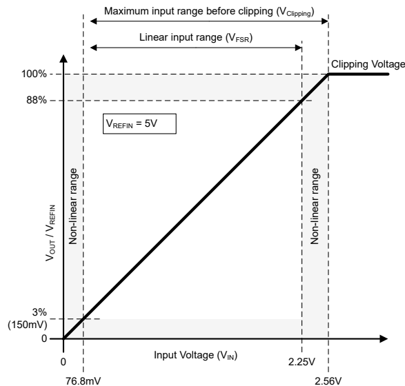
図 7-2. AMC0x11R の入力から出力への伝達曲線
