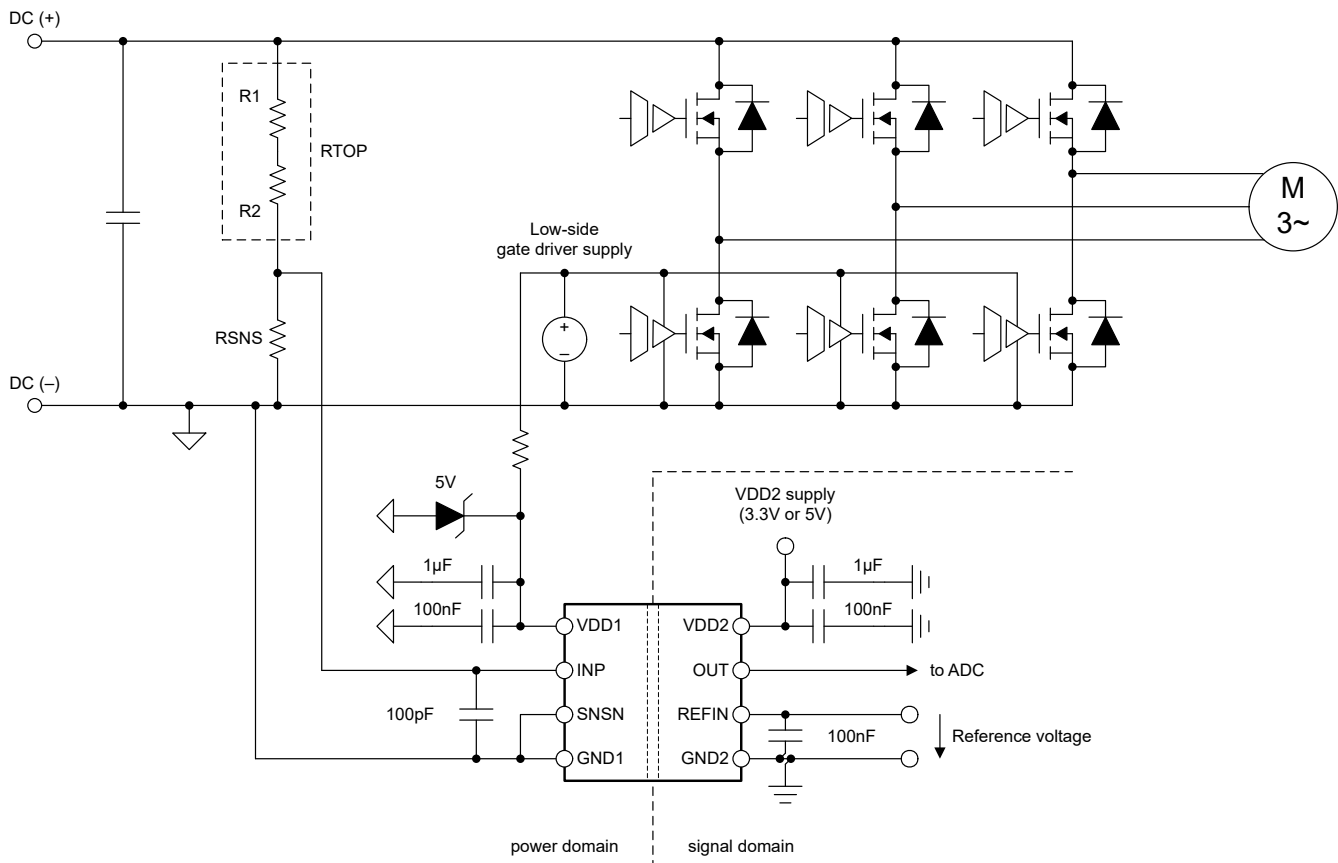
図 8-1. 代表的なアプリケーションで使用 AMC0x11R
