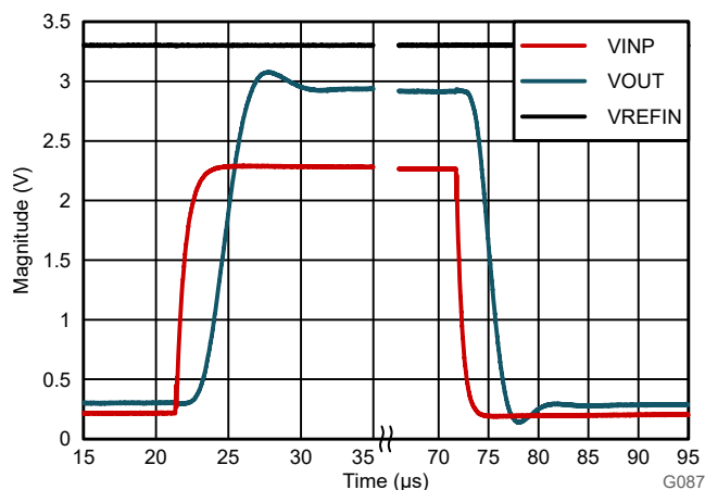
図 8-4. AMC0x11R のステップ応答
