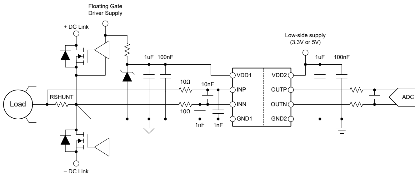
図 8-1. 代表的なアプリケーションでの電流検出に AMC0x02D-Q1 を使用
