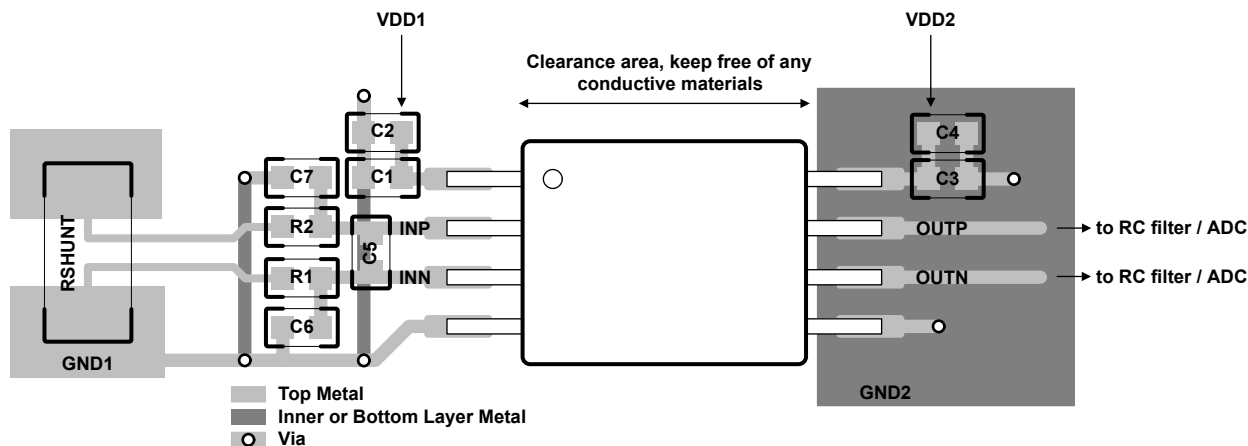
図 8-6. AMC0x02D-Q1
