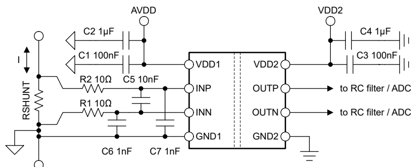
図 8-5. AMC0x02D-Q1 のデカップリング
