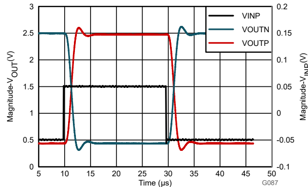
図 8-4. AMC0x02D-Q1 のステップ応答
