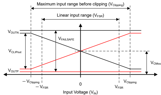
図 7-2. AMC0x02D-Q1 の入力から出力への伝達曲線
