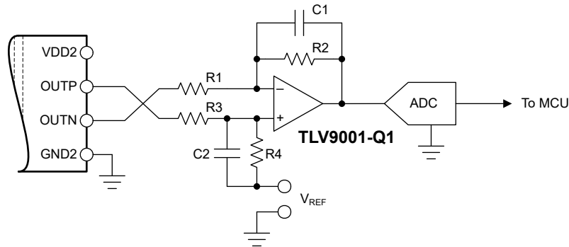
図 8-3. AMC0x02D-Q1 出力をシングルエンド入力 ADC に接続する
