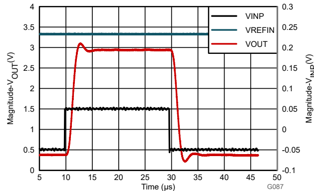
図 8-4. AMC0x02R-Q1 の出力ステップ応答
