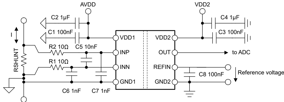
図 8-6. AMC0x02R-Q1 のデカップリング
