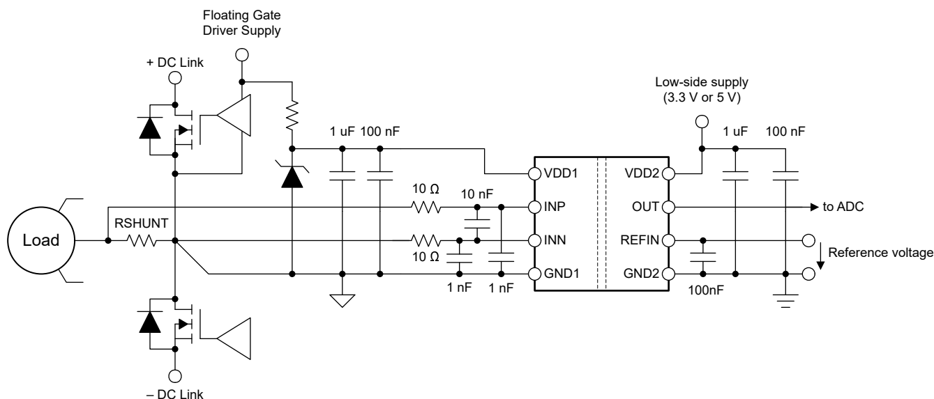
図 8-1. 代表的なアプリケーションでの電流検出に AMC0x02R-Q1 を使用
