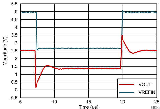
図 8-5. AMC0x02R-Q1 のリファレンス入力ステップ応答
