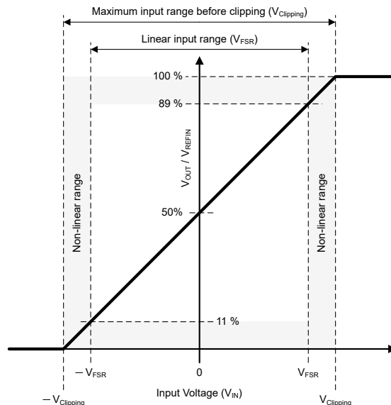
図 7-3. AMC0x02R-Q1 の入力から出力への伝達曲線
