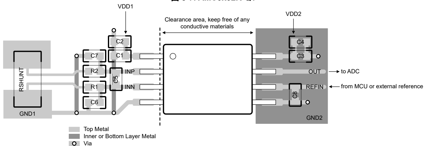
図 8-7. AMC0x02R-Q1
