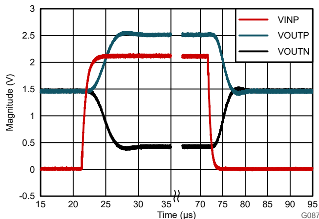
図 8-4. AMC0x11D-Q1 のステップ応答
