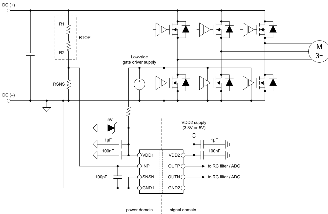
図 8-1. 代表的なアプリケーションで使用する AMC0x11D-Q1
