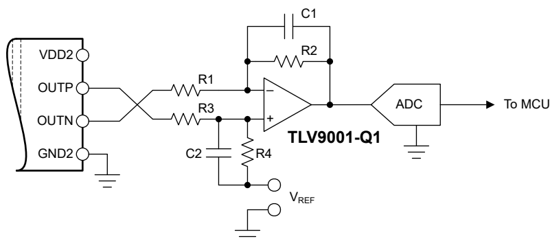
図 8-3. AMC0x11D-Q1 出力をシングルエンド入力 ADC に接続する
