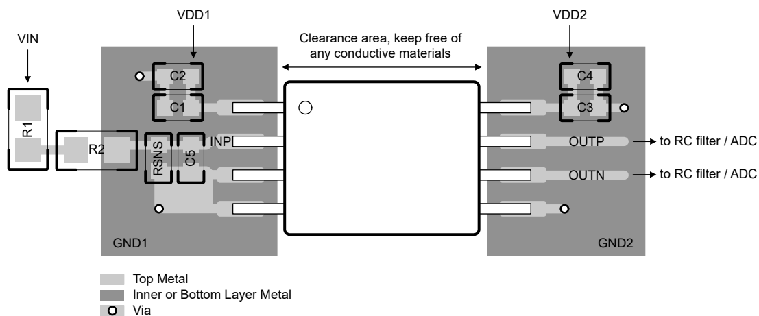
図 8-6. AMC0x11D-Q1 の推奨レイアウト
