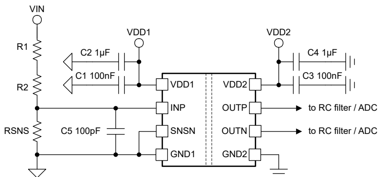
図 8-5. AMC0x11D-Q1 のデカップリング
