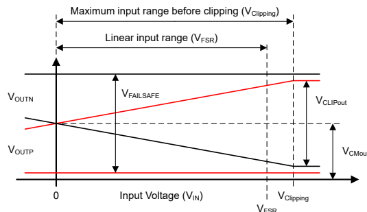
図 7-2. AMC0x11D-Q1 の入力から出力への伝達曲線
