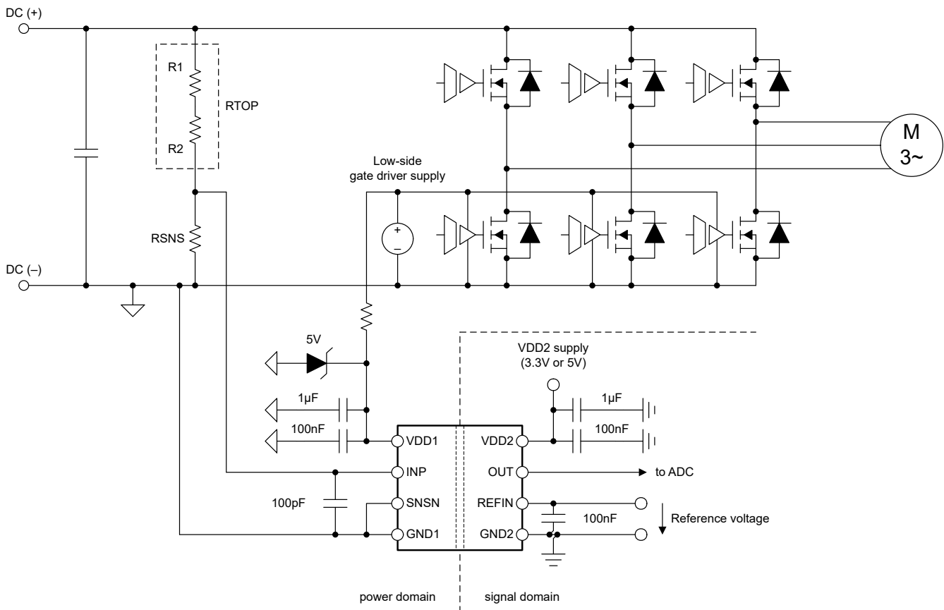
図 8-1. 代表的なアプリケーションで使用する AMC0x11R-Q1
