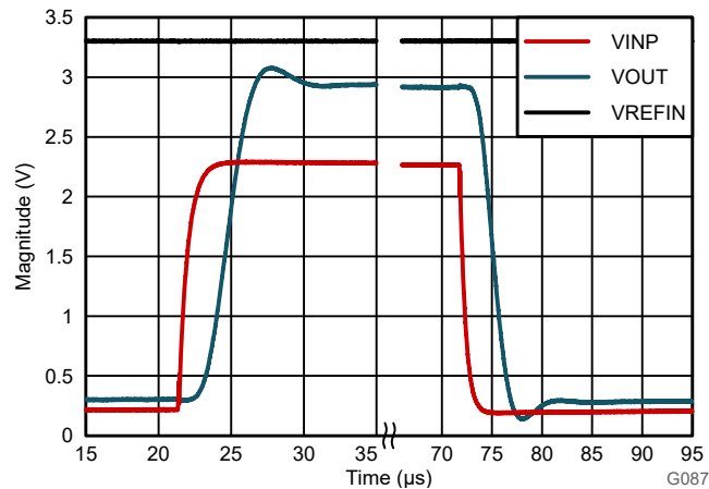
図 8-4. AMC0x11R-Q1 のステップ応答
