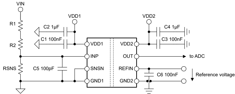
図 8-5. AMC0x11R-Q1 のデカップリング
