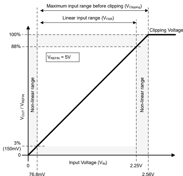
図 7-2. AMC0x11R-Q1 の入力から出力への伝達曲線
