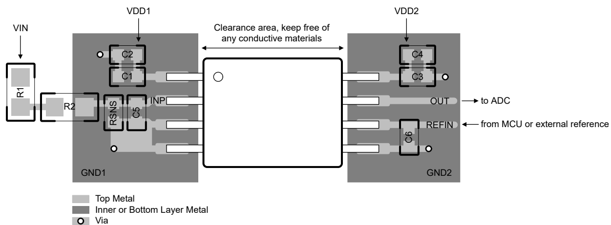
図 8-6. AMC0x11R-Q1 の推奨レイアウト
