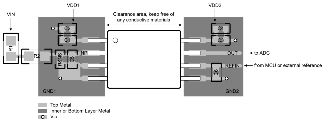
図 8-6. AMC0x11S-Q1 の推奨レイアウト
