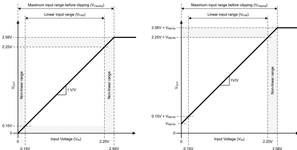
図 7-2. AMC0x11S-Q1
