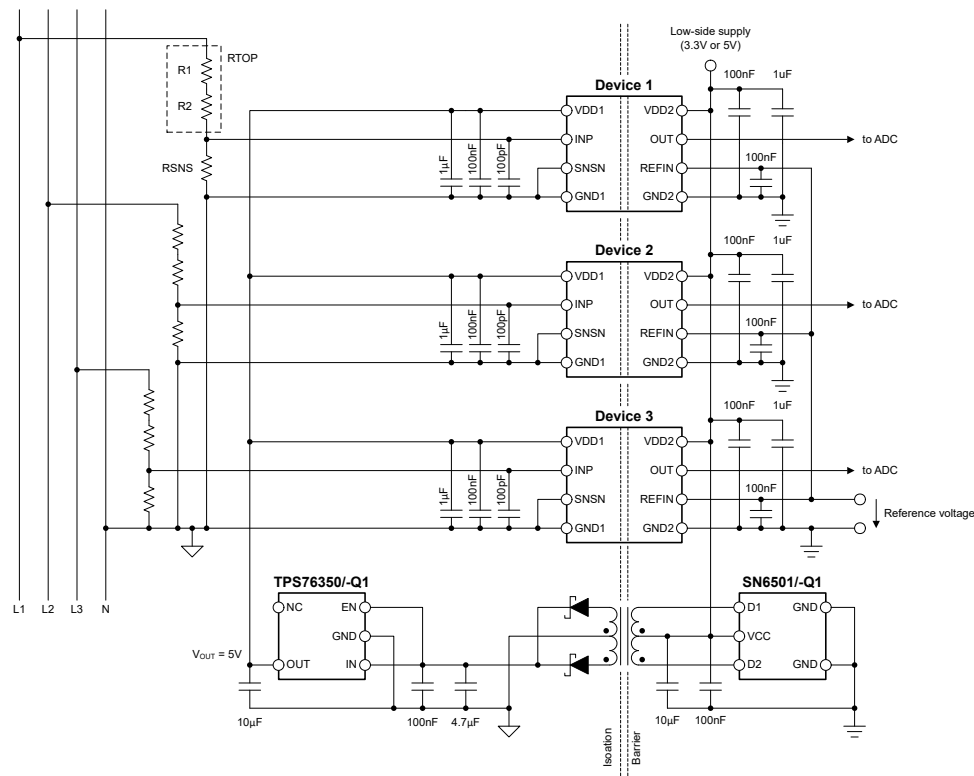
図 8-1. 代表的なアプリケーションで使用する AMC0380R-Q1
