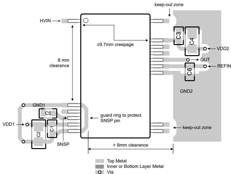
図 8-6. AMC0381R の推奨レイアウト
