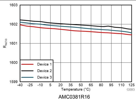
図 6-10. 分圧比と温度との関係
