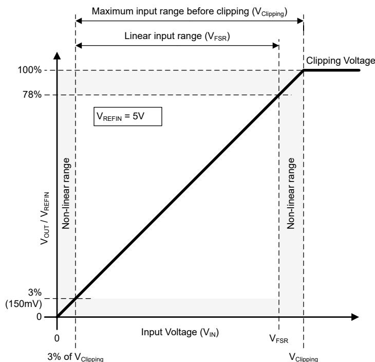
図 7-2. AMC0381R の入力から出力への伝達曲線
