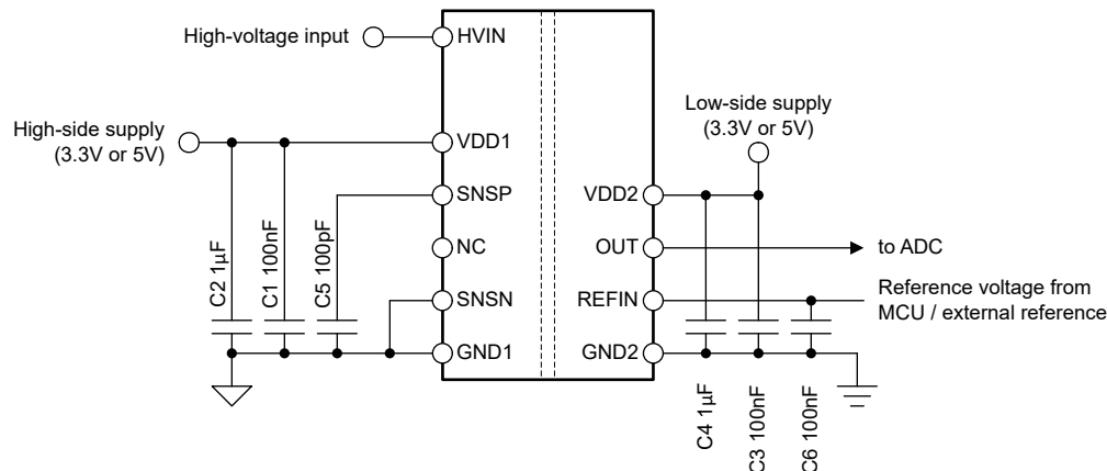
図 8-5. AMC0381R のデカップリング
