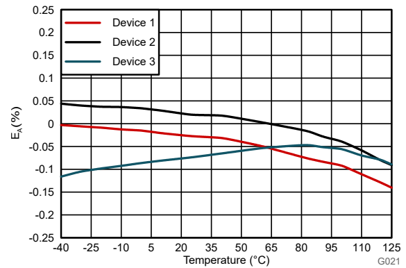
図 6-18. 減衰誤差と温度との関係
