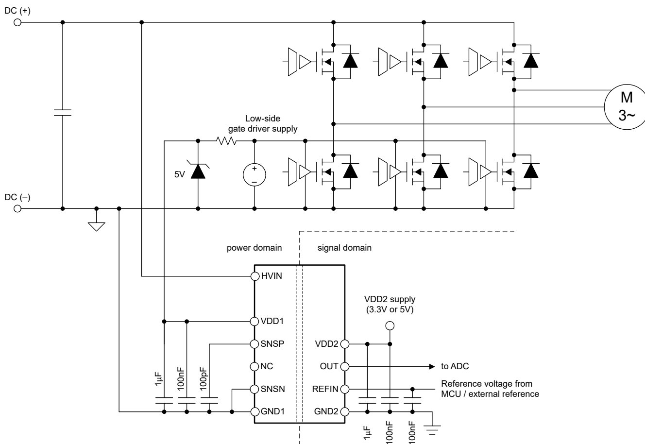
図 8-1. 代表的なアプリケーションで使用 AMC0381R
