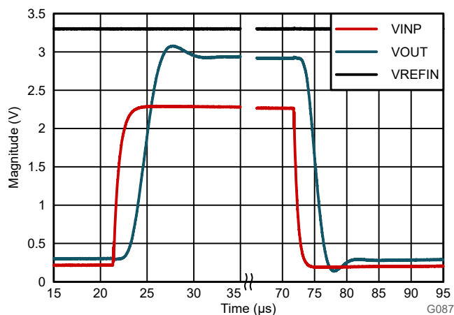
図 8-4. AMC0381R のステップ応答
