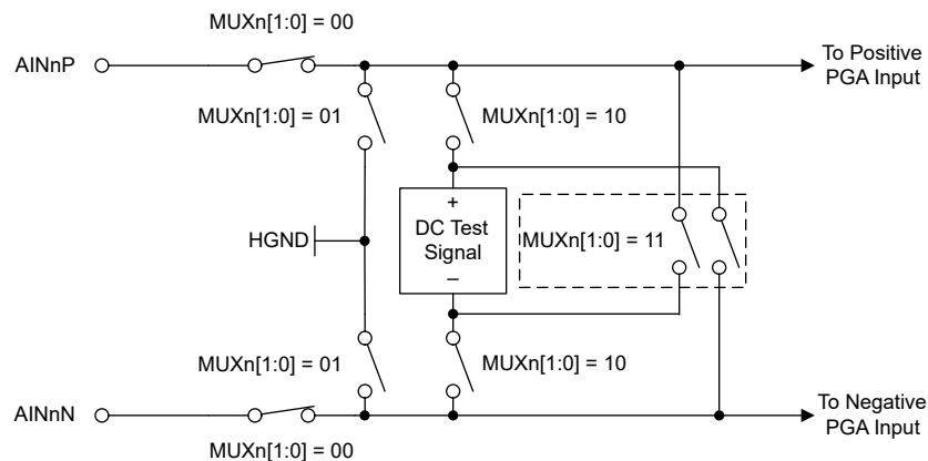
图 8-4. Input Multiplexer
