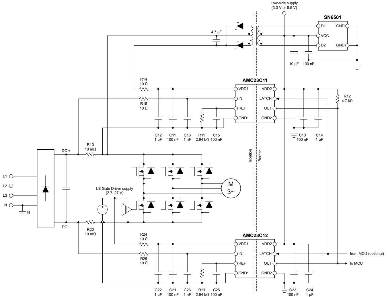
図 7-1. AMC23C11 による DC+ 過電流検出
