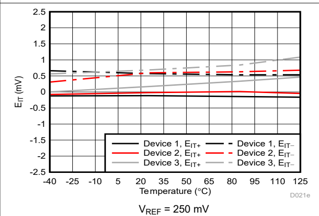
図 5-15. のトリップスレッシュホールド誤差と温度との関係
