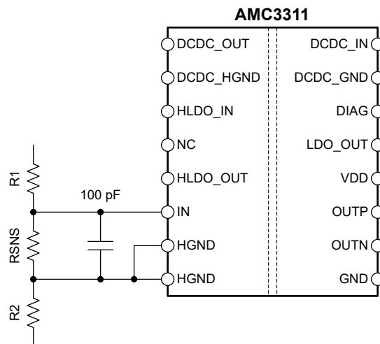
図 8-2. Input Filter
