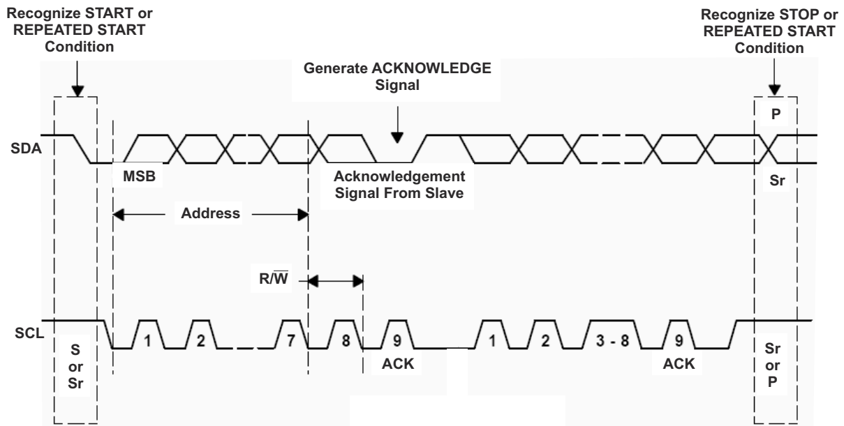
图 7-12. Bus Protocol
