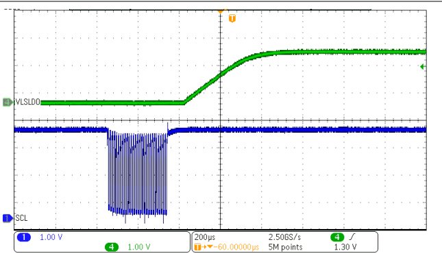
VBAT = 3.6V
