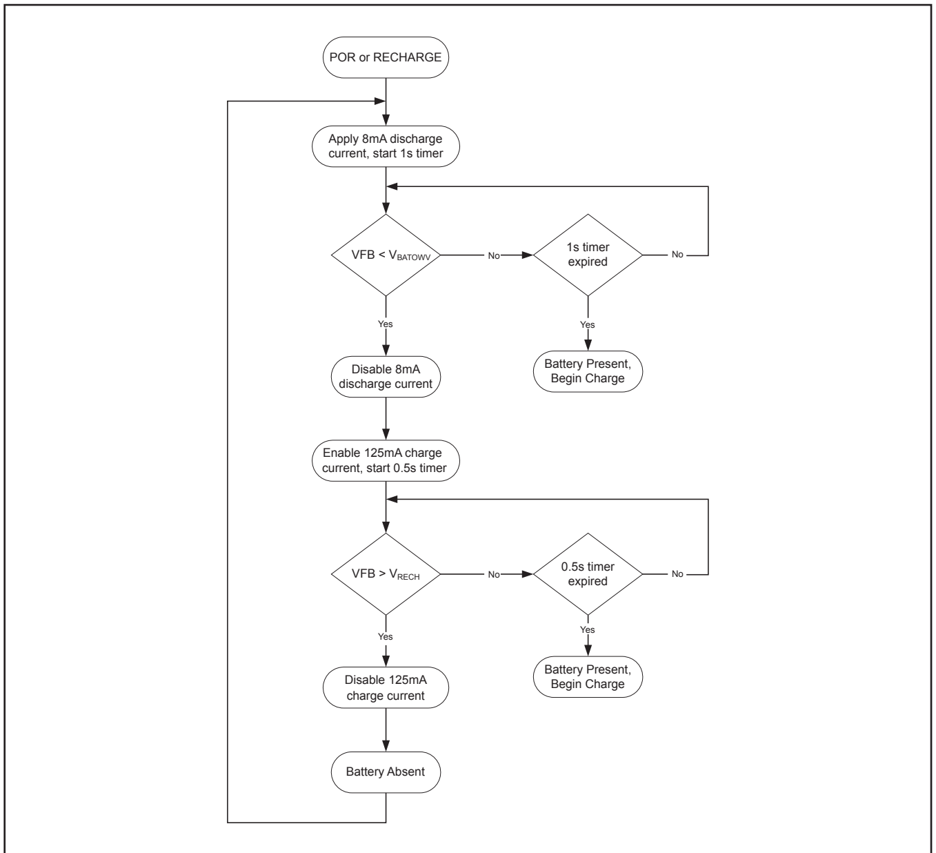
図 20. バッテリー検出フローチャート
