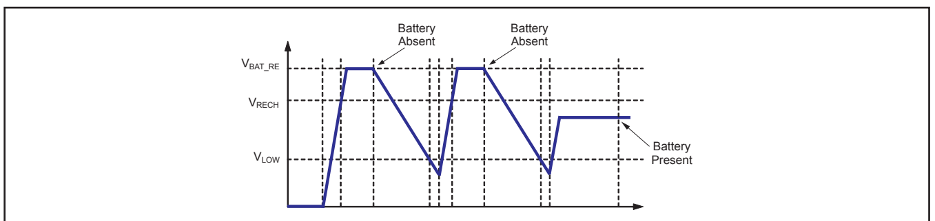
図 21. バッテリー検出タイミング図
