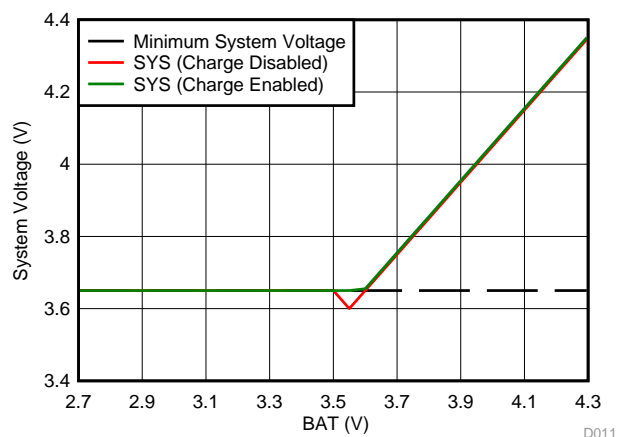
10. V(SYS) vs V(BAT)
