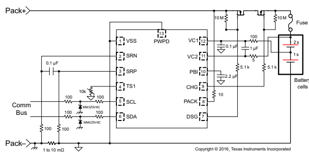
概略回路図
