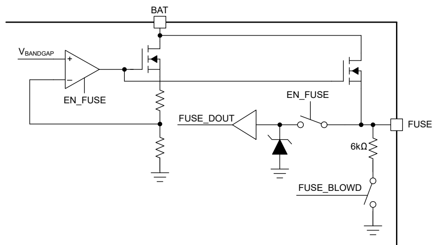
図 5-4. Fuse Pin
