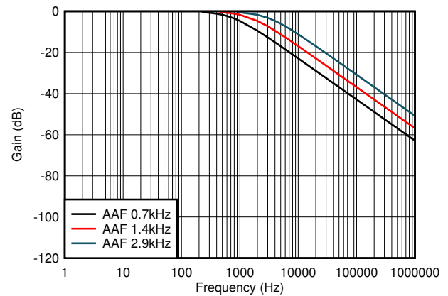
7-6. AUX ADC Filter
