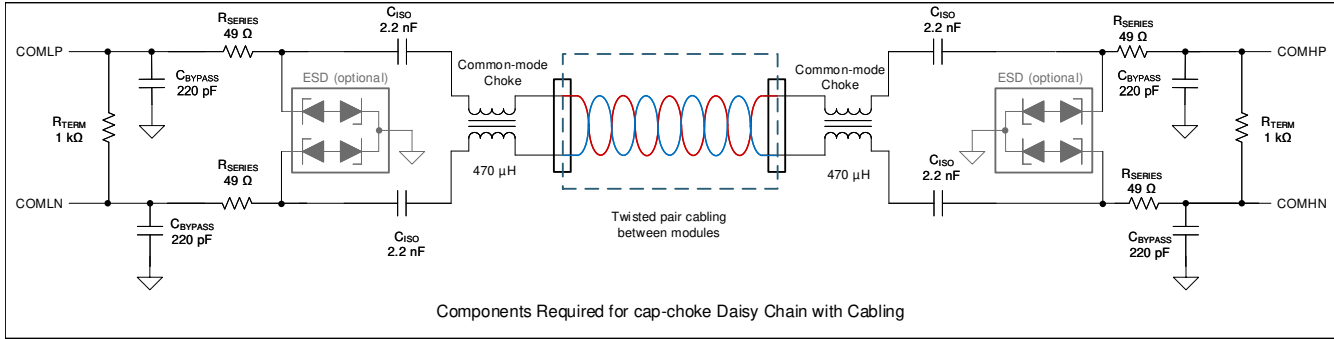
图 9-8. Capacitor Plus Choke Isolation
