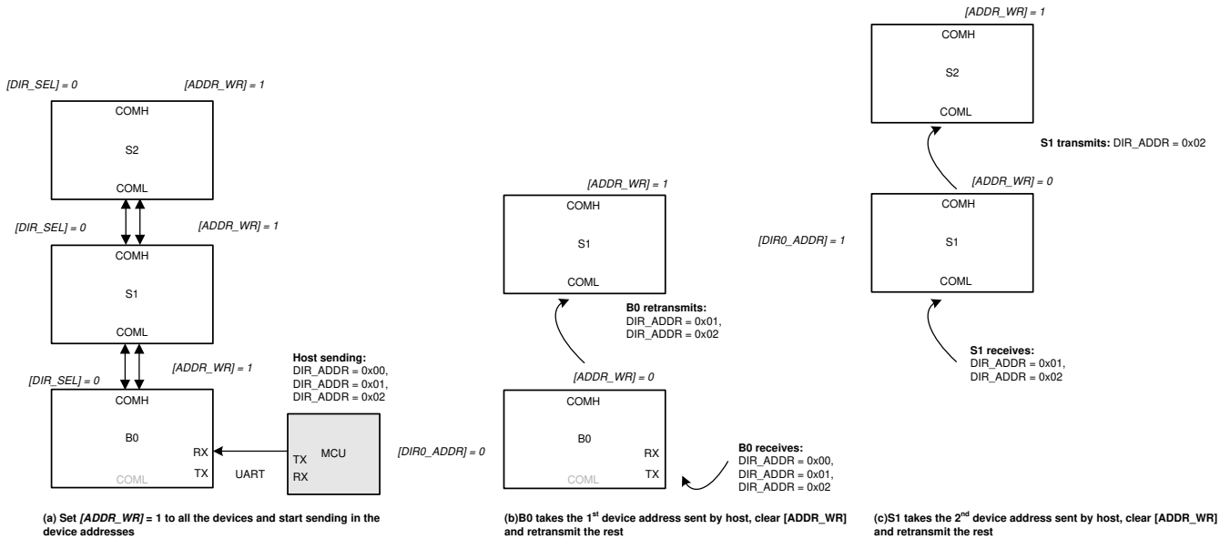
图 8-36. Auto-Addressing
