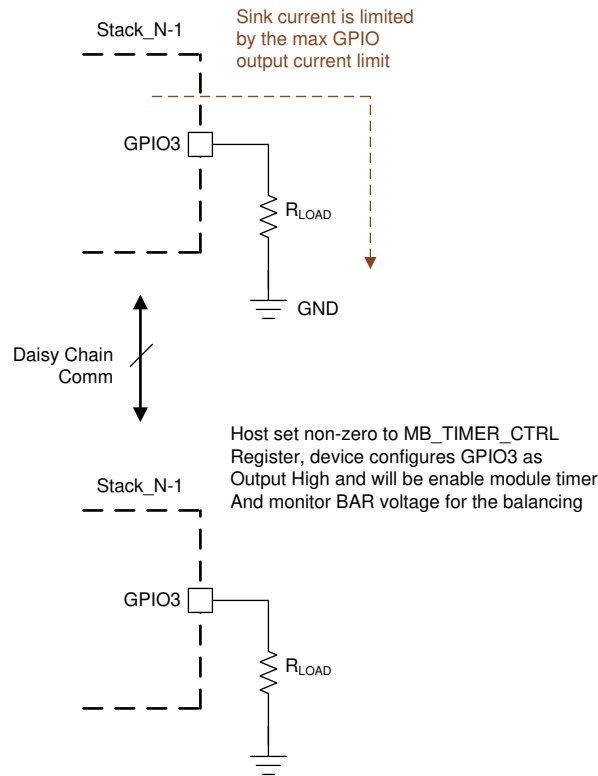
图 8-18. Module Balancing
