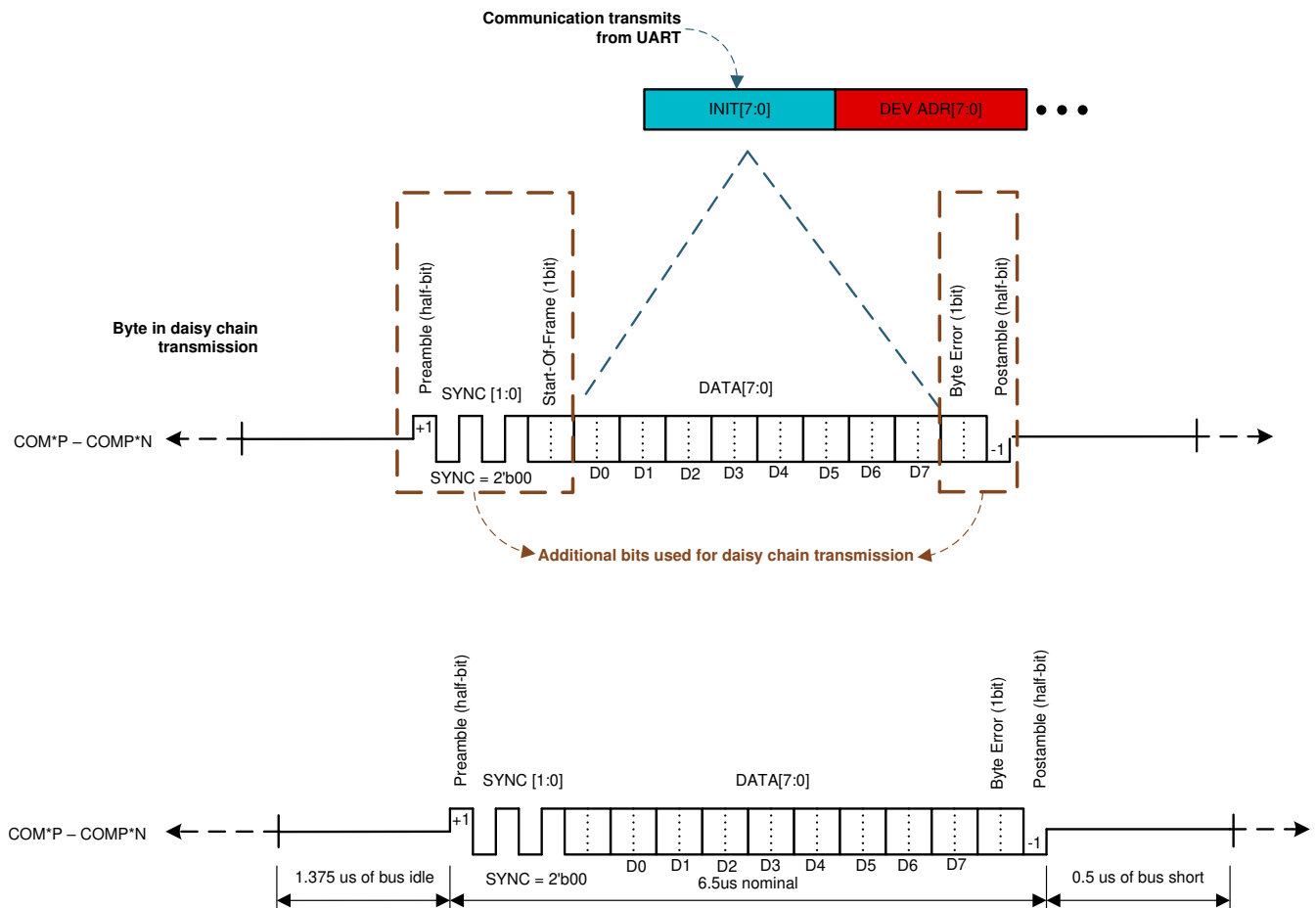
图 8-33. Daisy Chain Byte Definition
