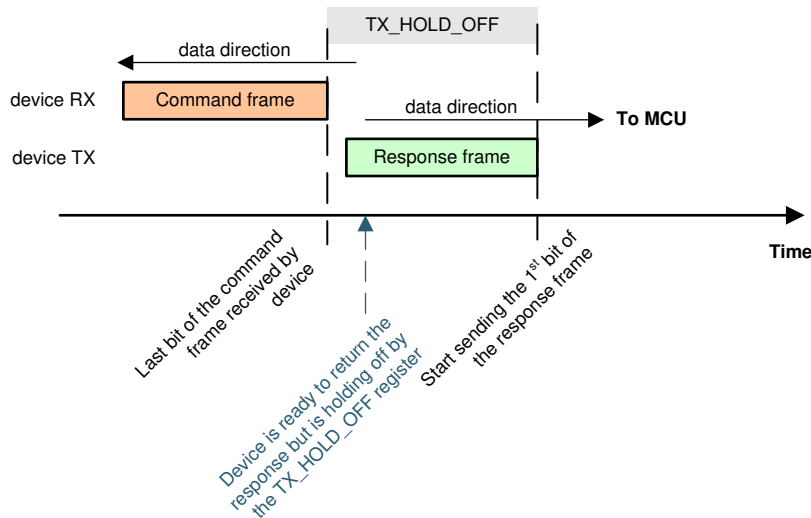
8-25. UART TX_HOLD_OFF
