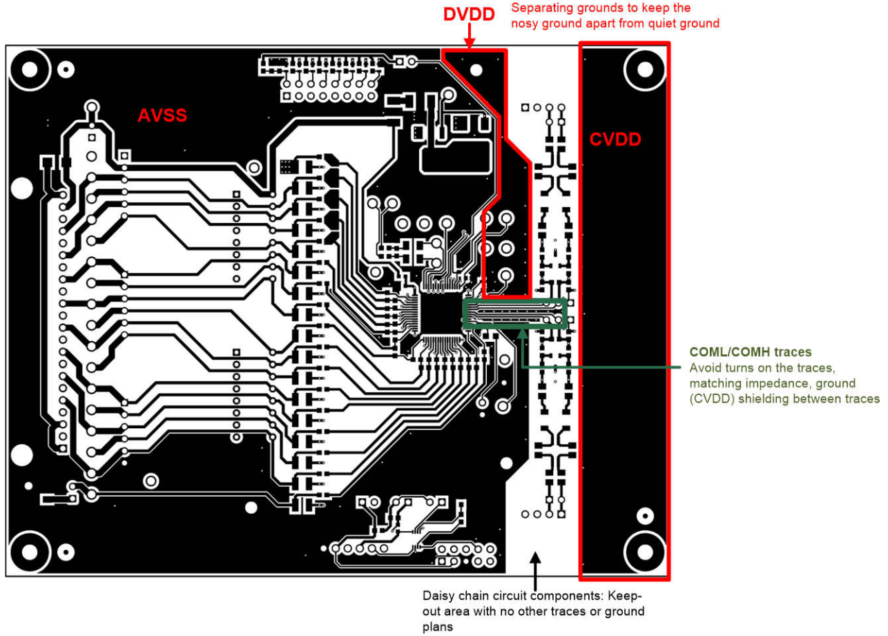
11-4. Top Signal Layer
