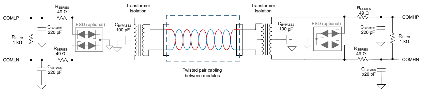
图 9-9. Transformer Isolation
