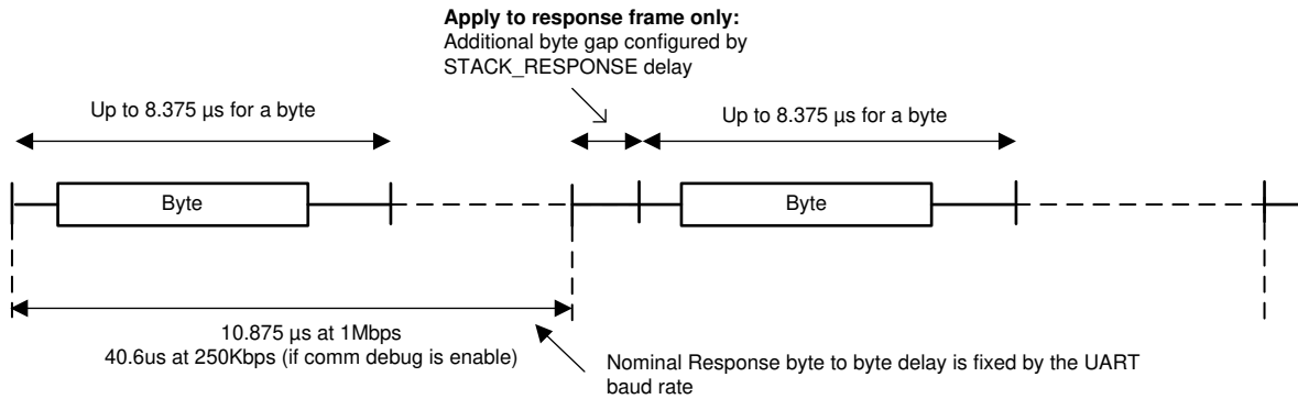
图 8-34. Daisy Chain Byte Transfer
