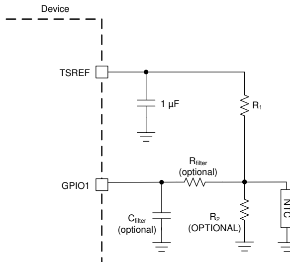
图 8-6. Thermistor Connection
