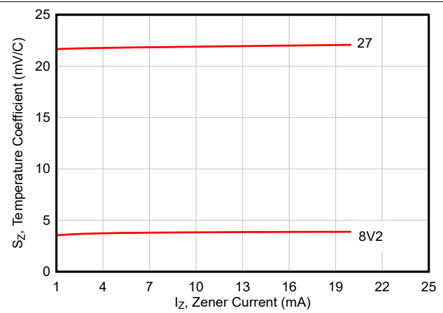
図 5-2. 温度係数
