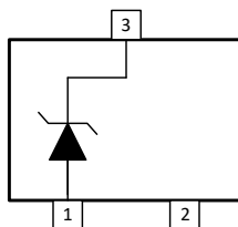
図 4-1. DCK パッケージ、3 ピン SC-70 (上面図)
