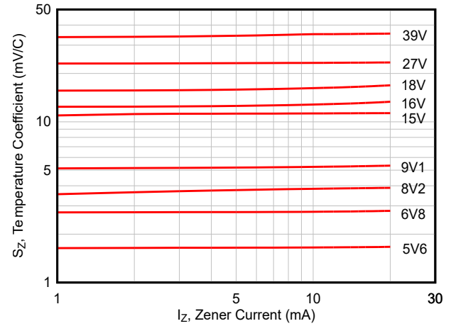
図 5-2. 温度係数
