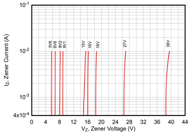
図 6-1. ツェナー電流とツェナー電圧との関係
