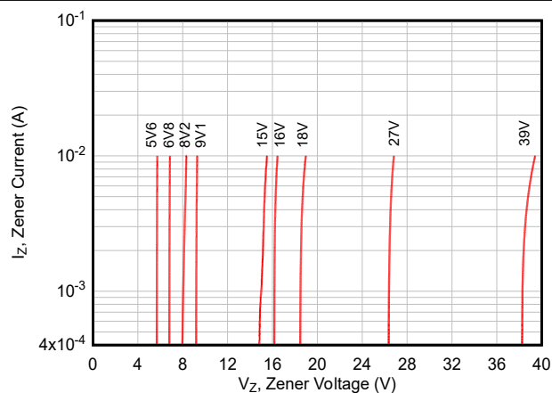
図 5-1. ツェナー電流とツェナー電圧との関係
