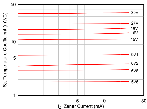
図 5-2. 温度係数
